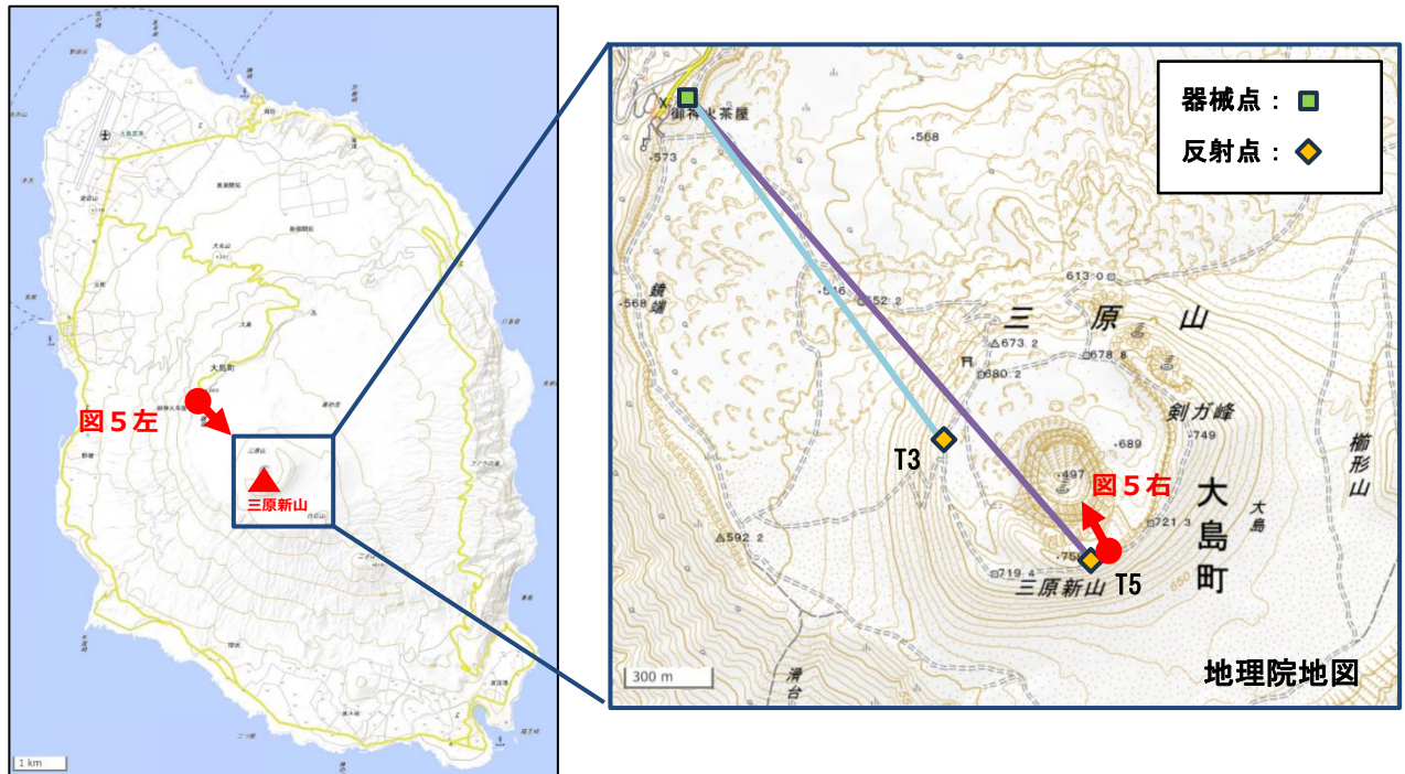
図8 伊豆大島 監視カメラの位置・撮影方向及び光波測距繰り返し観測の観測点 (赤丸：撮影位置、→：撮影方向)
