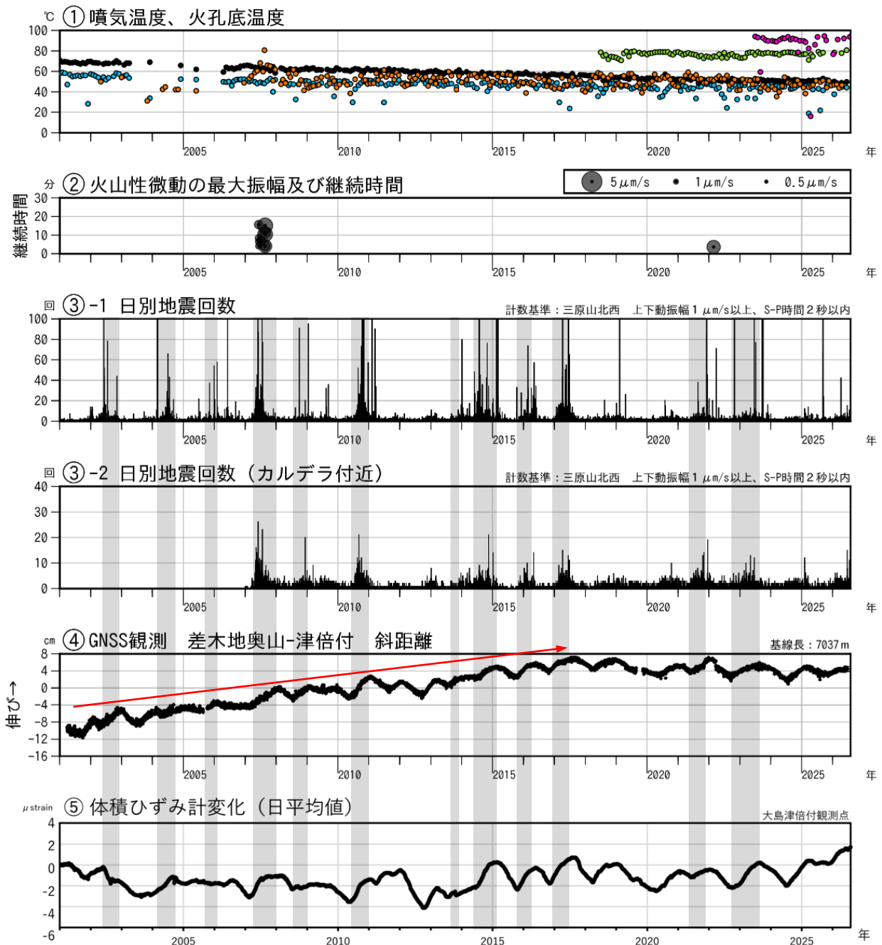
図2 伊豆大島 最近の火山活動経過図（2001年1月～2026年7月）
