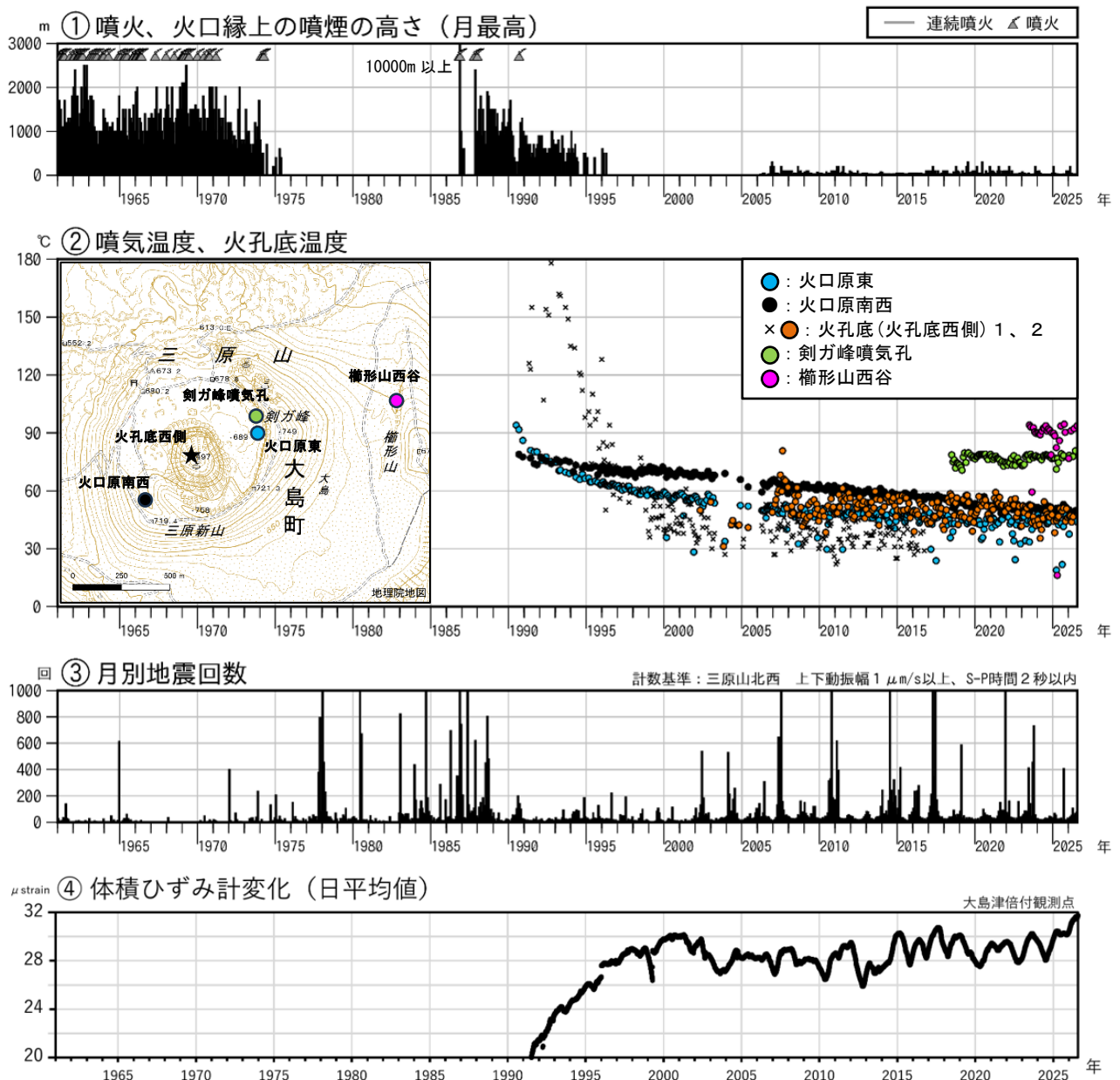
図1 伊豆大島 長期間の火山活動経過図（1961年1月～2026年7月）
