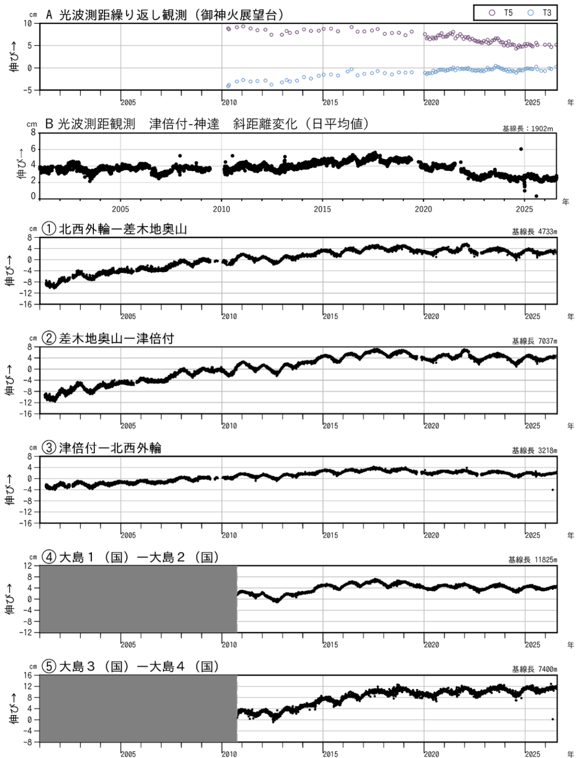
図3-1 伊豆大島 GNSS連続観測及び光波測距観測による基線長変化(2001年1月～2026年7月)
