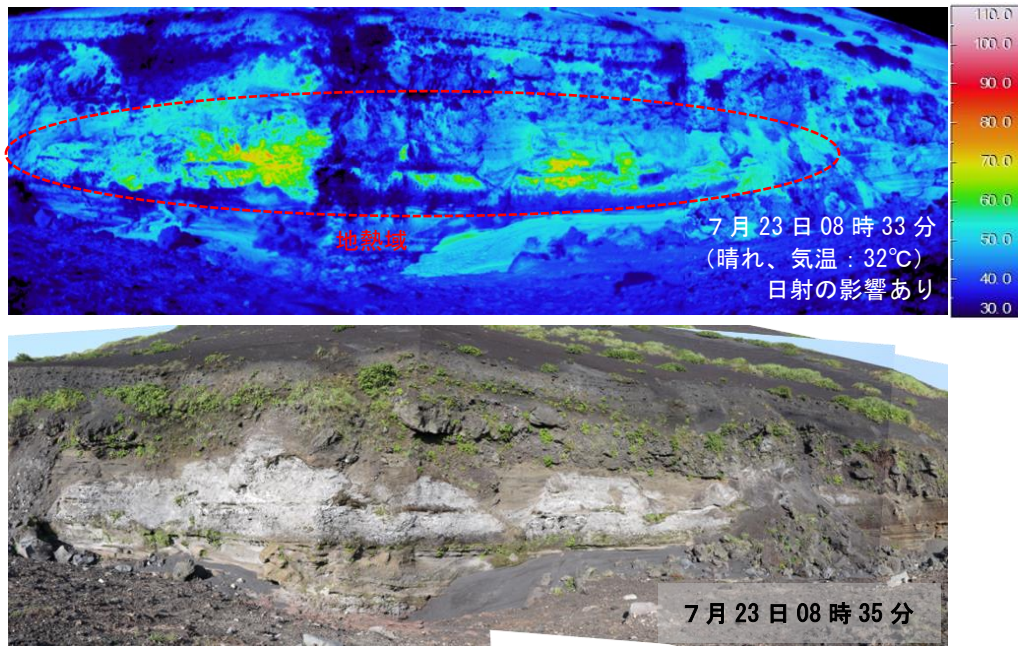
図6-2 伊豆大島 櫛形山西谷の状況（撮影方向は図6-3参照）
