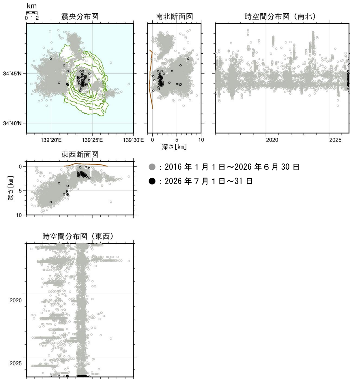
図4 伊豆大島 震源分布図（2016 年 1 月 1 日～2026 年 7 月 31 日）
