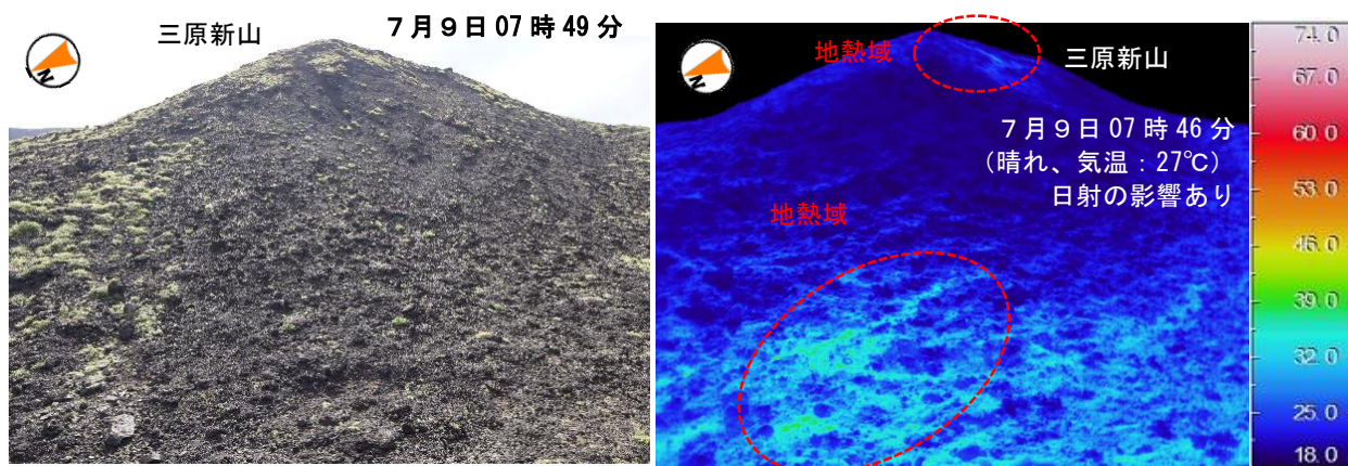
図6-1 伊豆大島 三原新山及び火口原南西の状況（撮影方向は図6-3参照）
