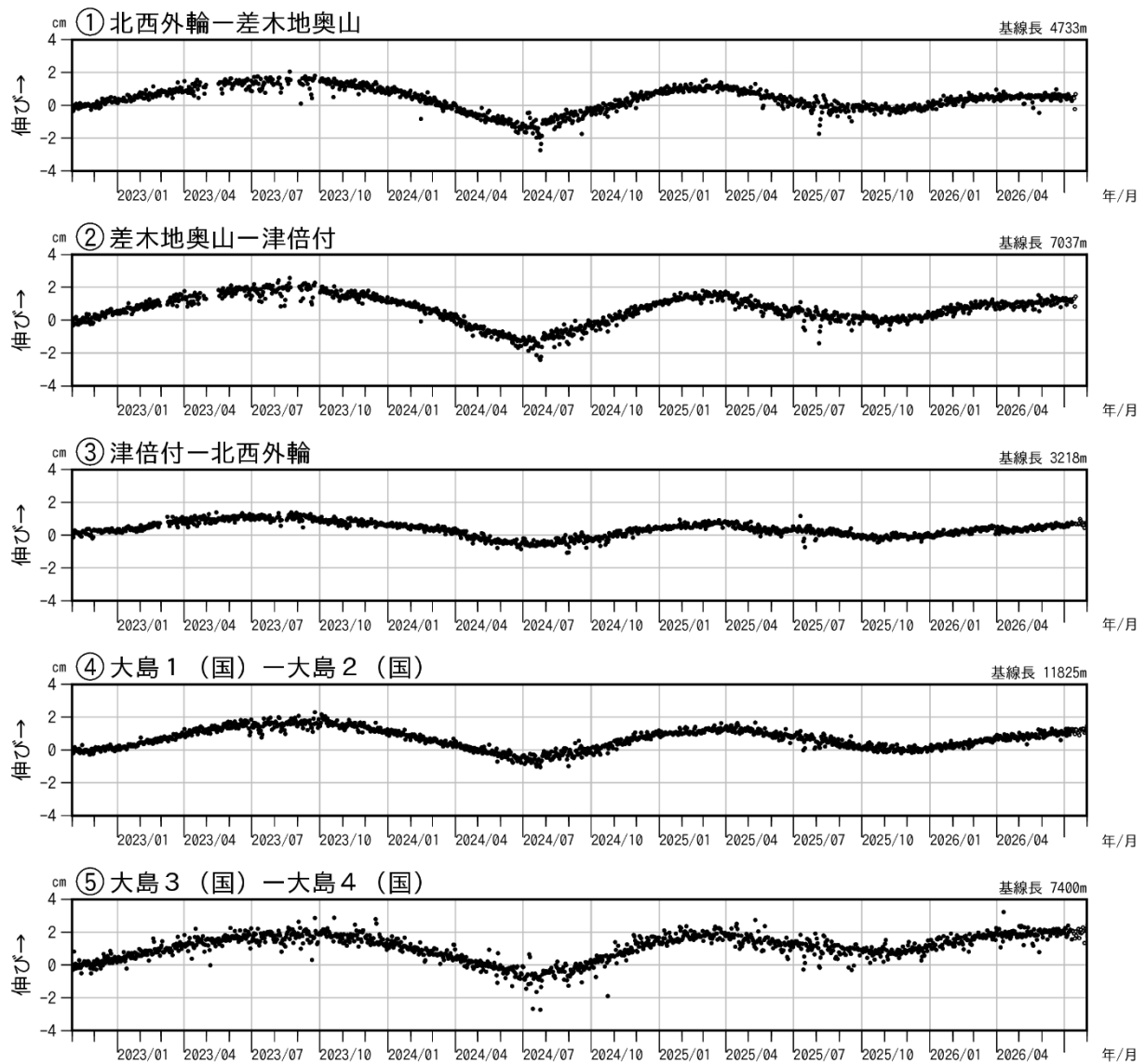
図3-2 伊豆大島 GNSS 連続観測による基線長変化(2022年11月～2026年7月)
