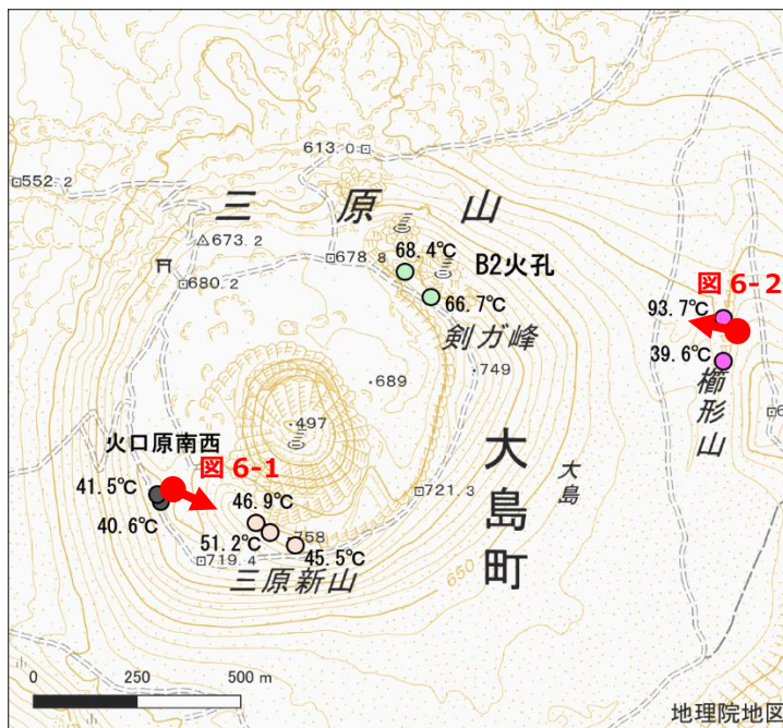
図6-3 伊豆大島 噴気温度の分布及び現地調査での撮影位置・撮影方向
