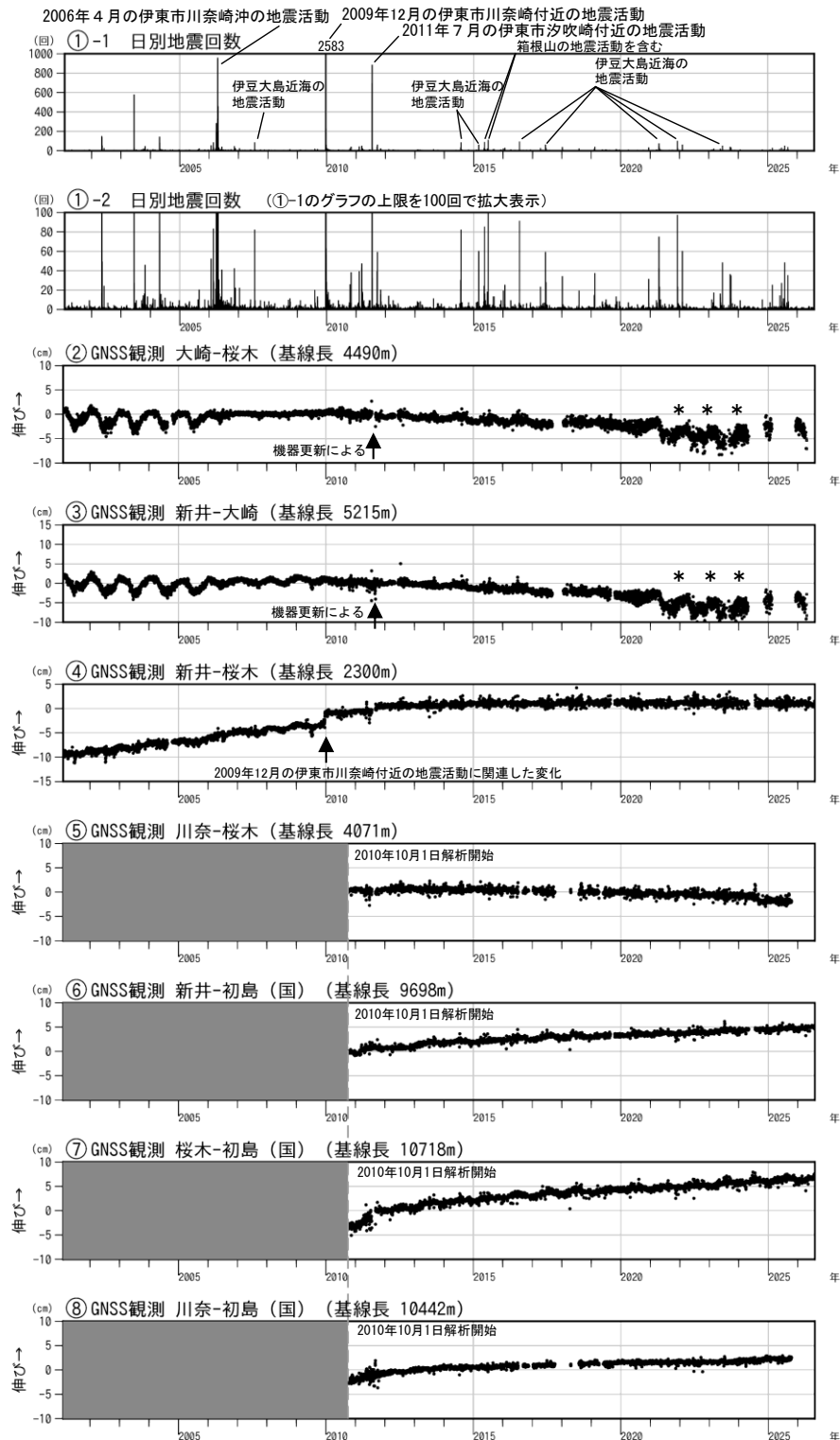
図3 伊豆東部火山群 火山活動経過図（2001年2月1日～2026年7月31日）
