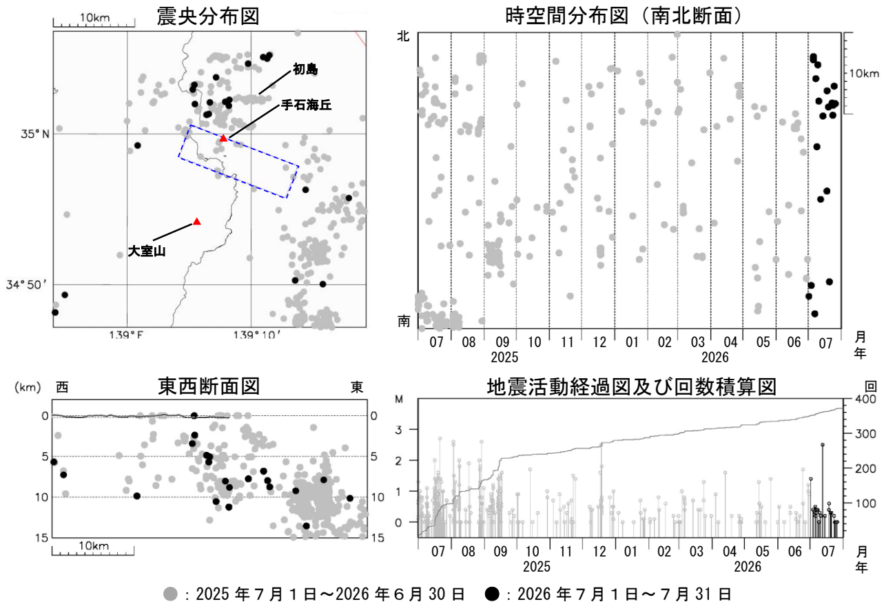
図2 伊豆東部火山群 広域地震観測網による震源分布図（2025年7月1日～2026年7月31日） □の領域は群発地震活動の発生する可能性がある範囲（火口が出現する可能性のある範囲）を示しています。 https://www.data.jma.go.jp/vois/data/filing/level/PDF/level_316.pdf 広域地震観測網により震源決定したもので、深さは全て海面以下として決定しています。 M（マグニチュード）は地震の規模を表し、M0.0以上を表示しています。 図中の震源要素は一部暫定値が含まれており、後日変更することがあります。 この図では、関係機関の地震波形を一元的に処理し、地震観測点の標高を考慮する等した手法で得られた震源を用いています。
