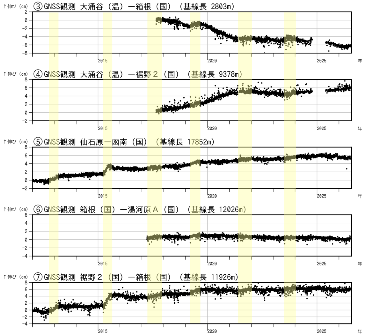
図3-2 箱根山 GNSS連続観測による 基線長変化及び観測点配置図 (2012年1月1日～2026年7月31日)
