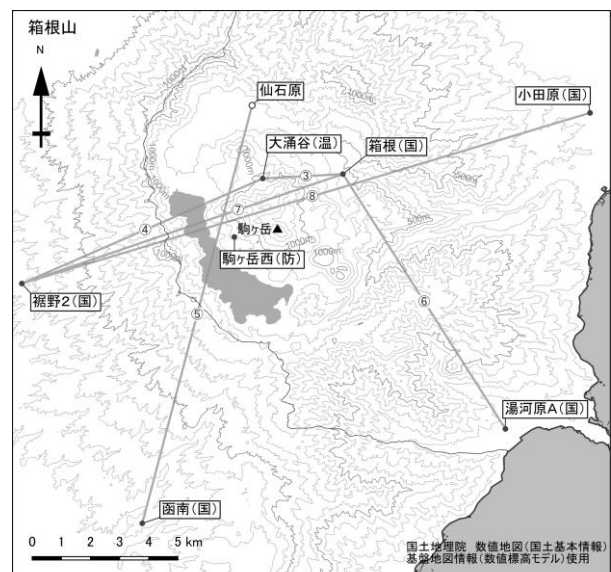
図3-2 箱根山 GNSS連続観測による 基線長変化及び観測点配置図 (2012年1月1日～2026年7月31日)
