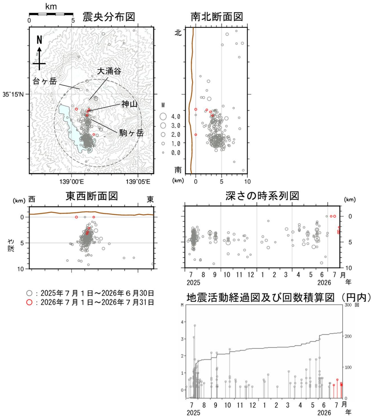
図4 箱根山 広域地震観測網による山体周辺の震源分布図（2025年7月1日～2026年7月31日）
