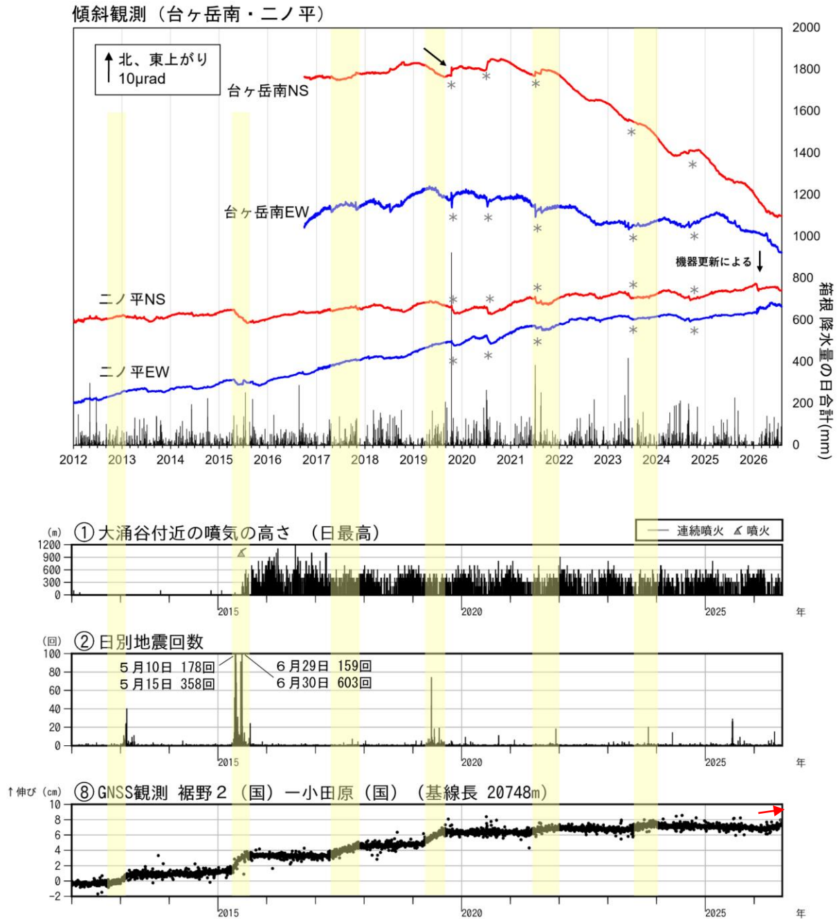
図3-1 箱根山 火山活動経過図（2012年1月1日～2026年7月31日）
