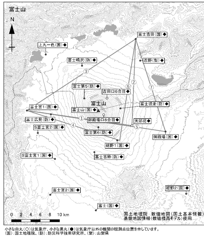
図5 富士山 GNSS 観測点配置図 GNSS 基線①～⑦は図4の①～⑦に対応しています。
