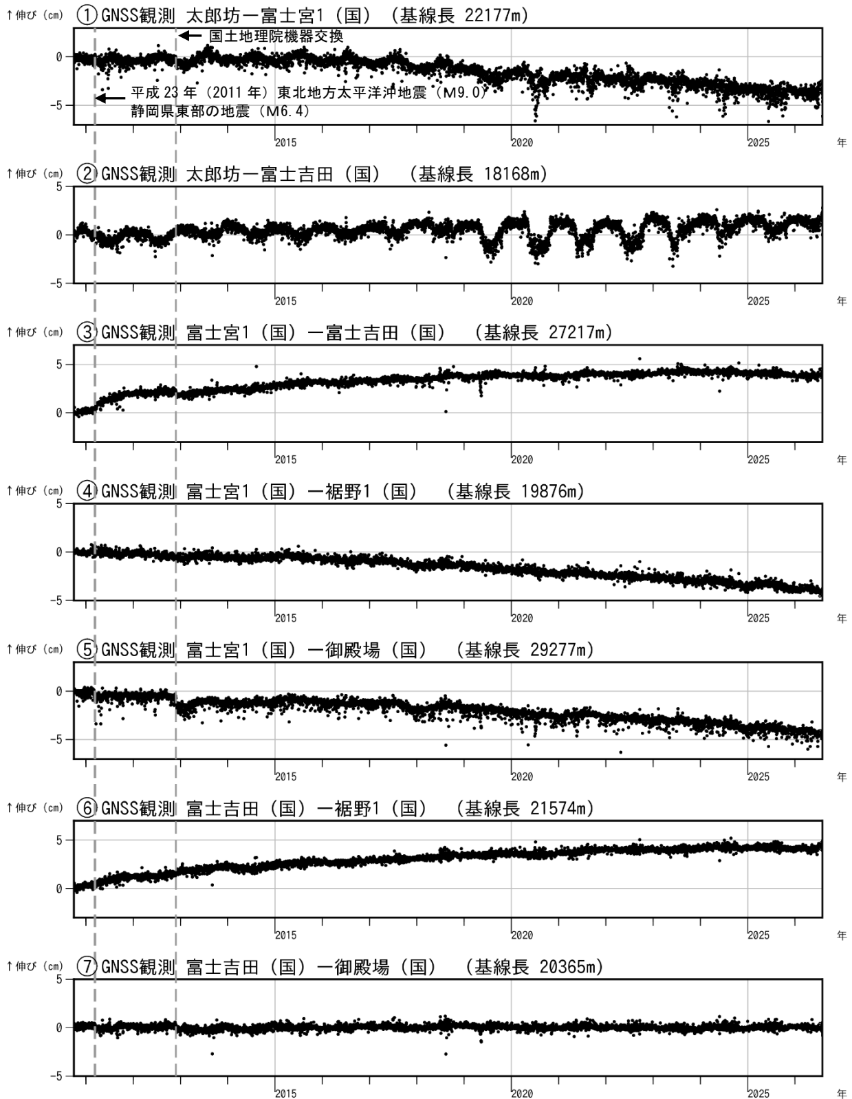
図4 富士山 GNSS 連続観測による基線長変化 (2010年10月1日～2026年7月31日)
