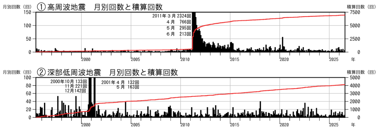
図2 富士山 月別地震回数（1995年6月1日～2026年7月31日）
