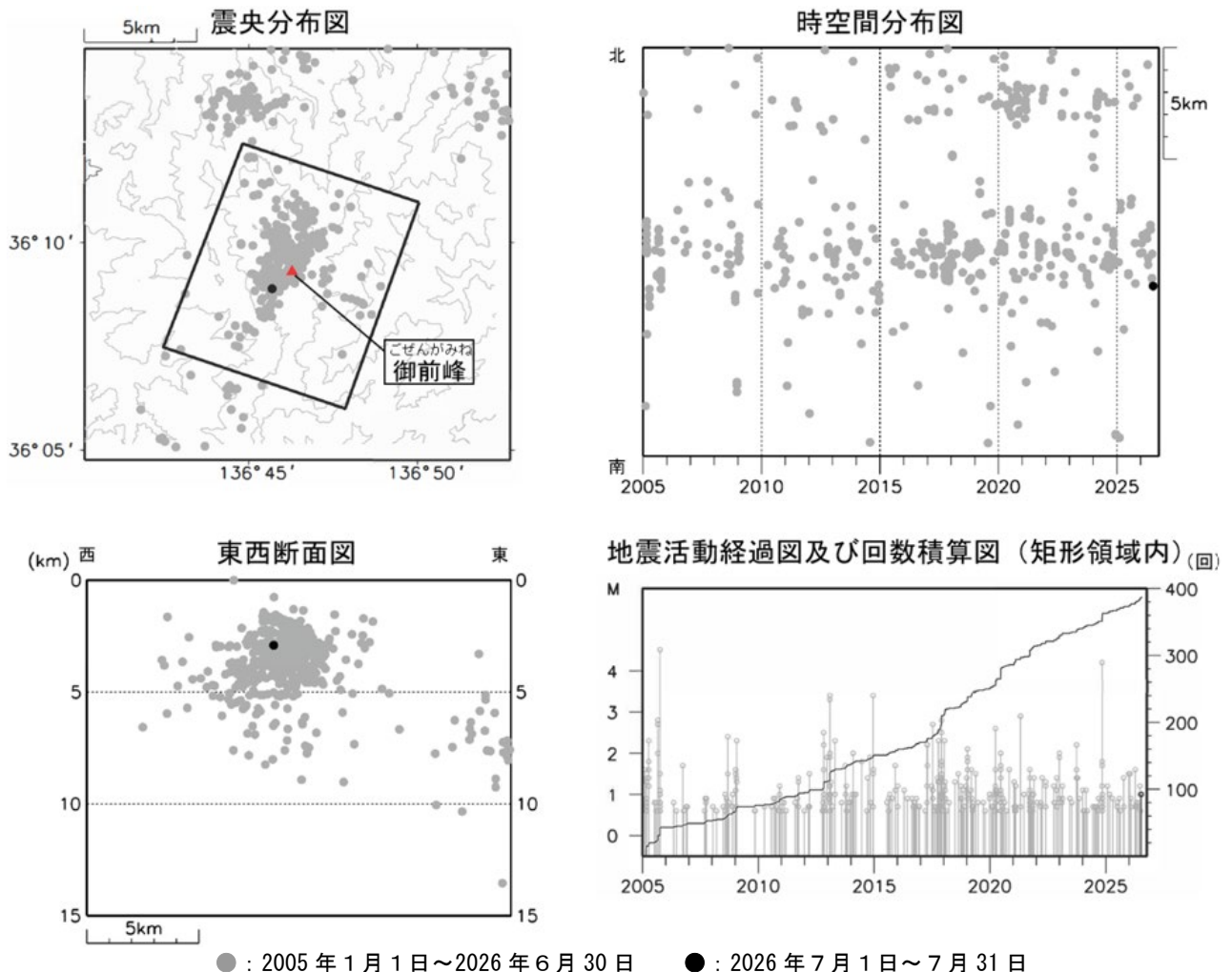
図4 白山 広域地震観測網による山体・周辺の地震活動（2005年1月1日～2026年7月31日）
