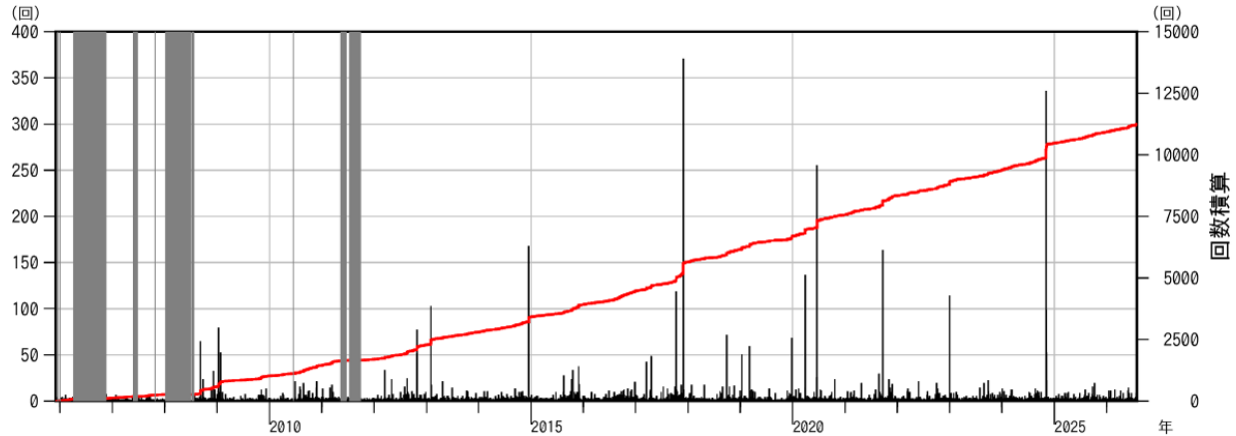
図3 白山 日別地震回数と積算回数（2005年12月1日～2026年7月31日）
