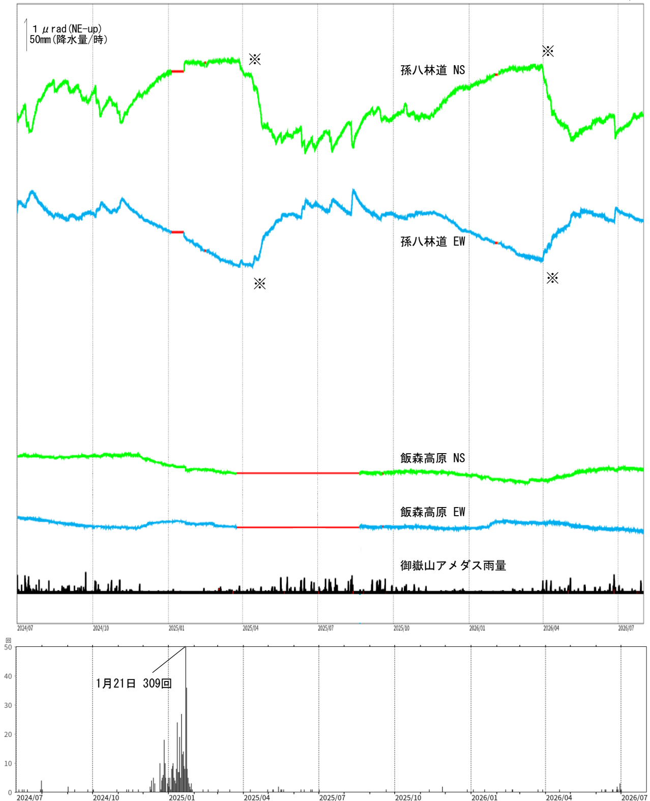
図8 御嶽山 傾斜変動と日別地震回数の推移（2024年7月1日～2026年7月31日）
