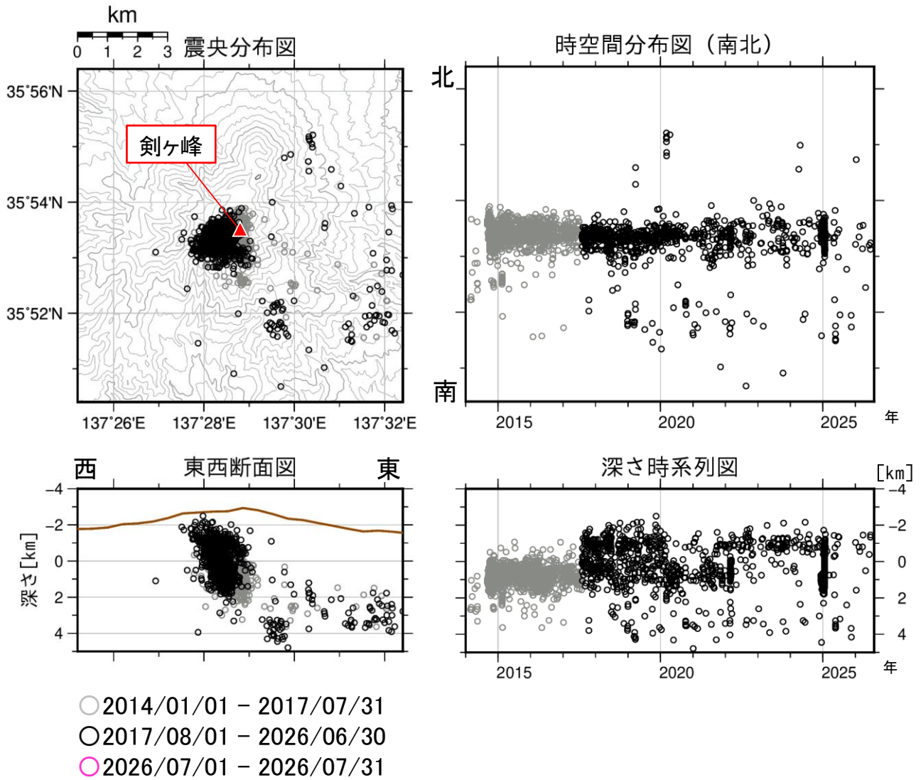
図5 御嶽山 震源分布図（2014年1月1日～2026年7月31日）
