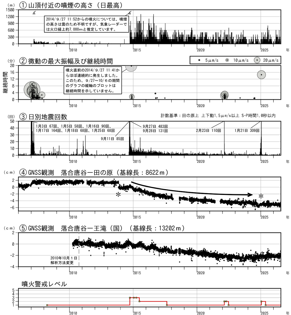
図1 御嶽山 長期間の火山活動経過図（2006年1月1日～2026年7月31日）
