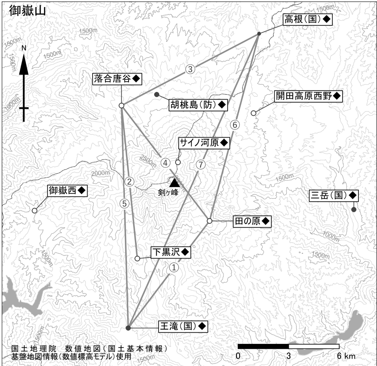
図7 御嶽山 GNSS 連続観測点と基線番号
