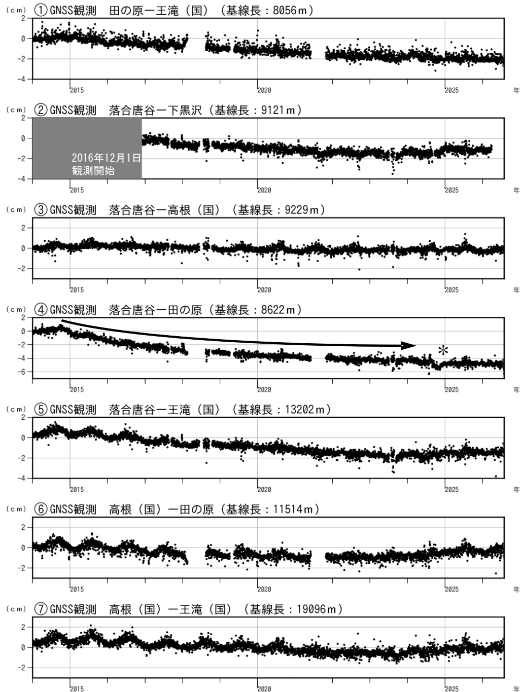
図6 御嶽山 GNSS 連続観測結果（2014年1月1日～2026年7月31日）
