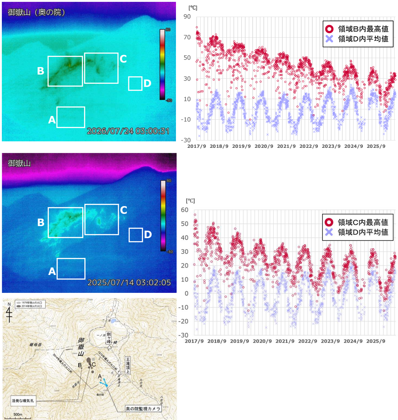
図3 御嶽山 奥の院赤外熱映像カメラによる地獄谷火口における最高温度の推移 (2017年9月13日～2026年7月31日)
