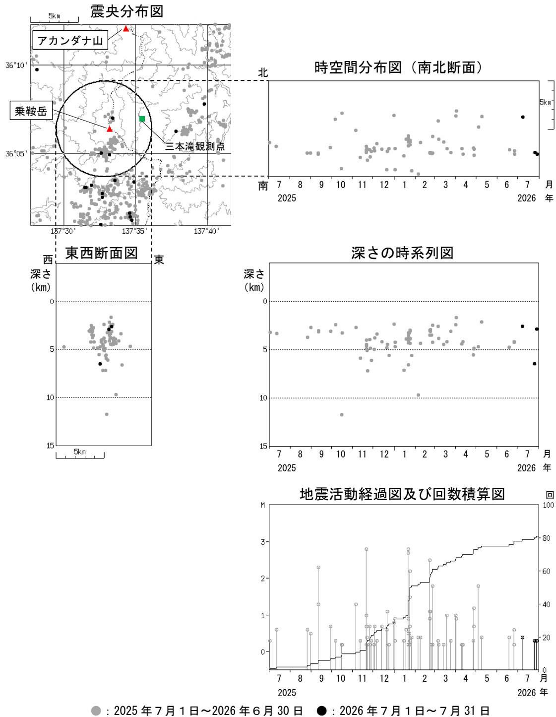
図3 乗鞍岳 広域地震観測網による山体・周辺の地震活動(2025年7月1日～2026年7月31日)
