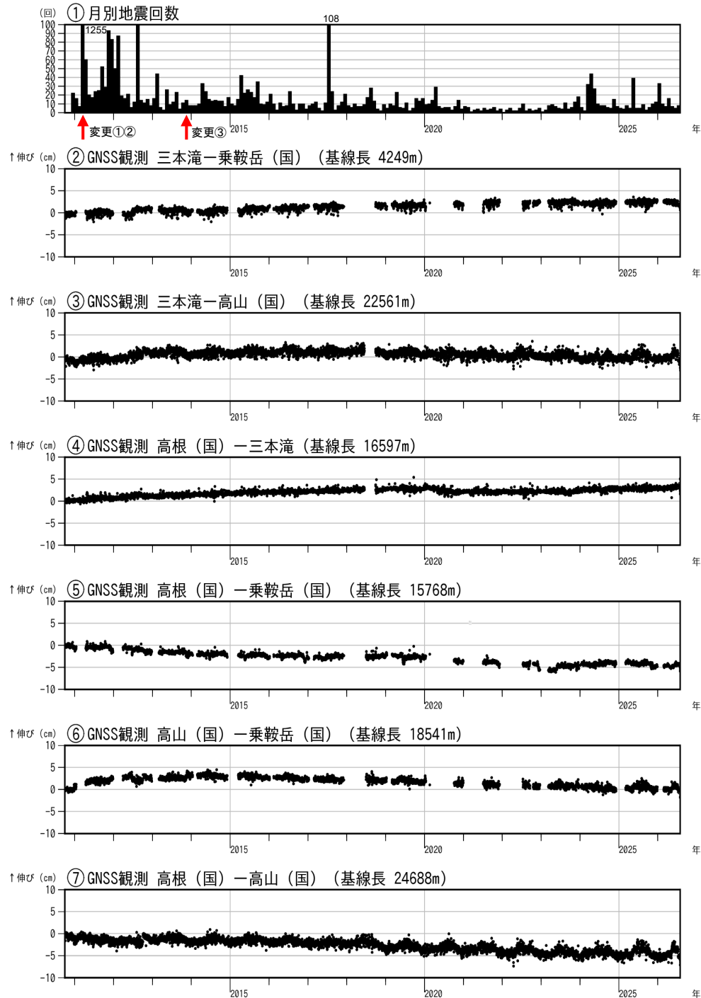
図2 乗鞍岳 火山活動経過図（2010年10月1日～2026年7月31日）
