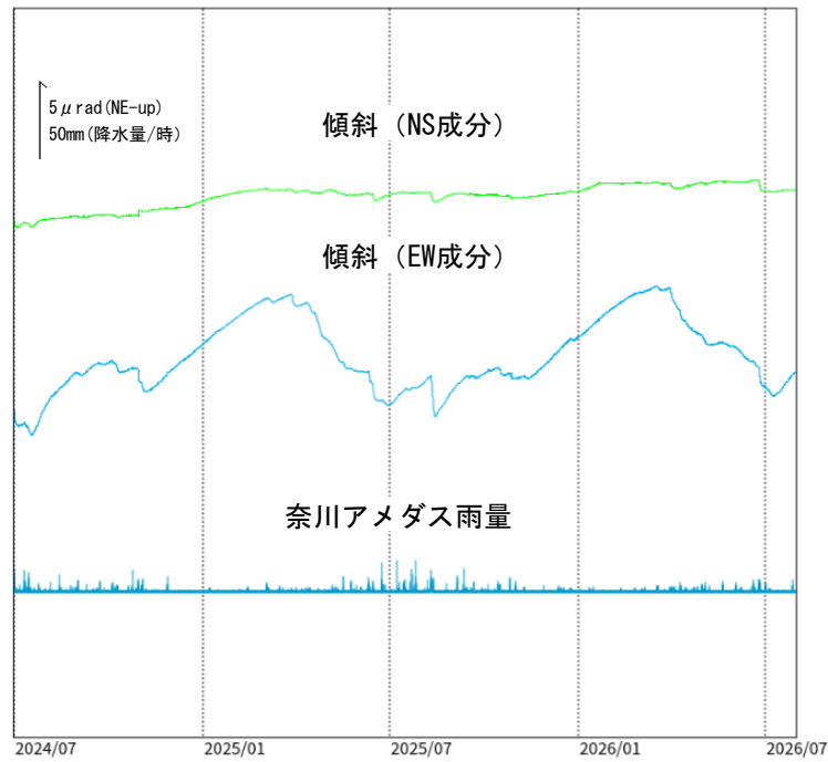
図4 乗鞍岳 三本滝観測点における傾斜データ（2024年7月1日～2026年7月31日） ・傾斜計による観測では、火山活動によるとみられる変動は認められません。
