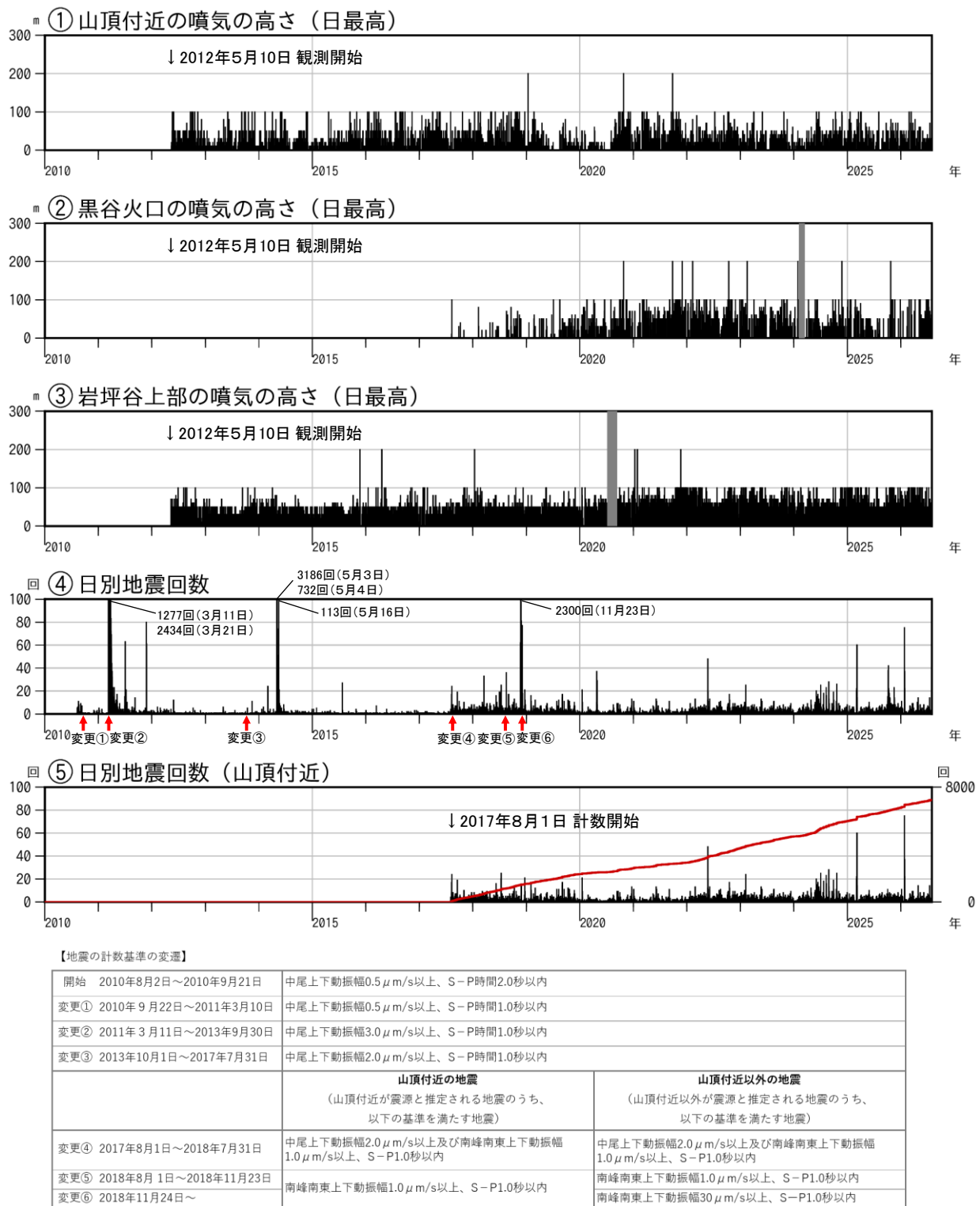
図5 焼岳 噴気の高さと地震回数の推移(2010年8月2日～2026年7月31日)
