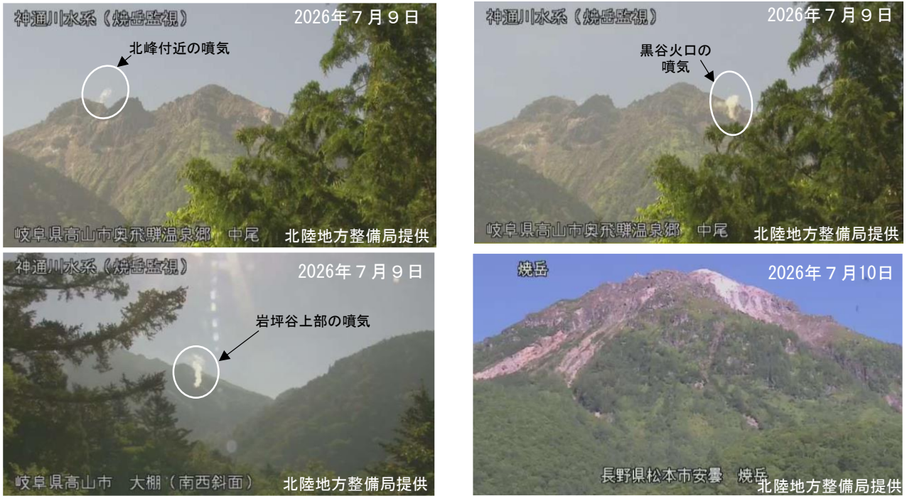
図3 焼岳 山頂部及び南西斜面の状況
