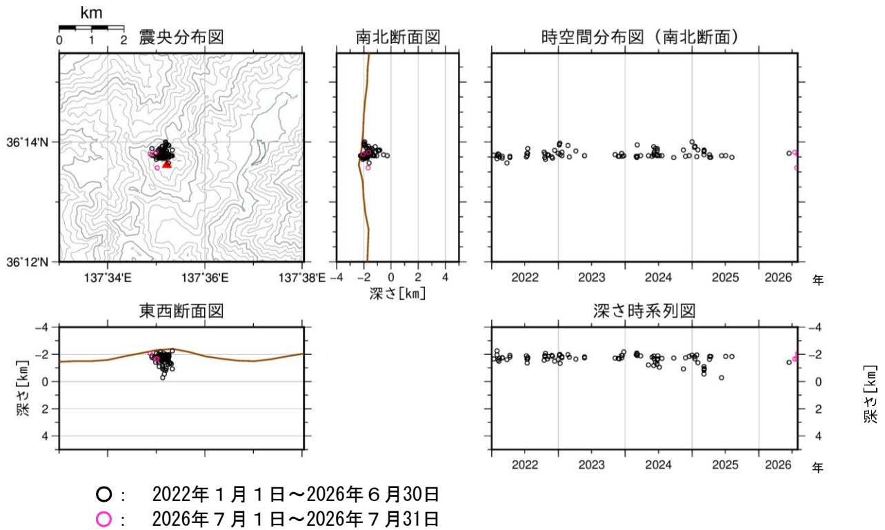
図2 焼岳 山頂付近の地震の震源分布図（2022年1月1日～2026年7月31日）
