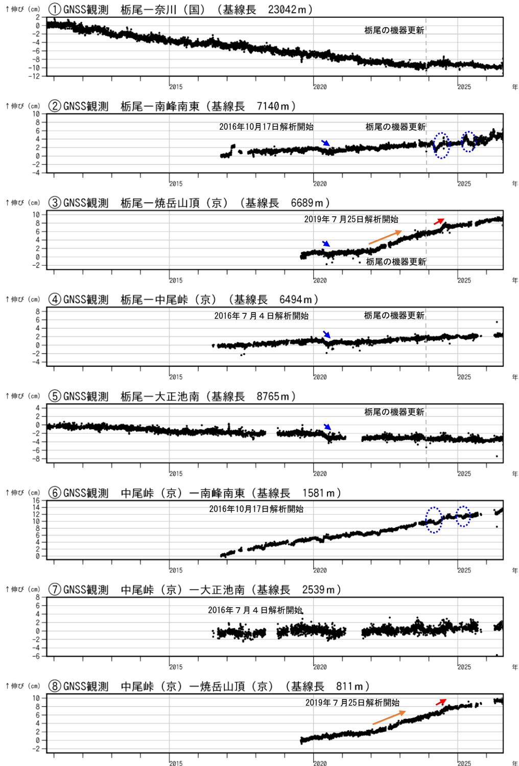
図6 焼岳 GNSS 連続観測による基線長変化（2010年10月1日～2026年7月31日）
