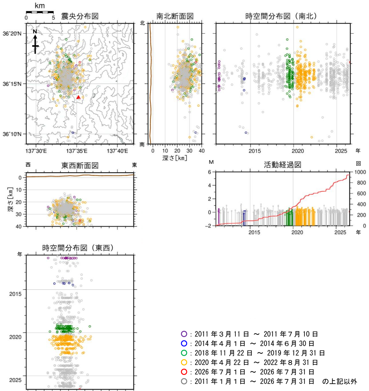
図10 焼岳 広域地震観測網による深部低周波地震の震源分布図（2011年1月1日～2026年7月31日）
