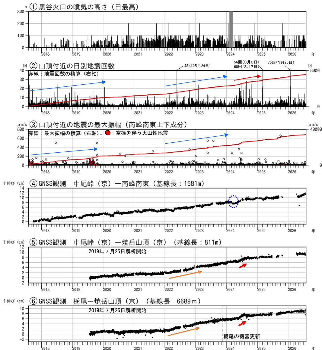
図1 焼岳 火山活動経過図（2017年8月1日～2026年7月31日）
