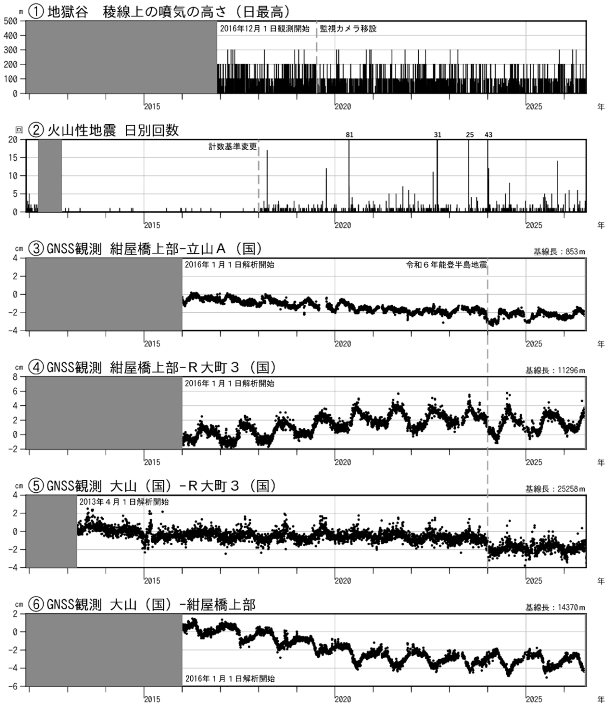
図3 弥陀ヶ原 火山活動経過図（2011年12月1日～2026年7月31日）
