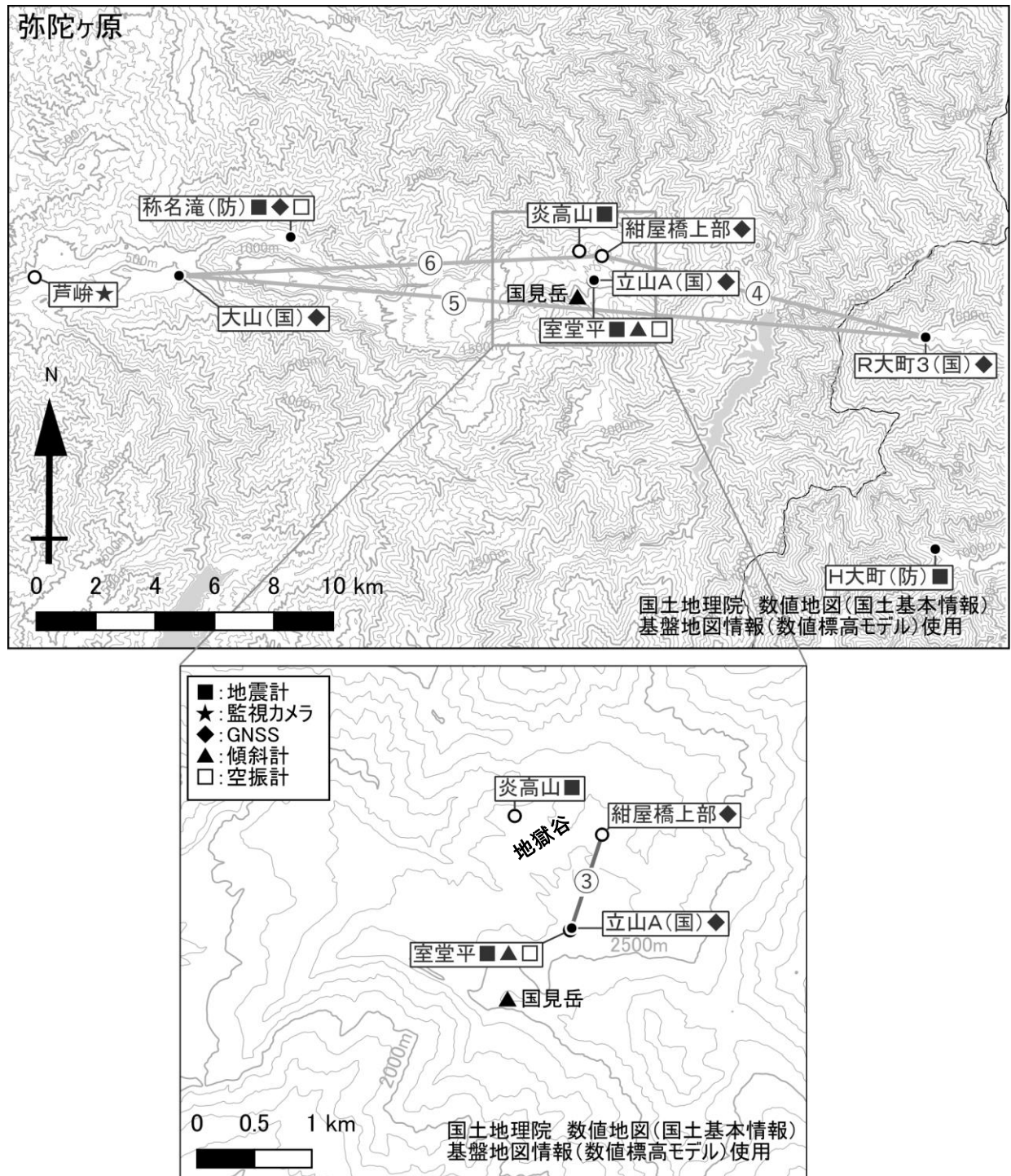
（国）：国土地理院、（防）：防災科学技術研究所。小さな白丸（○）は気象庁、小さな黒丸（●）は気象庁以外の機関の観測点位置を示しています。図中の GNSS 基線③～⑥は図 3 の③～⑥にそれぞれ対応しています。
