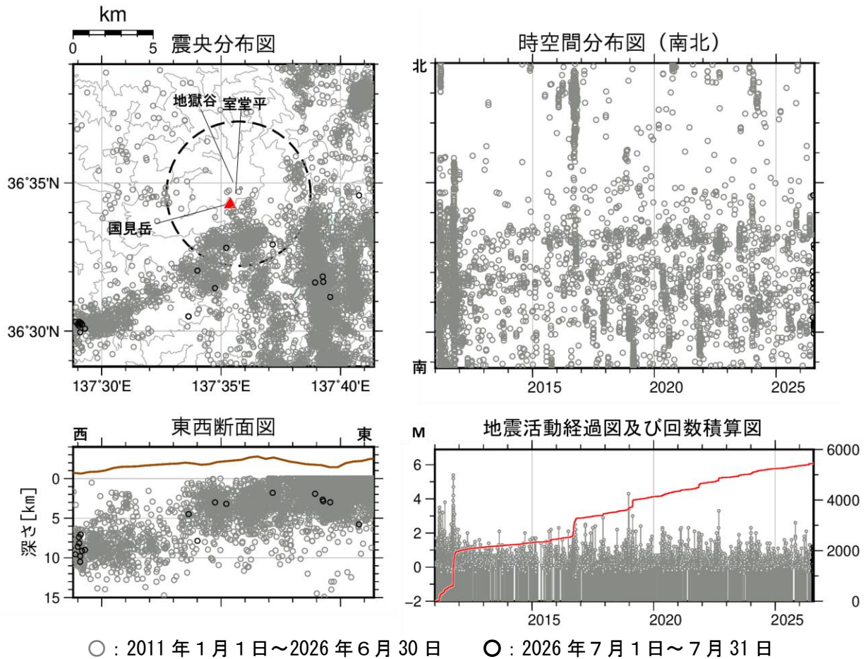
図2 弥陀ヶ原 広域地震観測網による山体・周辺の地震活動（2011年1月1日～2026年7月31日） 震央分布図中の円は弥陀ヶ原の計数対象地震（室堂平でS-P時間1秒以内）のおよその範囲を示しています。 広域地震観測網により震源決定したもので、深さは全て海面以下として決定しています。なお、2020年9月以降については、地震観測点の標高を考慮する等、震源決定の手法を変更しています。 図中の震源要素は一部暫定値が含まれており、後日変更することがあります。
