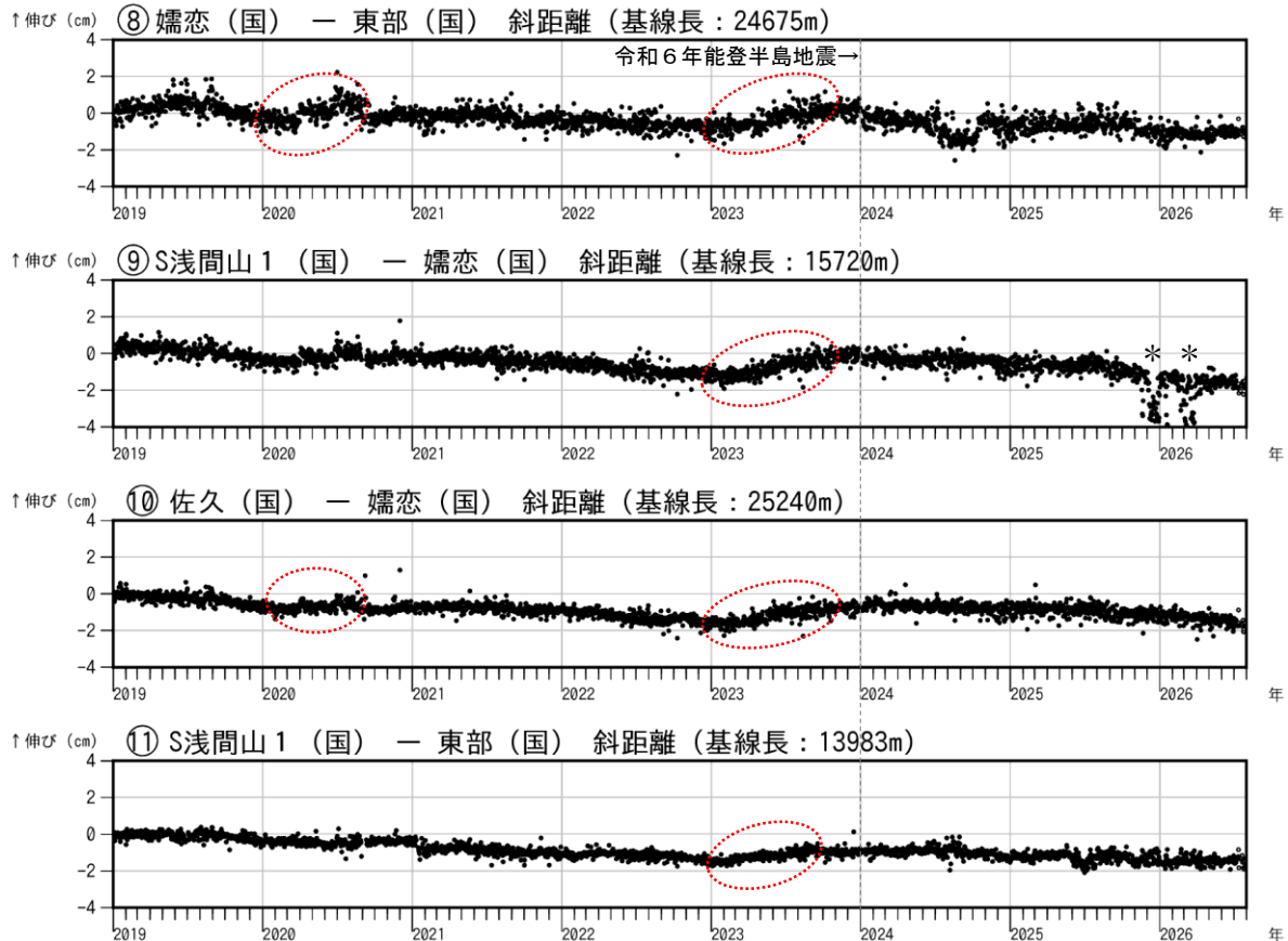
図7-2 浅間山 GNSS 連続観測結果(2019年1月1日～2026年7月31日)
