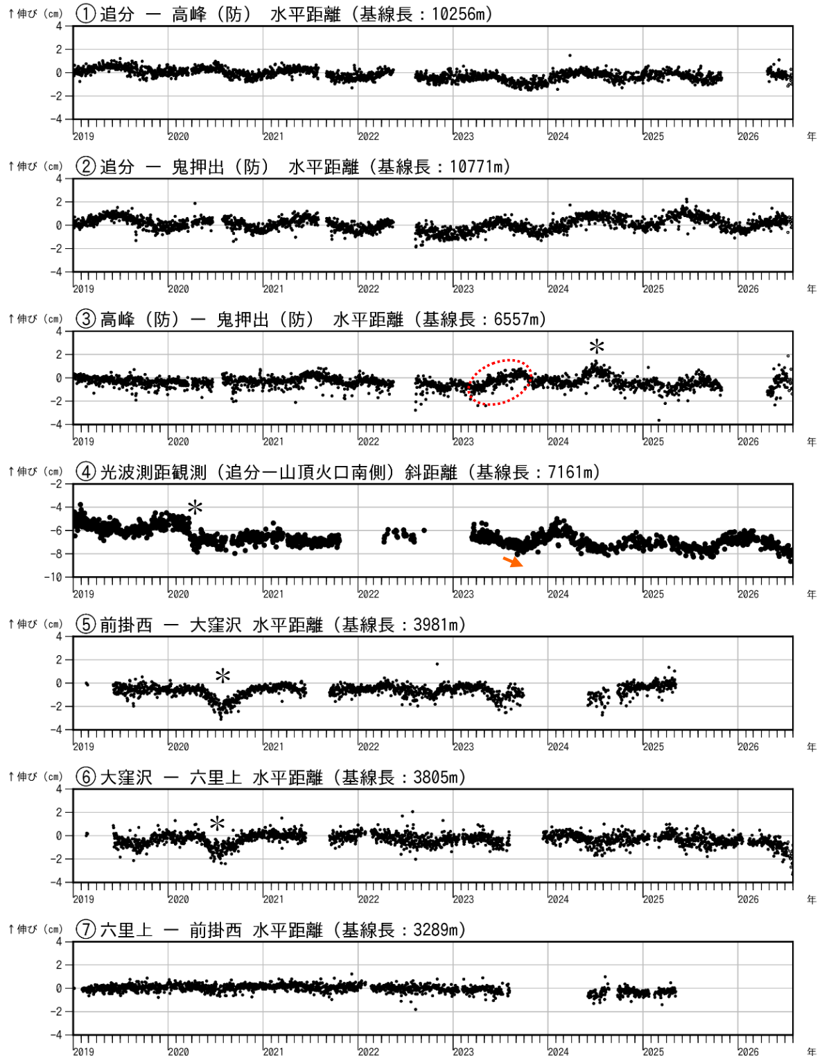
図7-1 浅間山 GNSS 連続観測及び光波測距観測結果(2019年1月1日~2026年7月31日)
