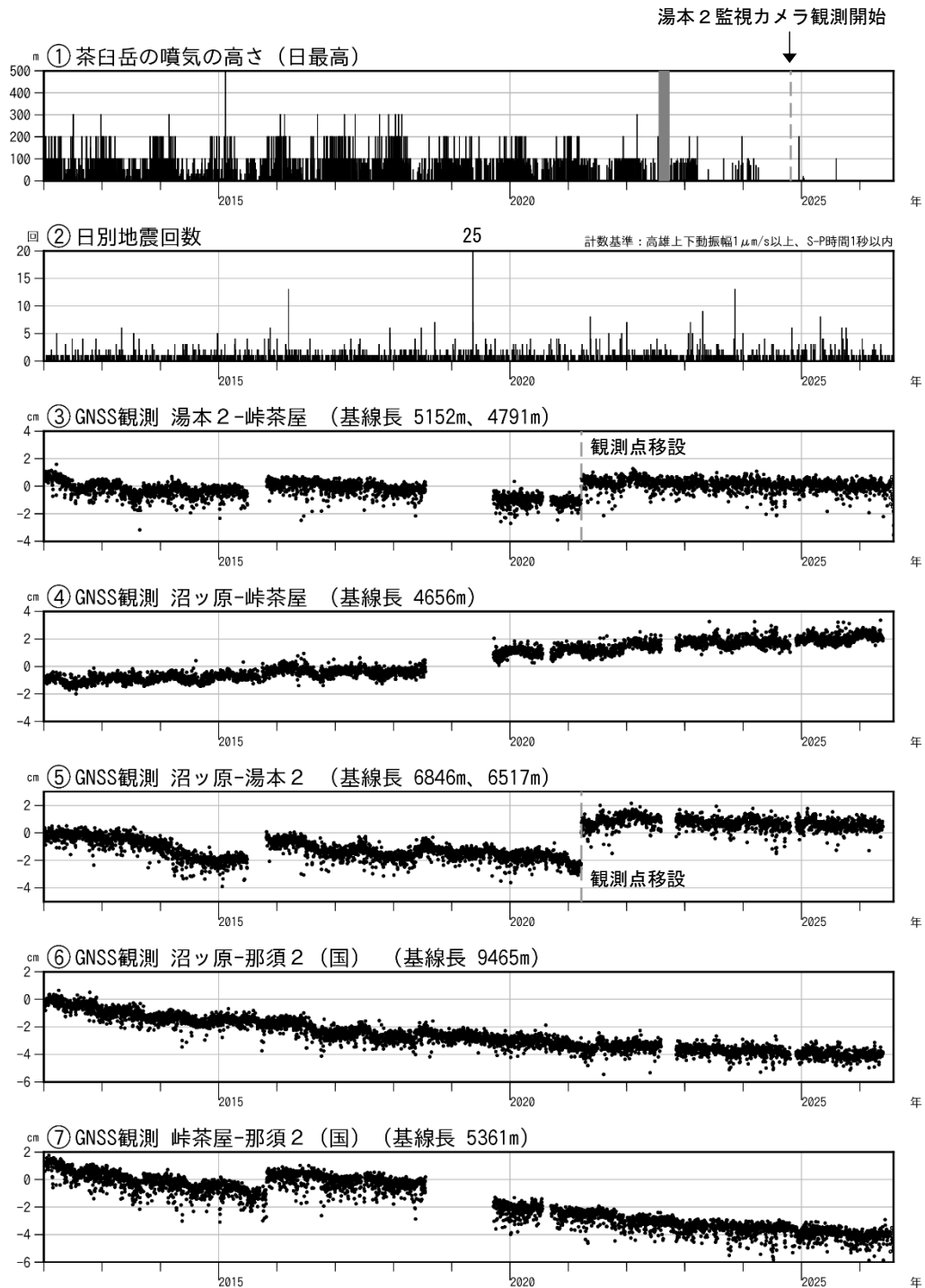
図4 那須岳 火山活動経過図（2012年1月1日～2026年7月31日）
