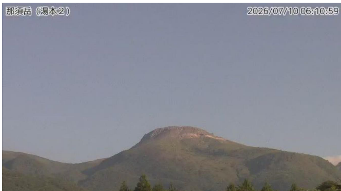
図1 那須岳 茶臼岳の状況（7月10日、湯本2監視カメラによる）
