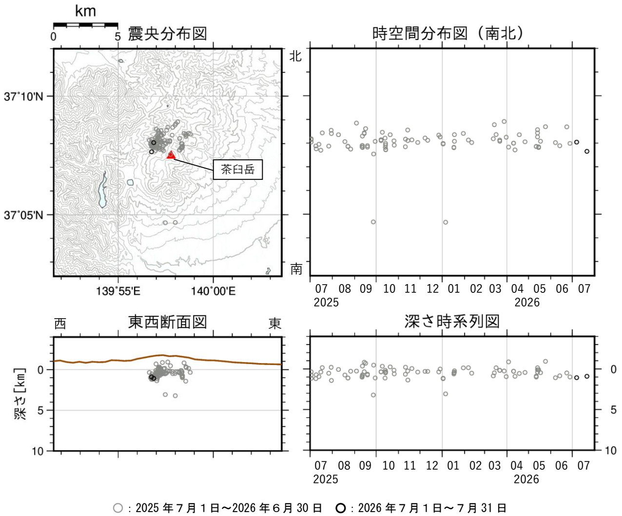
図5 那須岳 震源分布図（2025 年 7 月 1 日～2026 年 7 月 31 日）
