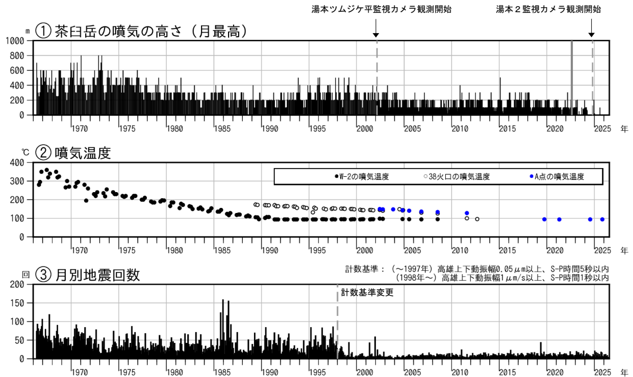
図3-1 那須岳 火山活動経過図（1966年6月～2026年7月）
