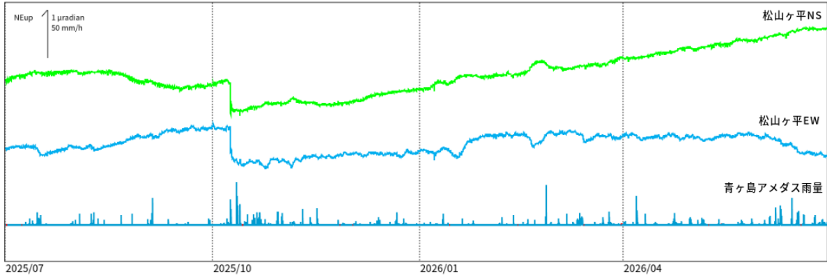
図4 青ヶ島 松山ヶ平観測点における傾斜データ（2025年7月1日～2026年6月30日） ・傾斜計による観測では、火山活動によるとみられる変動は認められません。
