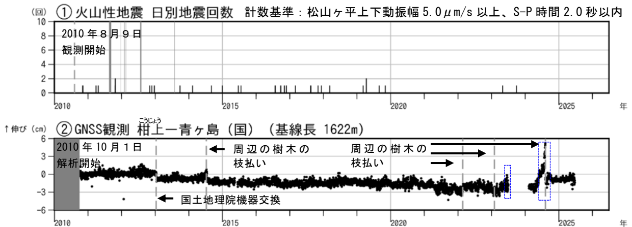
図3 青ヶ島 火山活動経過図（2010年8月9日～2026年6月30日） ① グラフの灰色部分は機器障害による欠測を示す。 ② （国）：国土地理院、図5のGNSS基線②に対応。グラフの空白部分は柑上の障害による欠測を示す。青破線内の期間に見られる変化は、柑上観測点周囲の樹木によるものです。
