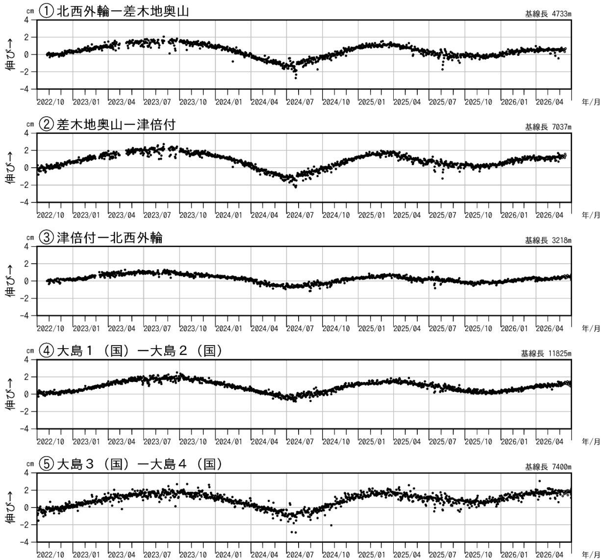
図3-2 伊豆大島 GNSS連続観測による基線長変化(2022年10月～2026年6月)
