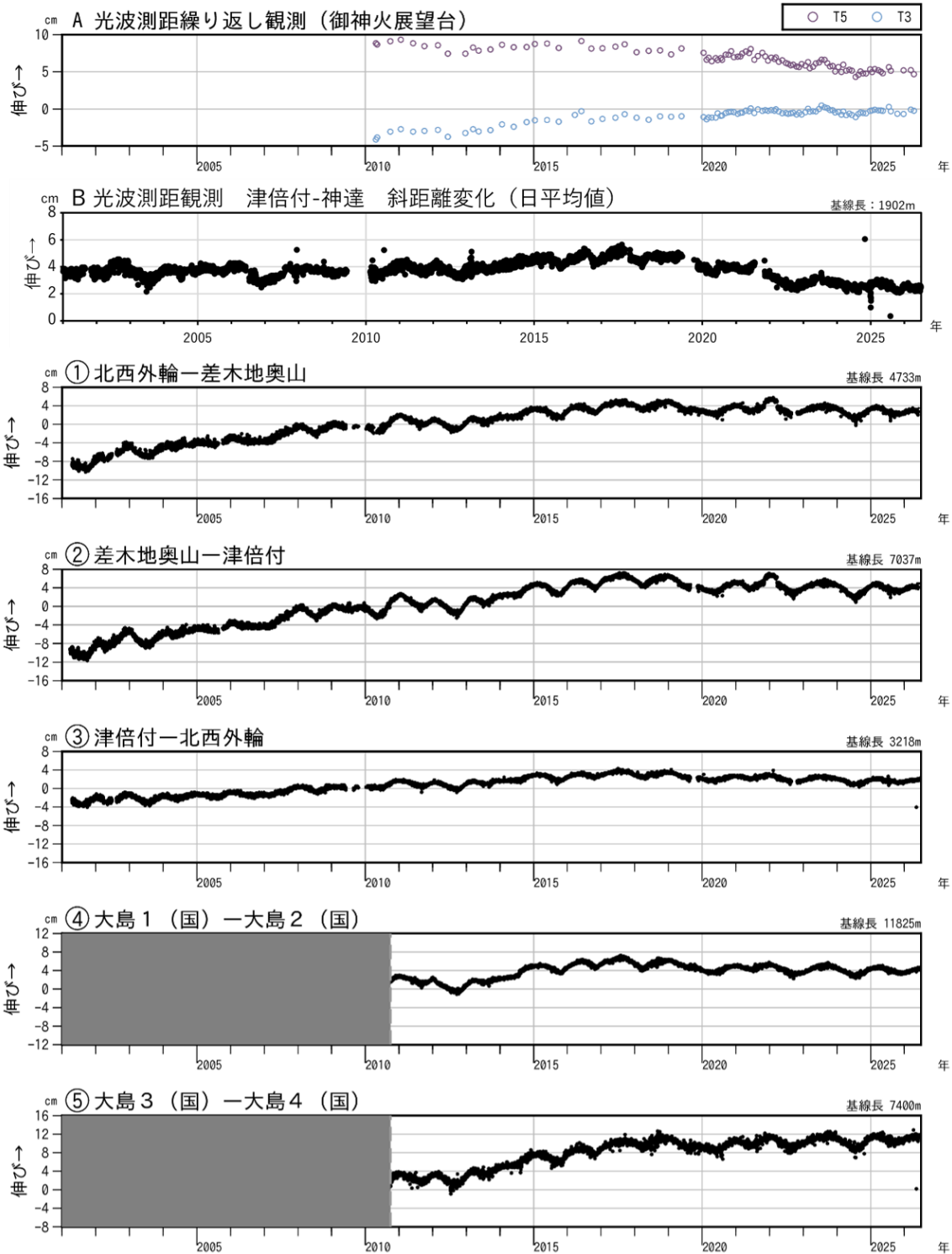
図3-1 伊豆大島 GNSS連続観測及び光波測距観測による基線長変化(2001年1月～2026年6月)
