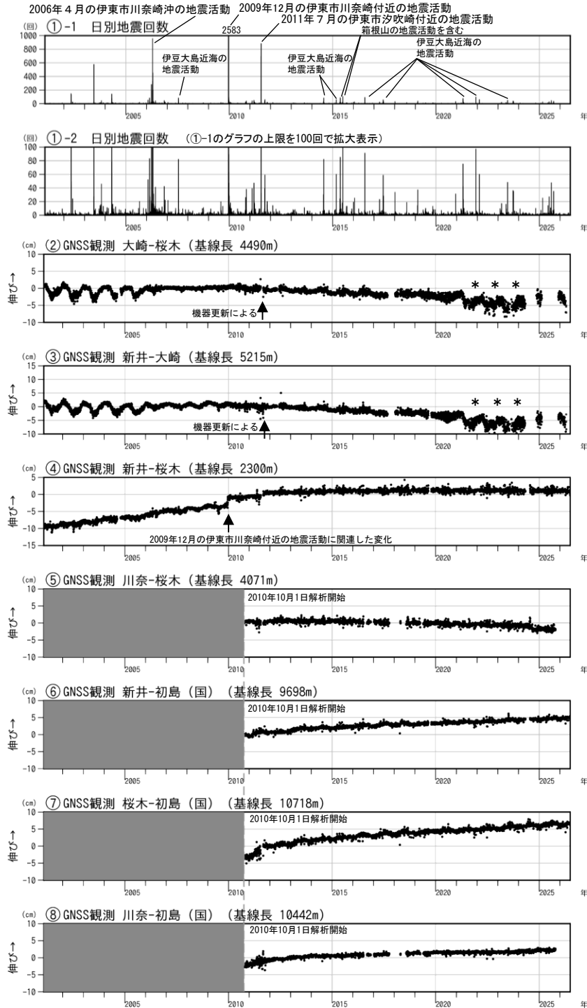
図3 伊豆東部火山群 火山活動経過図（2001年2月1日～2026年6月30日）
