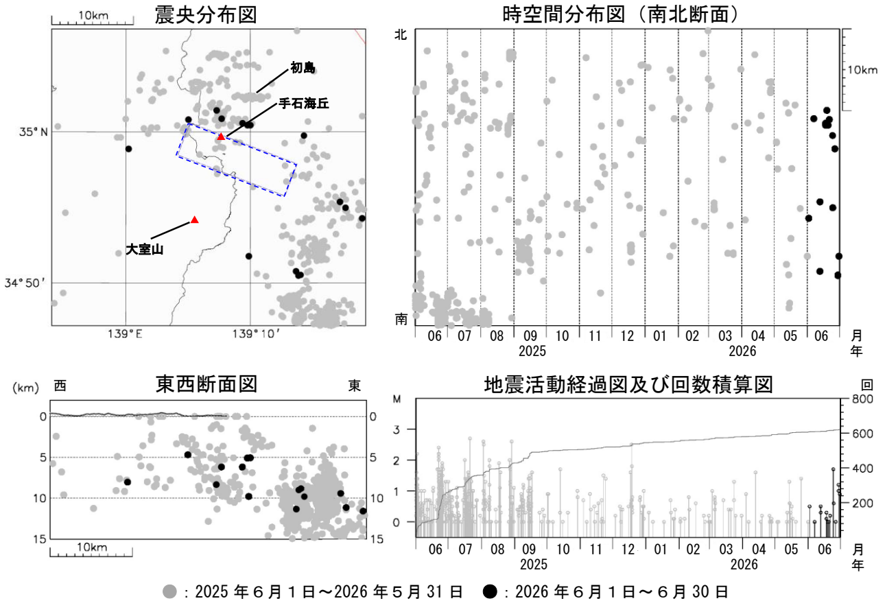
図2 伊豆東部火山群 広域地震観測網による震源分布図（2025年6月1日～2026年6月30日） □の領域は群発地震活動の発生する可能性がある範囲（火口が出現する可能性のある範囲）を示しています。 https://www.data.jma.go.jp/vois/data/filing/level/PDF/level_316.pdf 広域地震観測網により震源決定したもので、深さは全て海面以下として決定しています。 M（マグニチュード）は地震の規模を表し、M0.0以上を表示しています。 図中の震源要素は一部暫定値が含まれており、後日変更することがあります。 この図では、関係機関の地震波形を一元的に処理し、地震観測点の標高を考慮する等した手法で得られた震源を用いています。
