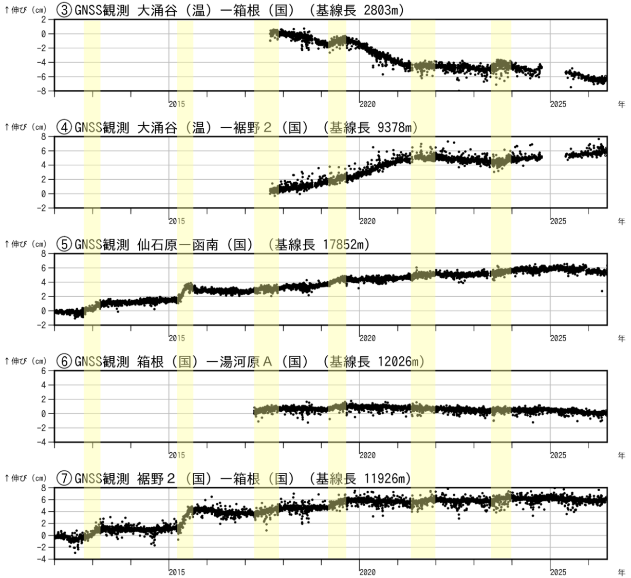
図3-2 箱根山 GNSS連続観測による 基線長変化及び観測点配置図 (2012年1月1日~2026年6月30日)
