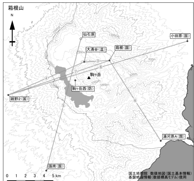
図3-2 箱根山 GNSS連続観測による 基線長変化及び観測点配置図 (2012年1月1日~2026年6月30日)
