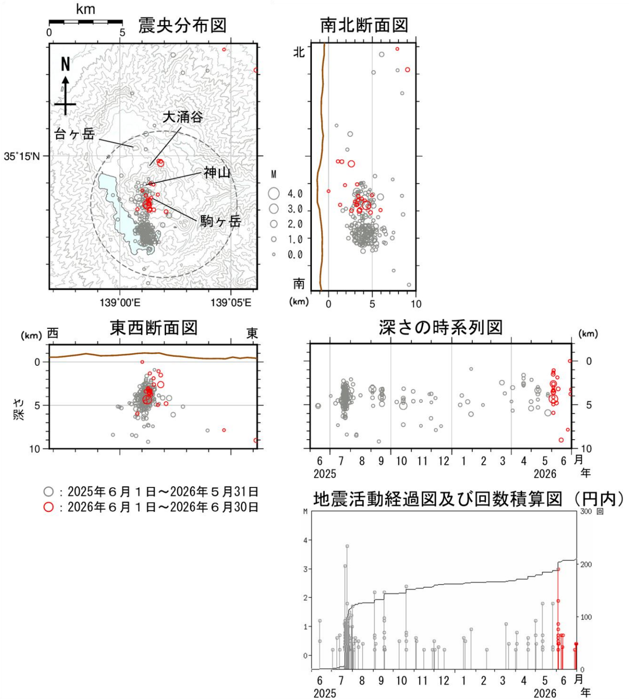
図4 箱根山 広域地震観測網による山体周辺の震源分布図（2025年6月1日～2026年6月30日）
