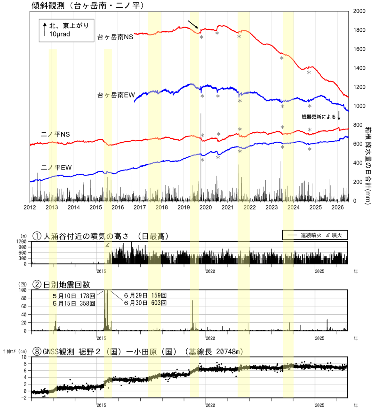
図3-1 箱根山 火山活動経過図（2012年1月1日～2026年6月30日）
