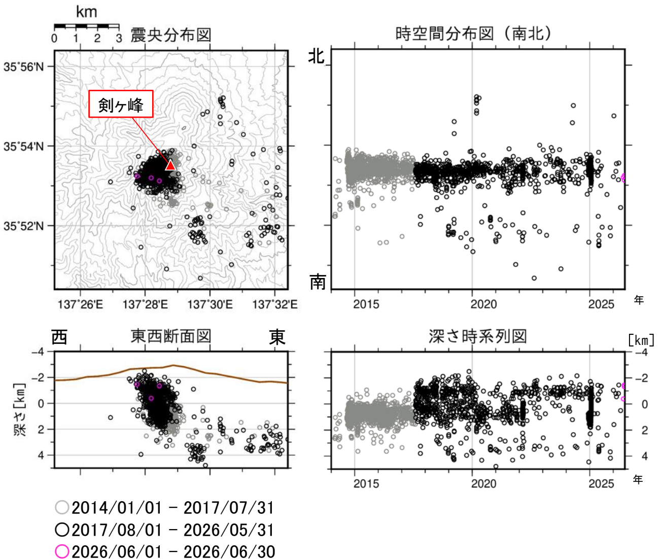
図5 御嶽山 震源分布図（2014年1月1日～2026年6月30日）
