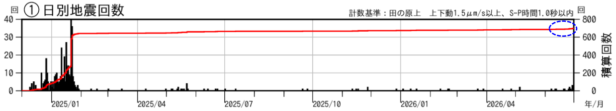
図4 御嶽山 日別地震回数（2024年12月1日～2026年6月30日）
