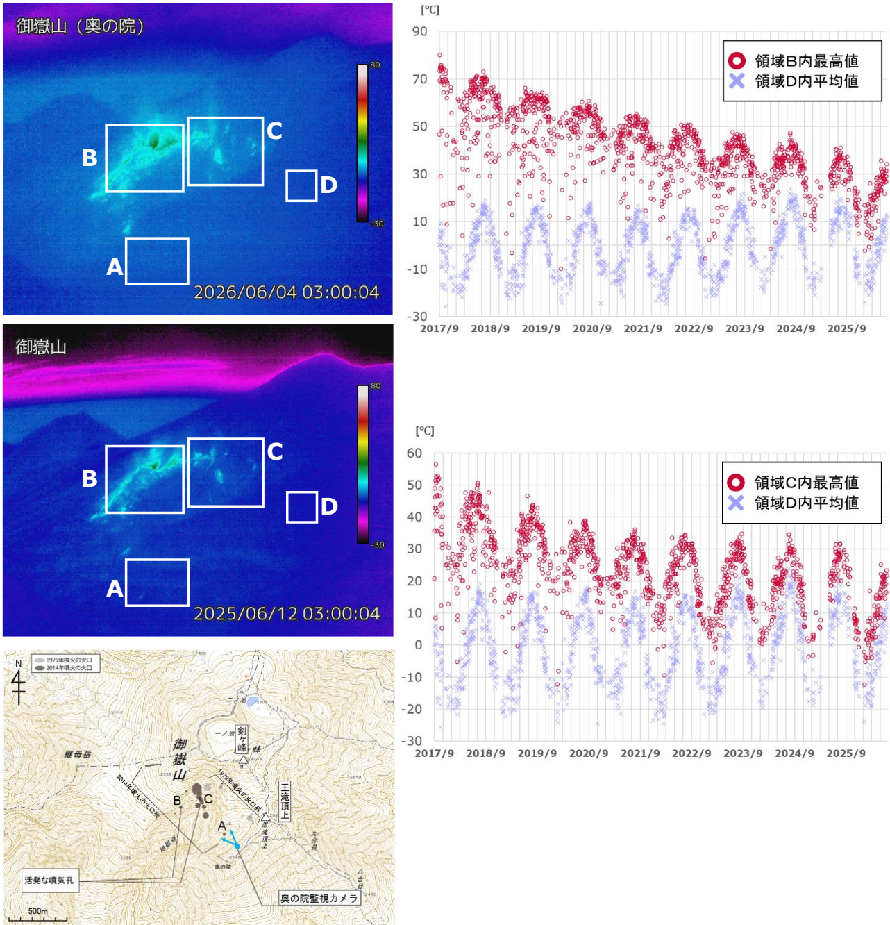
図3 御嶽山 奥の院赤外熱映像カメラによる地獄谷火口における最高温度の推移 (2017年9月13日～2026年6月30日)
