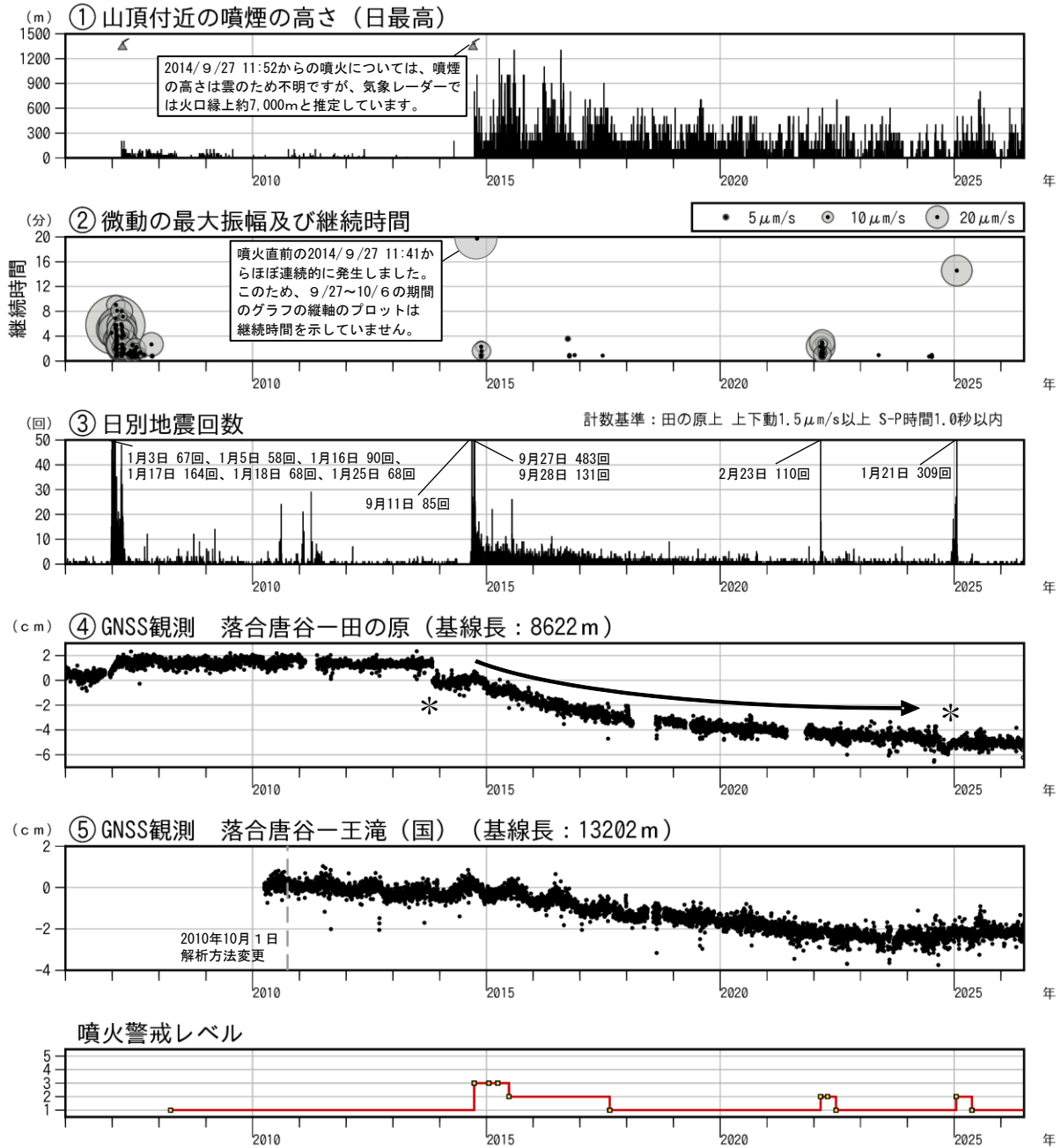
図1 御嶽山 長期間の火山活動経過図（2006年1月1日～2026年6月30日）
