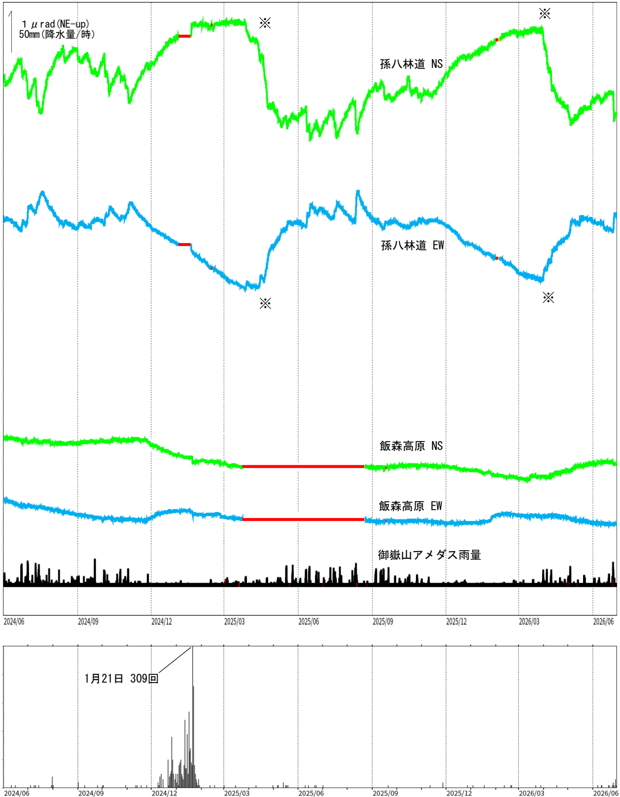
図8 御嶽山 傾斜変動と日別地震回数の推移（2024年6月1日～2026年6月30日）
