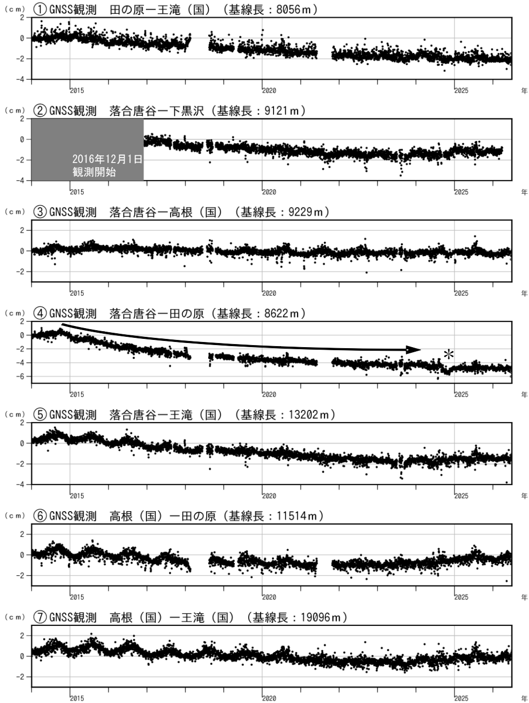
図6 御嶽山 GNSS連続観測結果（2014年1月1日～2026年6月30日）
