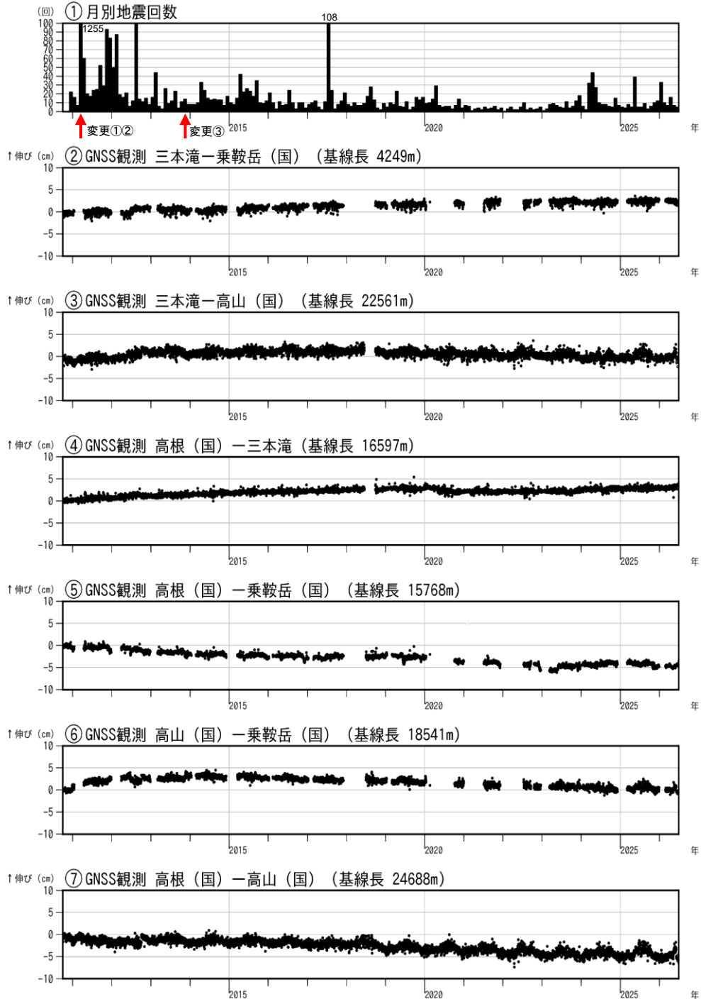
図2 乗鞍岳 火山活動経過図（2010年10月1日～2026年6月30日）
