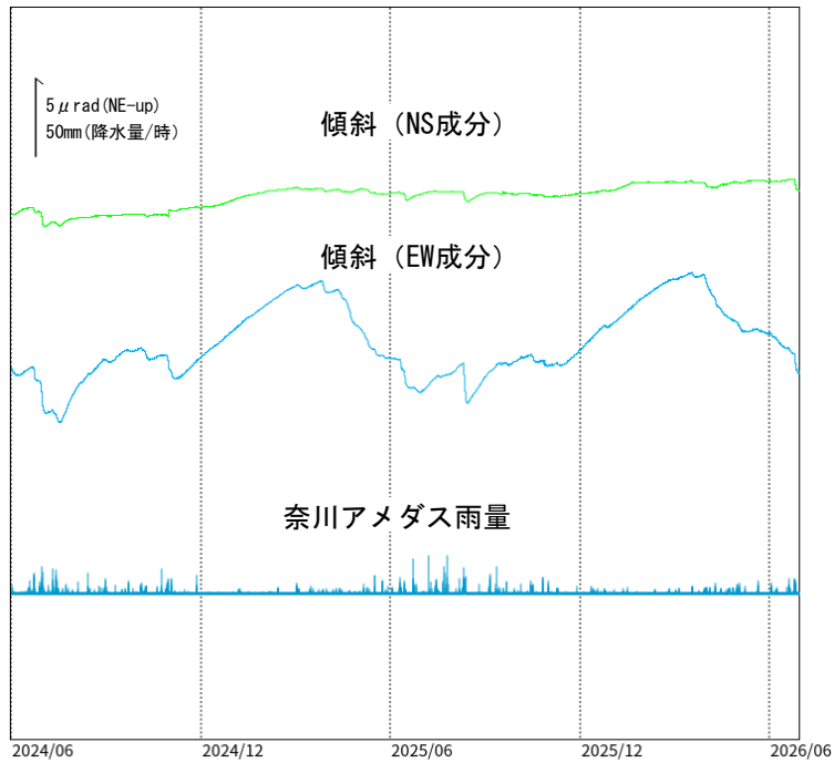
図4 乗鞍岳 三本滝観測点における傾斜データ (2024年6月1日~2026年6月30日) ・傾斜計による観測では、火山活動によるとみられる変動は認められません。
