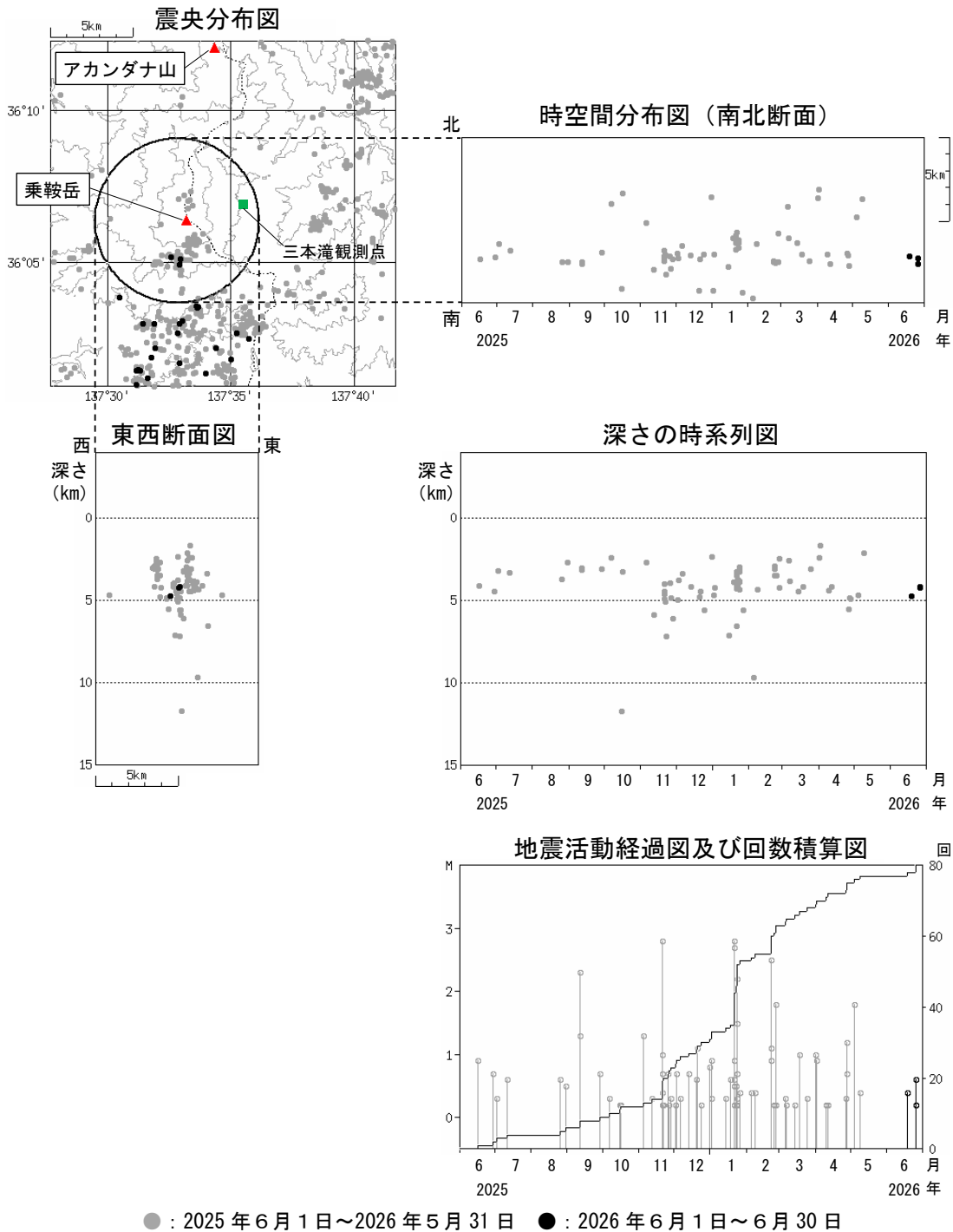
図3 乗鞍岳 広域地震観測網による山体・周辺の地震活動(2025年6月1日～2026年6月30日)
