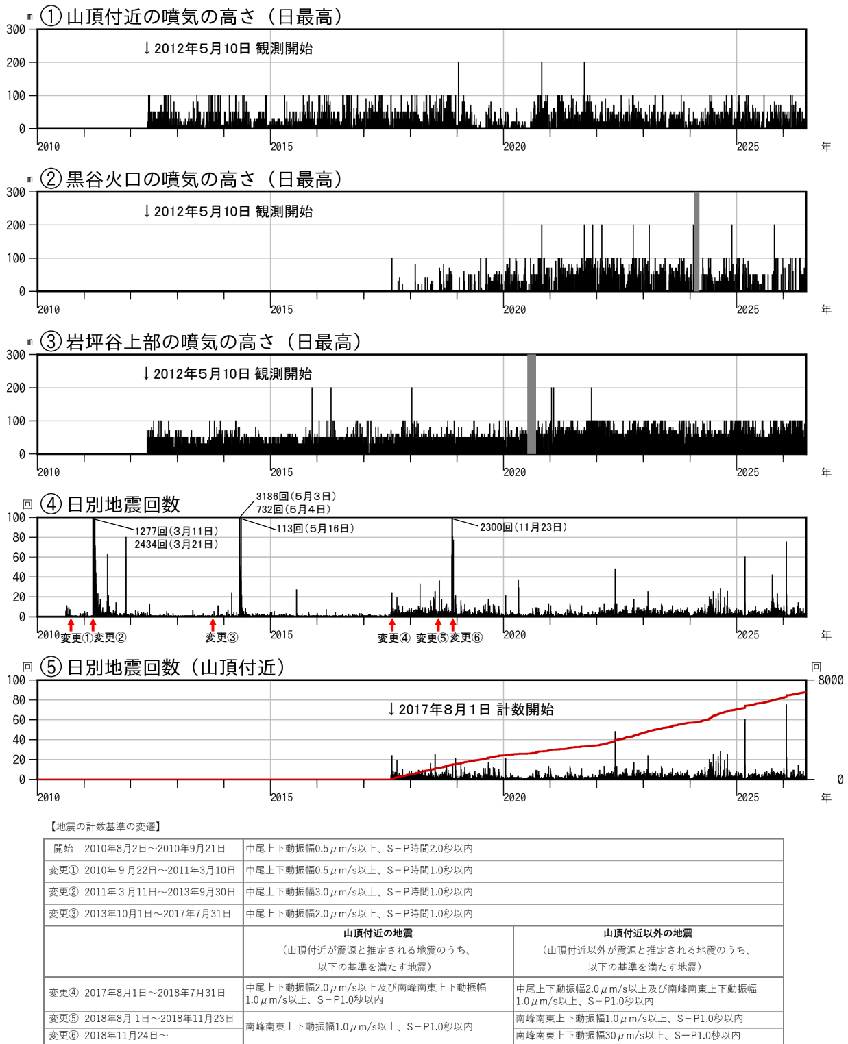
図5 焼岳 噴気の高さと地震回数の推移(2010年8月2日～2026年6月30日)
