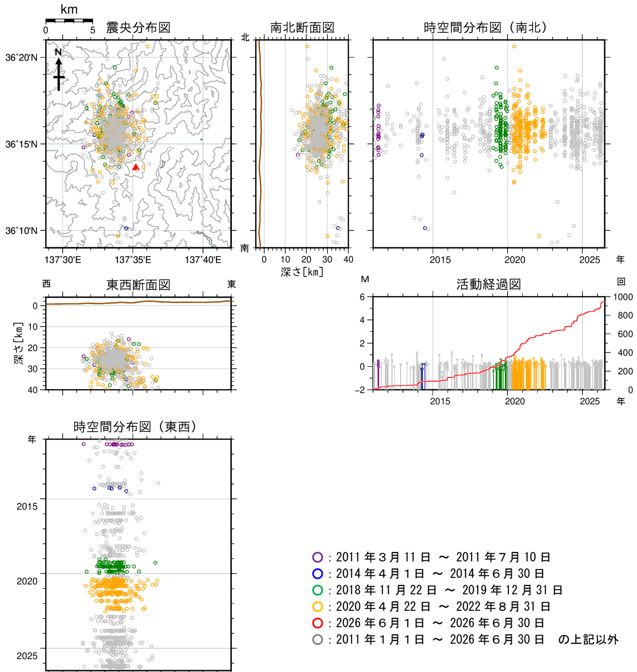
図10 焼岳 広域地震観測網による深部低周波地震の震源分布図（2011年1月1日～2026年6月30日）
