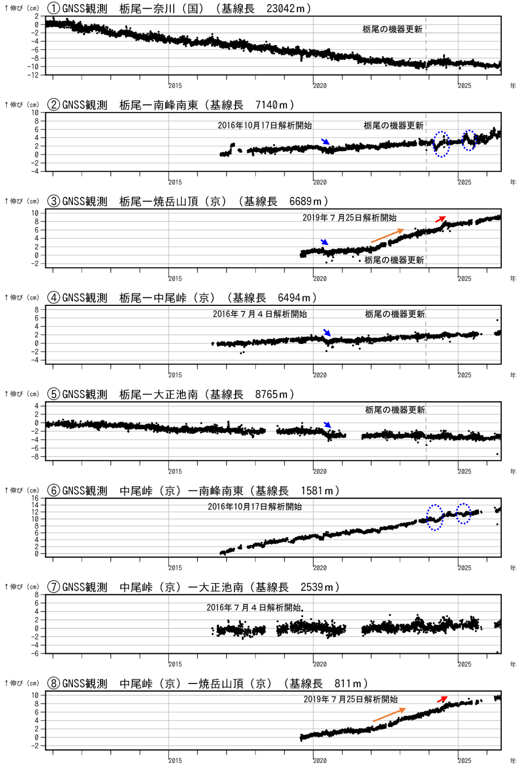
図6 焼岳 GNSS 連続観測による基線長変化（2010年10月1日～2026年6月30日）
