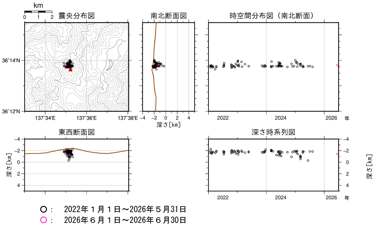
図2 焼岳 山頂付近の地震の震源分布図（2022年1月1日～2026年6月30日）
