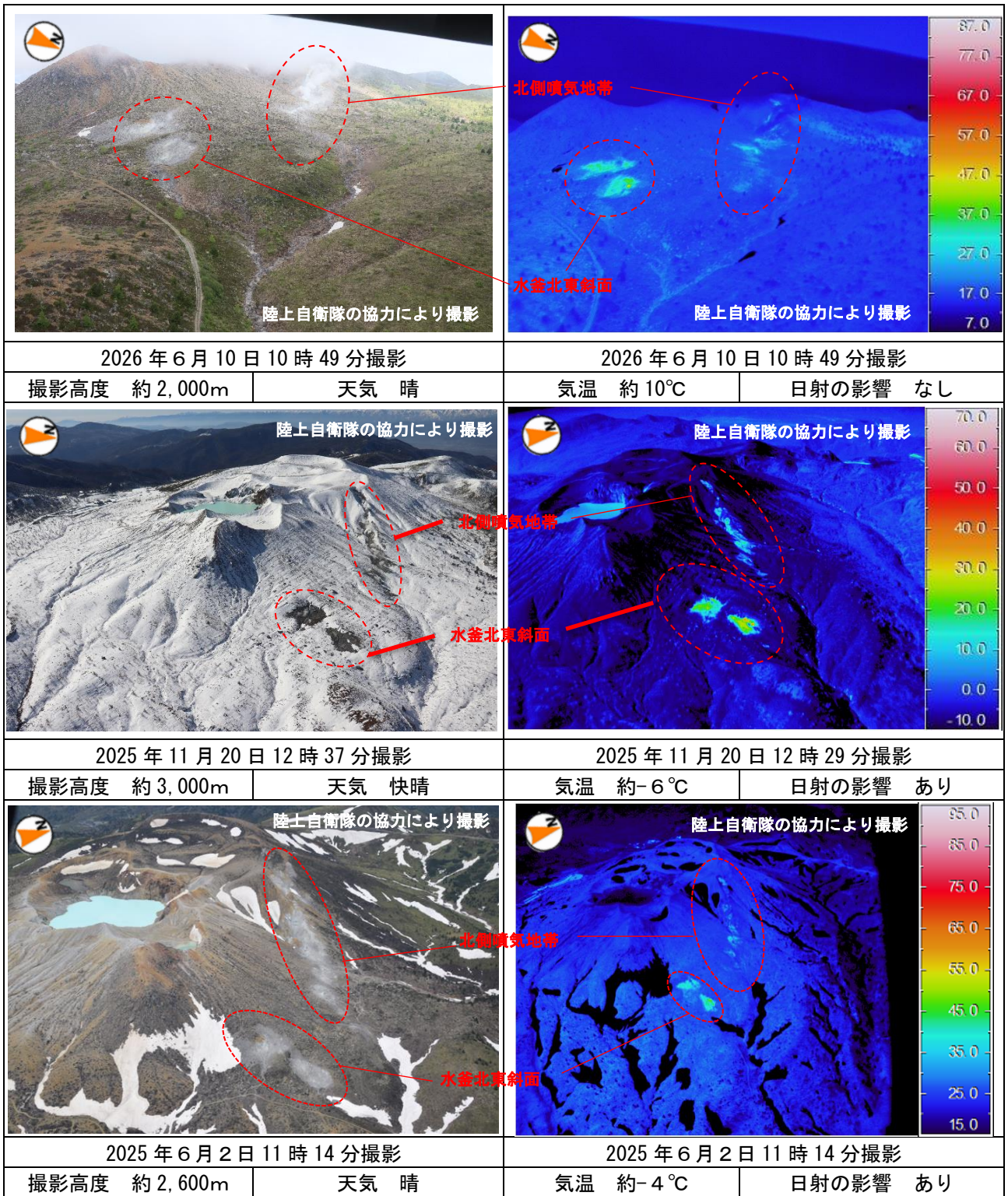
図1-7 草津白根山（白根山（湯釜付近）） 湯釜火口北側噴気地帯及び水釜北東斜面の状況
