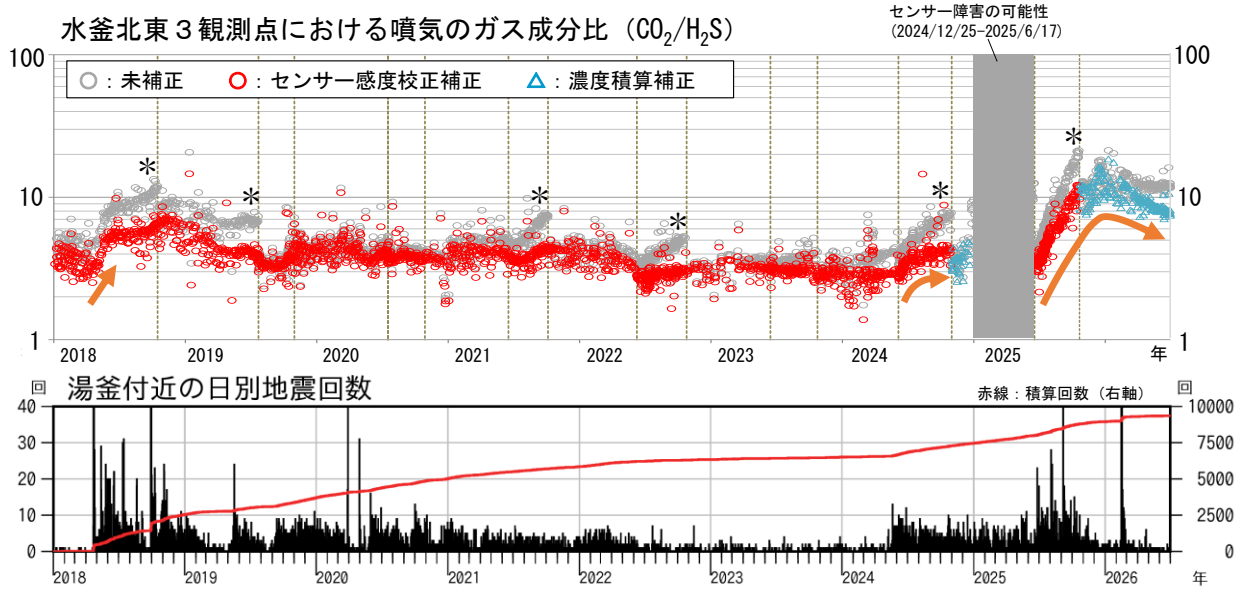
図2 草津白根山（白根山（湯釜付近）） 火山ガス観測結果（2018年1月～2026年6月30日）
