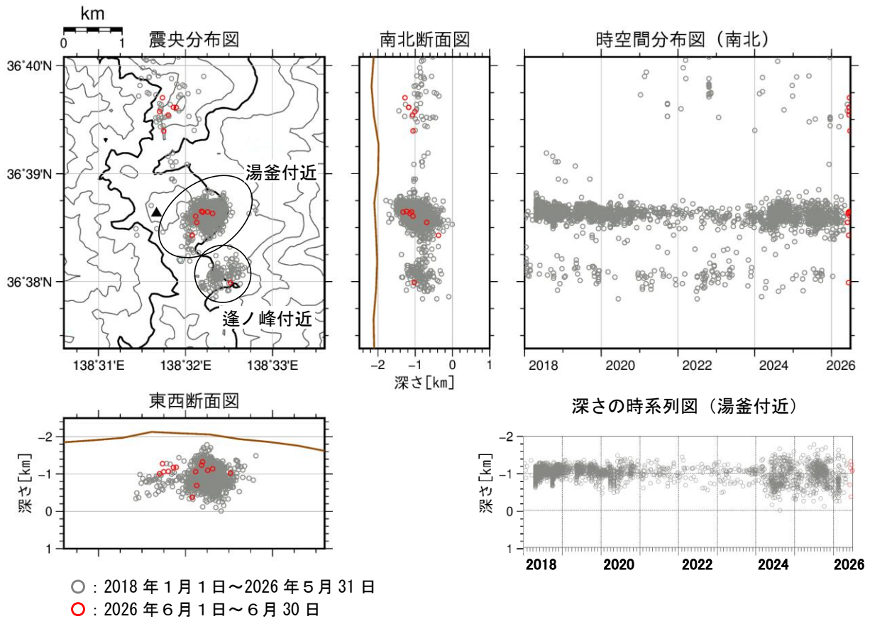
図4 草津白根山 震源分布図（2018年1月1日～2026年6月30日）
