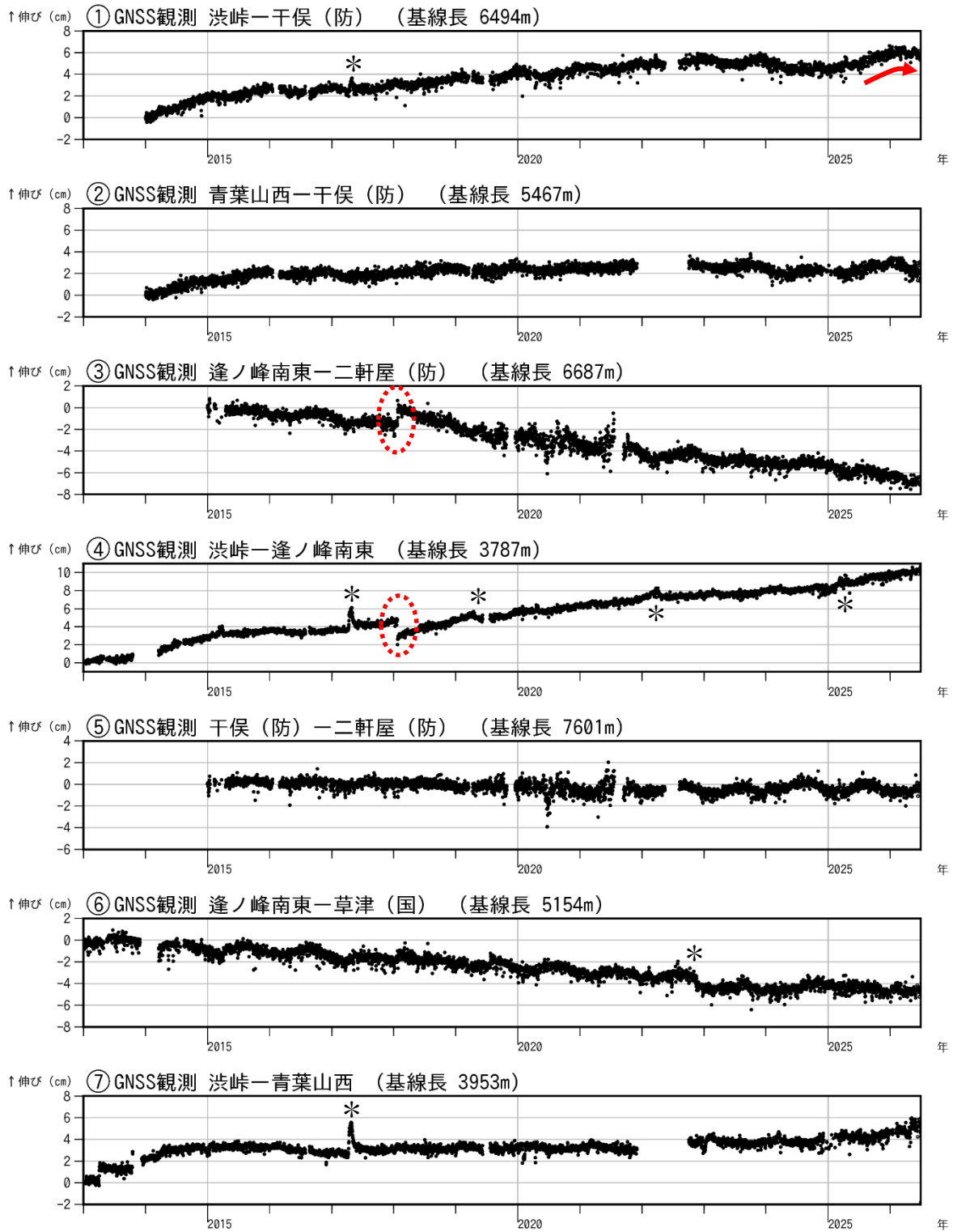
図6 草津白根山 GNSS 連続観測結果（2013年1月1日～2026年6月30日）
