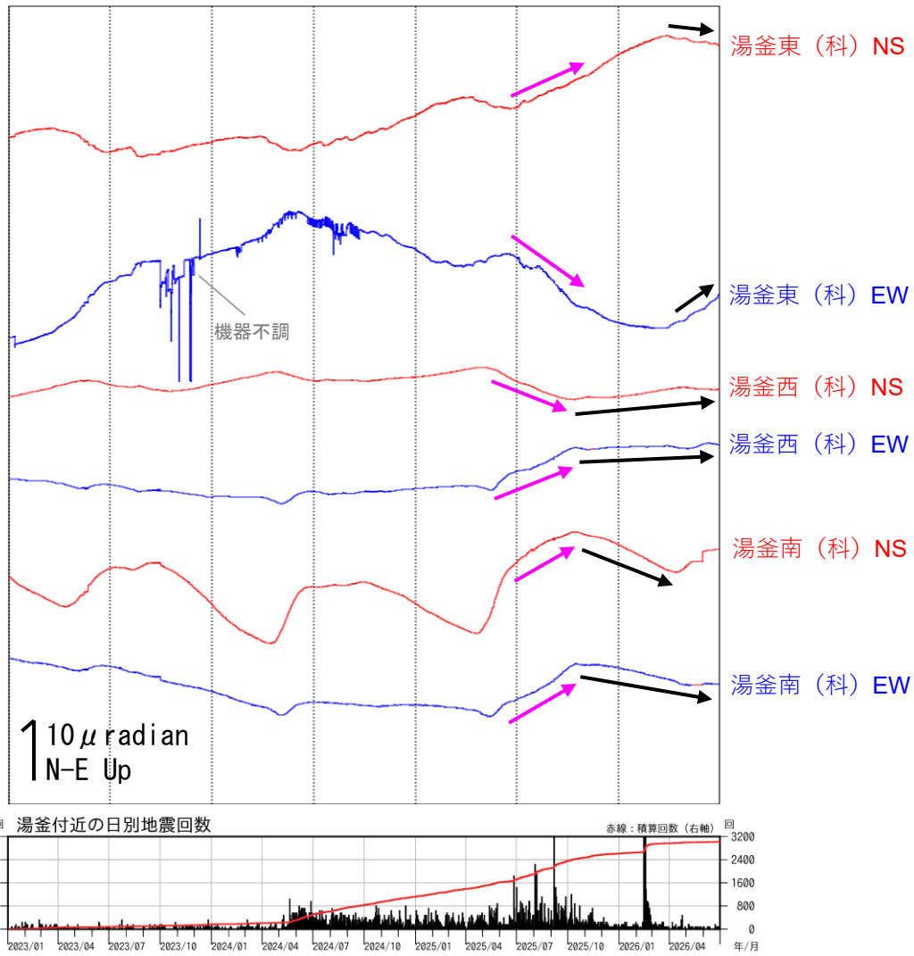
図5 草津白根山（白根山（湯釜付近）） 傾斜変動（2023年1月1日～2026年6月30日） データは時間平均値を使用しています。（科）：東京科学大学
