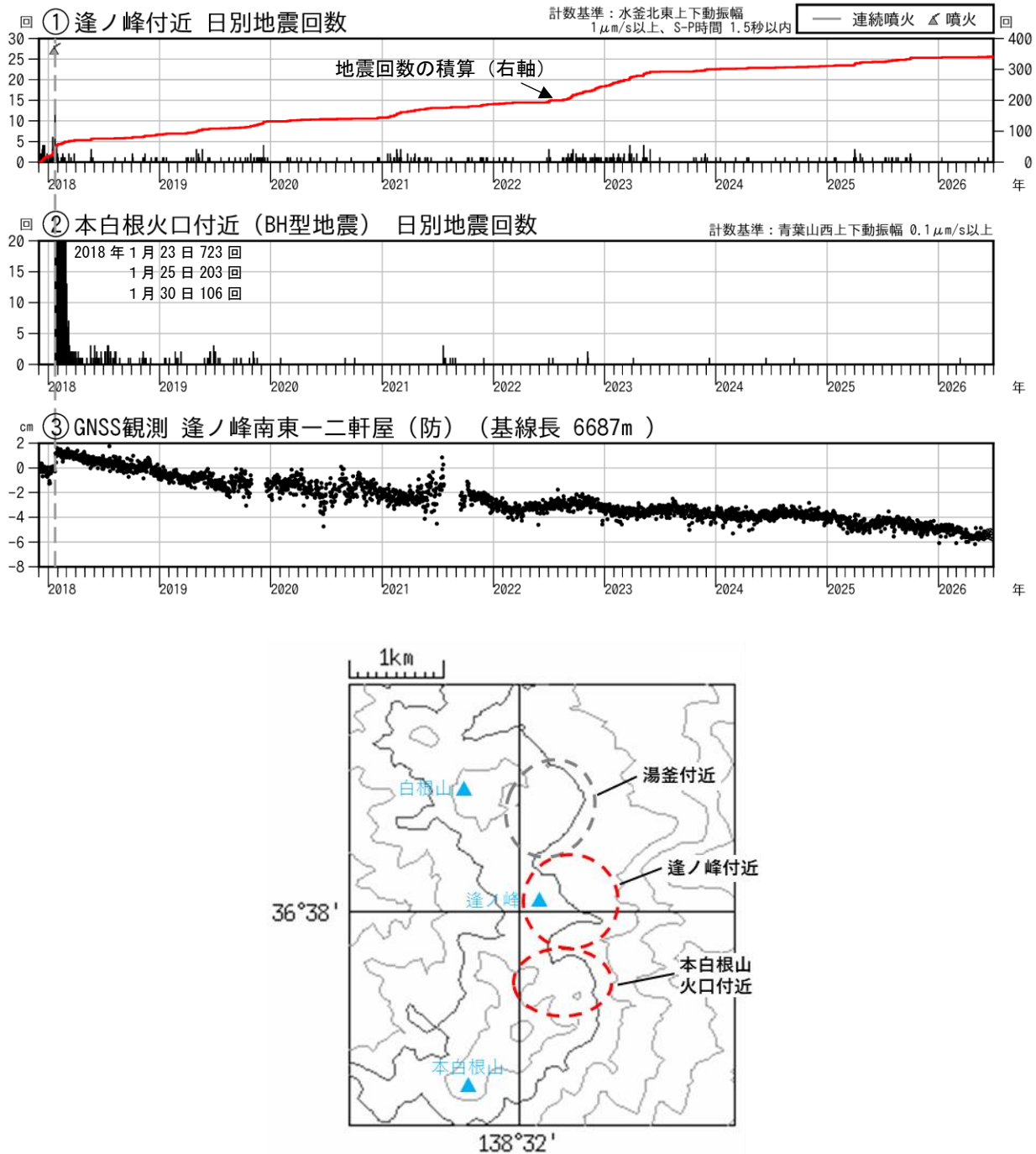
図13 草津白根山（本白根山） 火山活動経過図（2017年12月1日～2026年6月30日）
