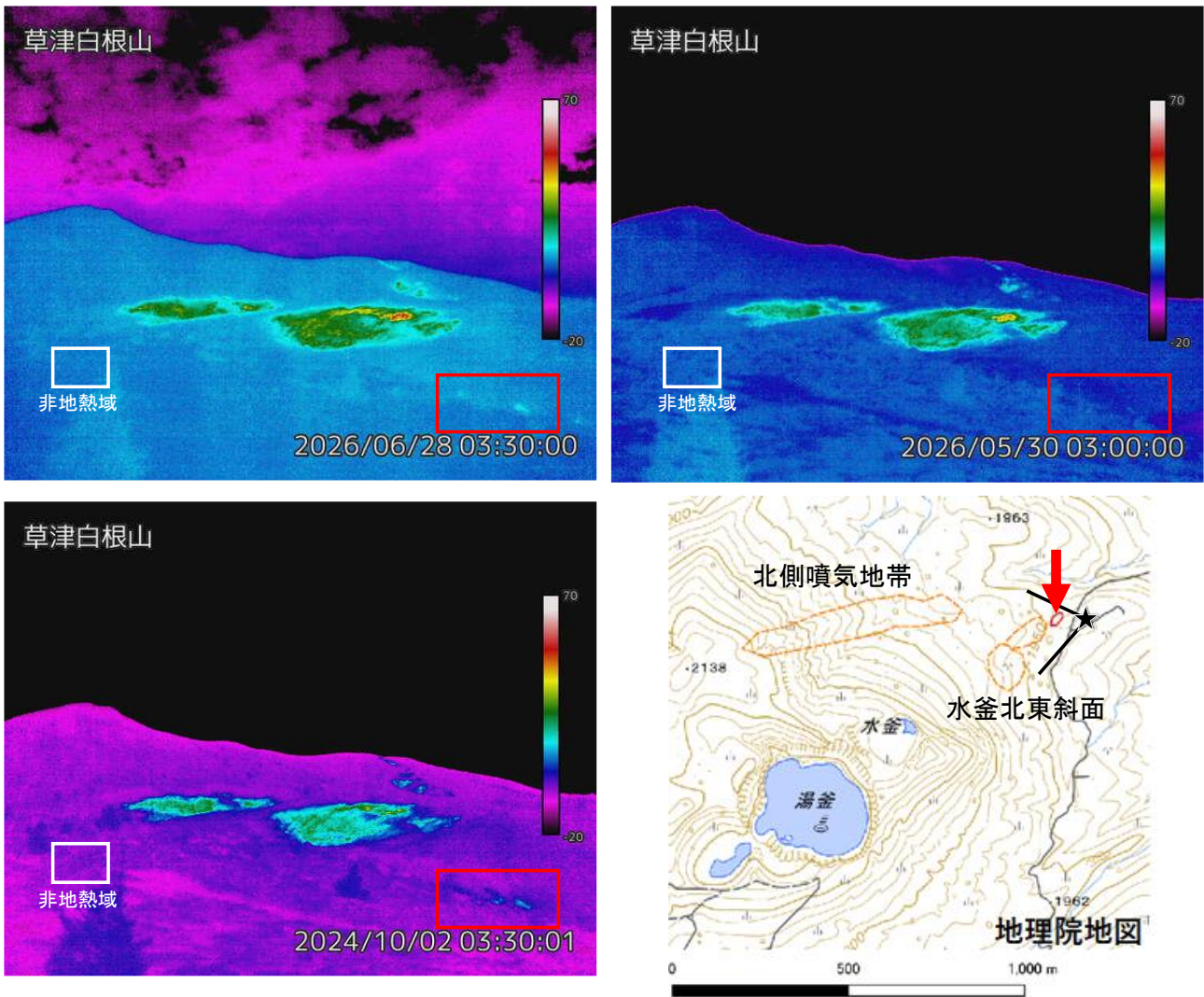
左上、右上及び左下の図はそれぞれ6月28日、5月30日及び2024年10月2日の夜間における地熱域の分布です。赤枠は、温度上昇が認められる領域に対応し、白枠は非地熱域（地熱域との比較のため設定）を示します。右下の地図の橙色で囲まれた領域は湯釜北側噴気地帯及び水釜北東の地熱域に対応し、矢印で示す赤枠は、温度上昇が認められる領域に対応します。星印は水釜北東2監視カメラの位置を示します。
