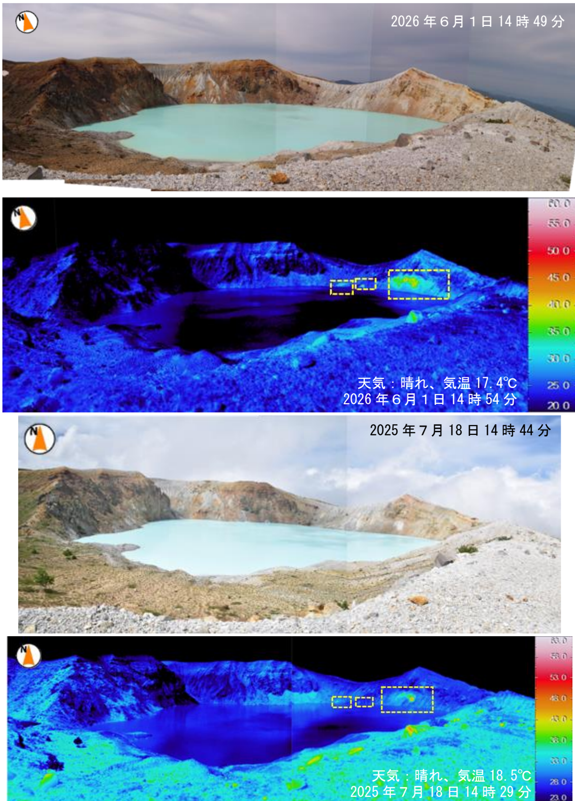
図1-4 草津白根山（白根山（湯釜付近））湯釜火口内の状況
