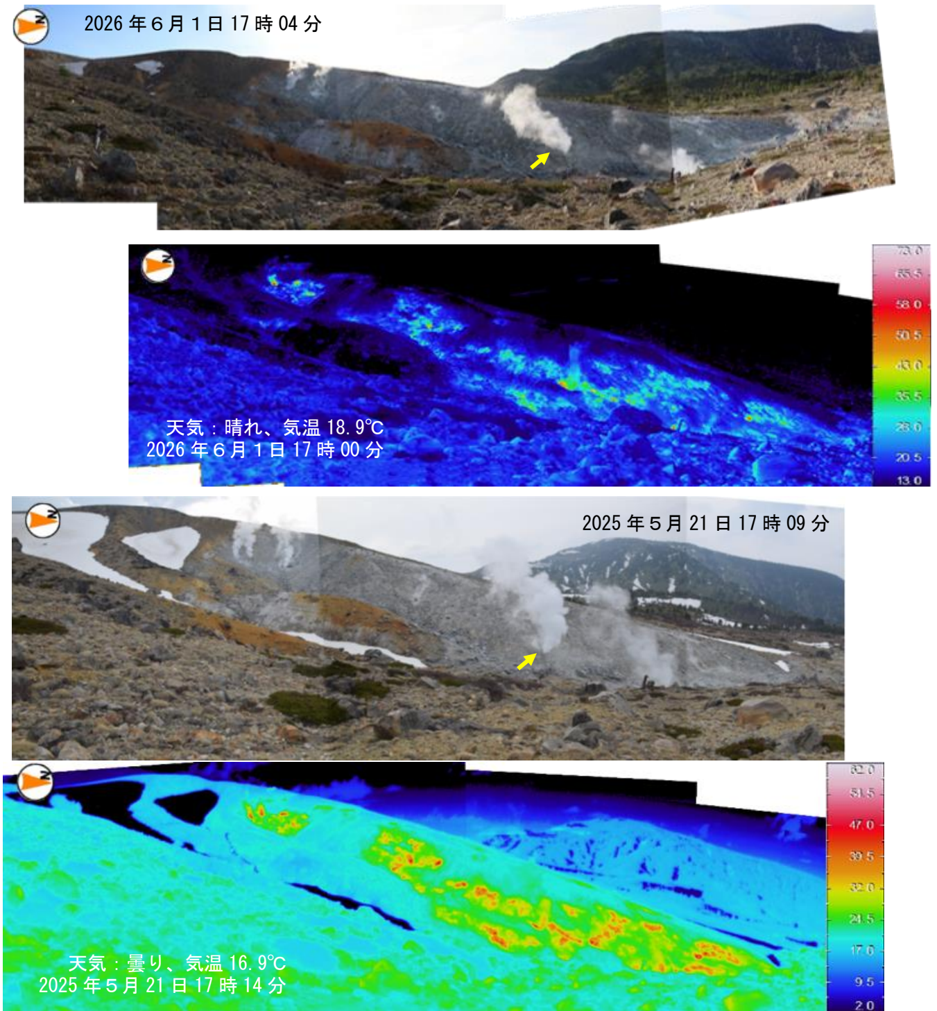
図1-6 草津白根山（白根山（湯釜付近））北側噴気地帯の状況
