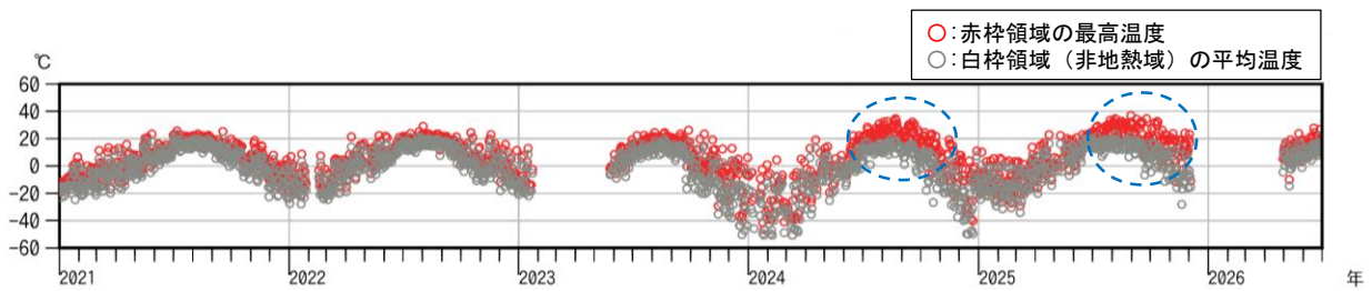
図1-8 草津白根山（白根山（湯釜付近）） 水釜北東の地熱域の状況 (2021年1月1日～2026年6月30日) ・水釜北東斜面の一部（上図の赤枠領域）で、2024年7月頃からみられていた周辺の非地熱域と比較して温度の高い箇所は、12月頃から次第に不明瞭となっていました。2025年7月以降、再び温度の高まりが認められていましたが、現在は不明瞭となっています（下図の青色破線内）。 ・その他の領域では、目立った変化は認められていません。
