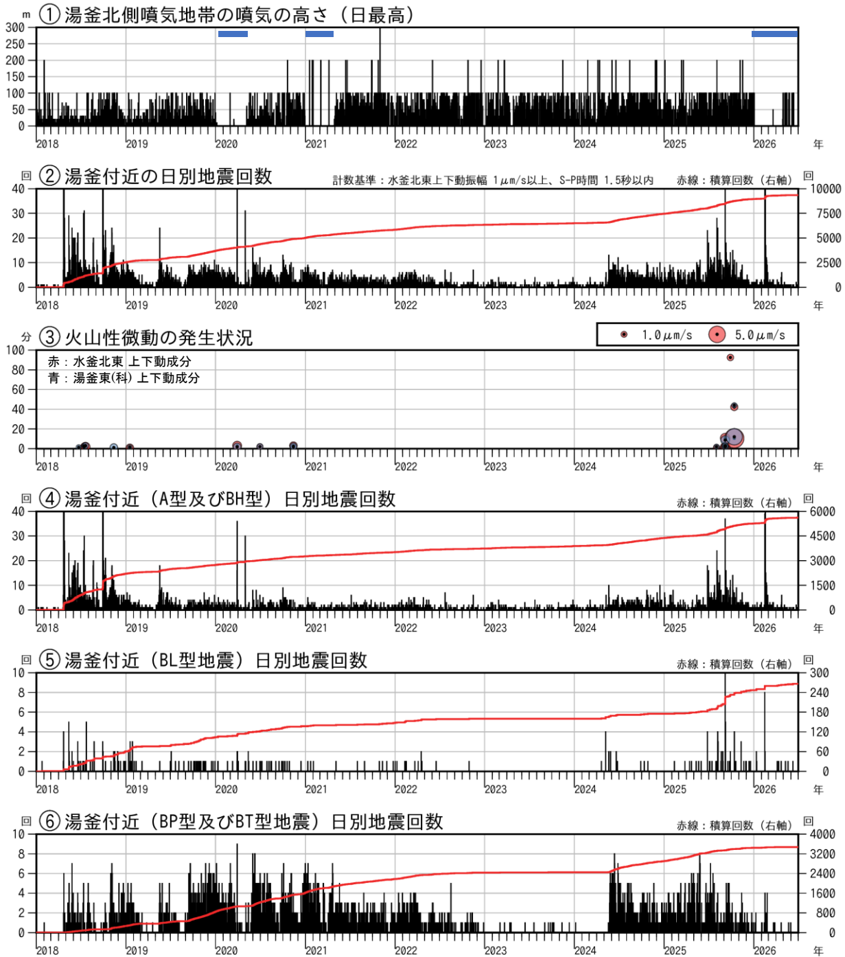
図3 草津白根山（白根山（湯釜付近）） 火山活動経過図（2018年1月1日～2026年6月30日） 上図①の青線で示す期間については、一部の観測機器で障害が発生したため、100m未満の噴気については観測できていない場合があります。 赤線は地震回数の積算を示しています。火山性地震の種類については図11を参照してください。
