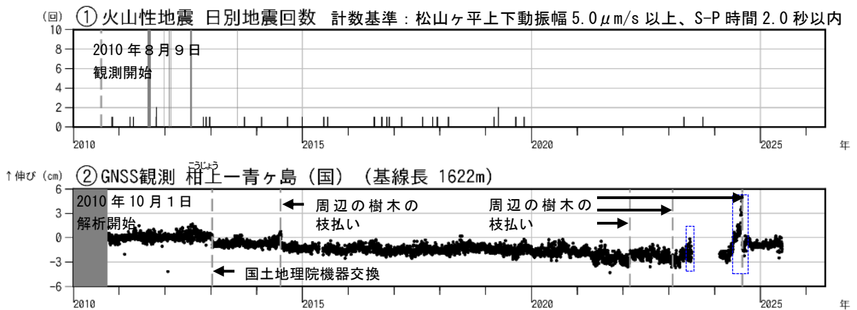
図3 青ヶ島 火山活動経過図（2010年8月9日～2026年5月31日） ① グラフの灰色部分は機器障害による欠測を示す。 ② （国）：国土地理院、図5のGNSS基線②に対応。グラフの空白部分は柑上の障害による欠測を示す。青破線内の期間に見られる変化は、柑上観測点周囲の樹木によるものです。
