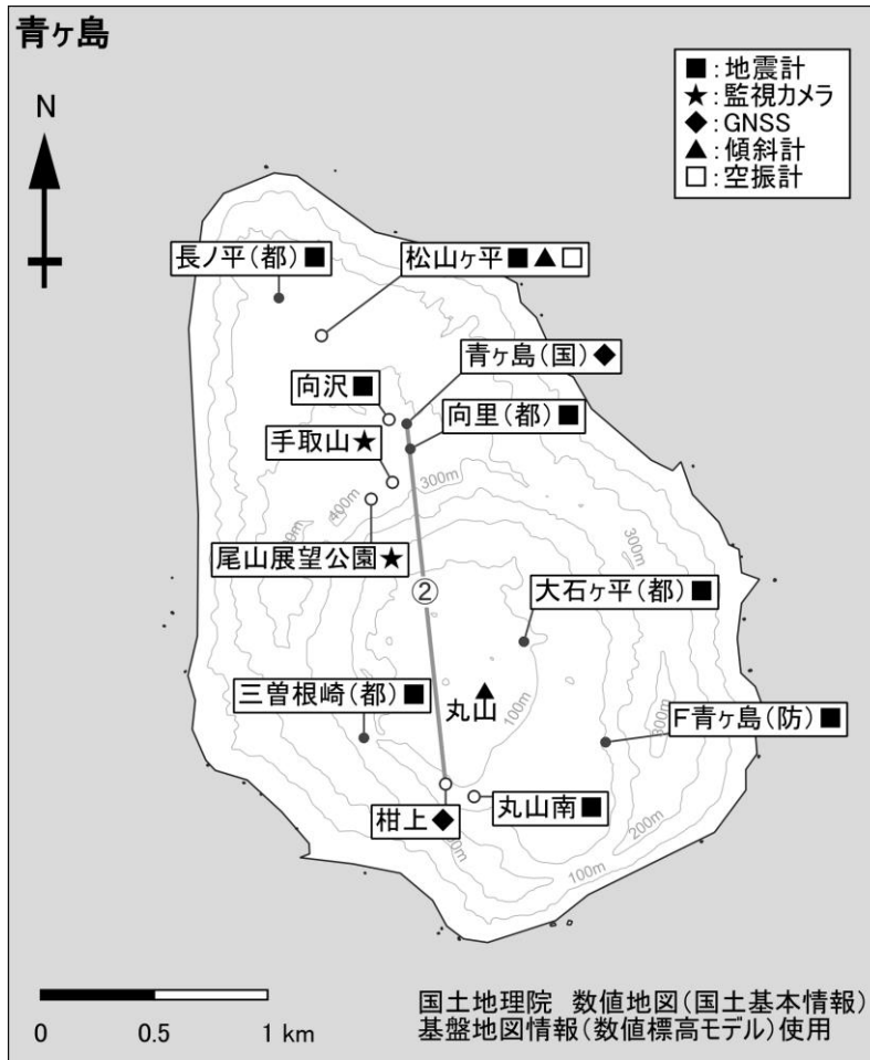
図5 青ヶ島 観測点配置図 GNSS 基線は図3の②に対応しています。
