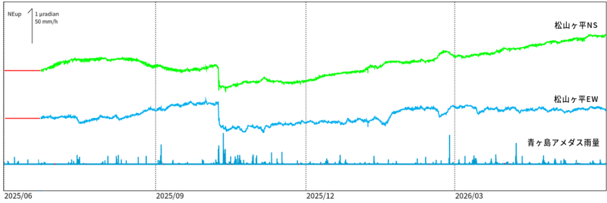
図4 青ヶ島 松山ヶ平観測点における傾斜データ（2025年6月1日～2026年5月31日） グラフの赤線部分は欠測を示す。 ・傾斜計による観測では、火山活動によるとみられる変動は認められません。
