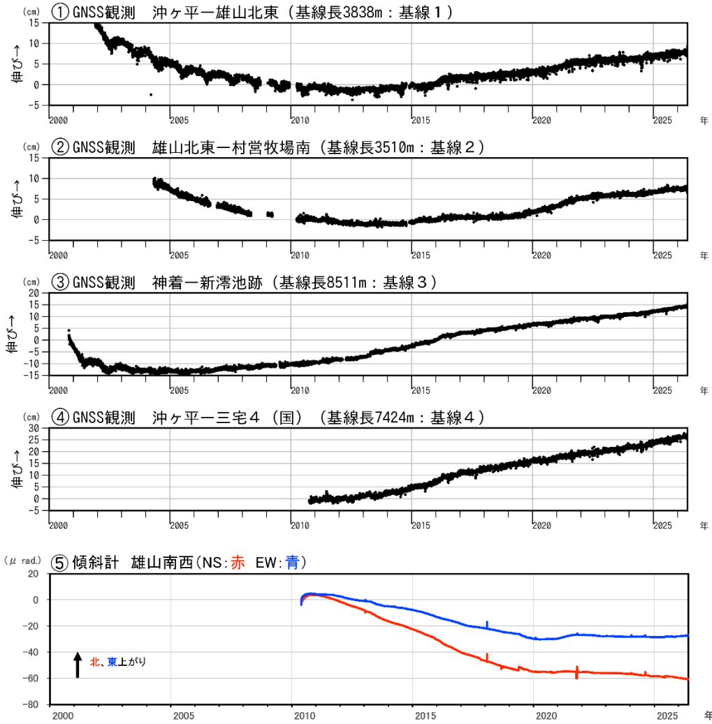
図6 三宅島 GNSS連続観測及び傾斜計観測結果 (2000年1月1日～2026年5月31日)
