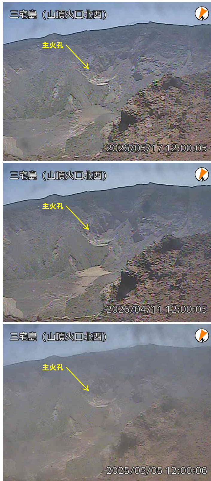
図3 三宅島 山頂火口内の状況（山頂火口北西監視カメラの可視画像）
