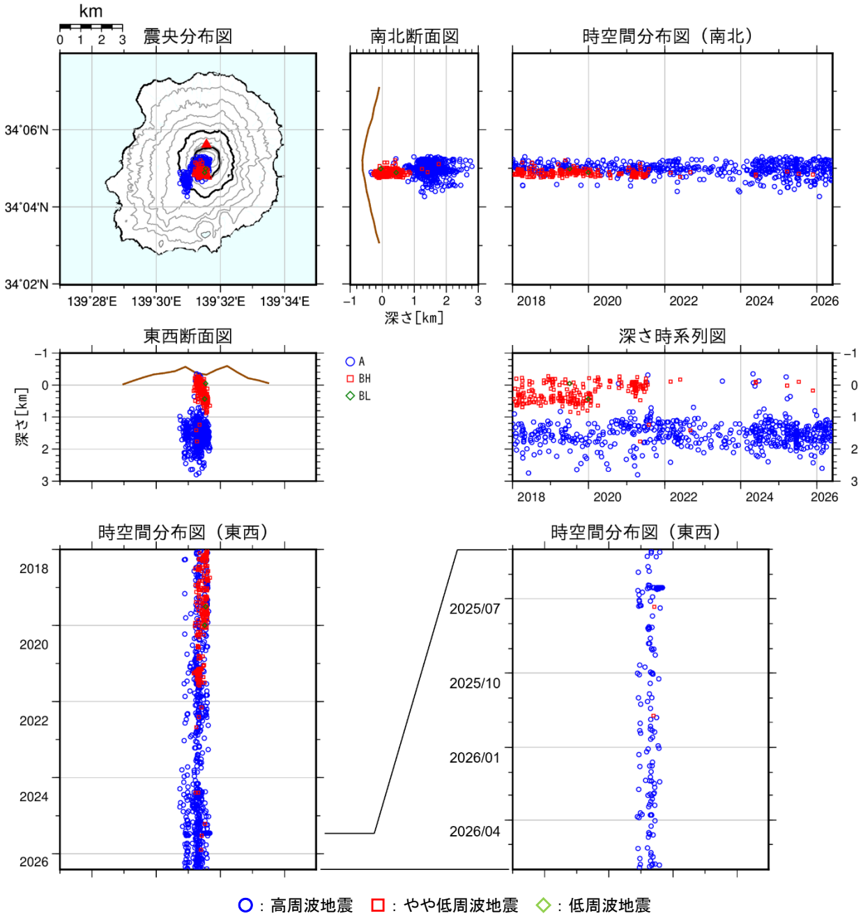
図7 三宅島 震源分布図（2018年1月1日～2026年5月31日）
