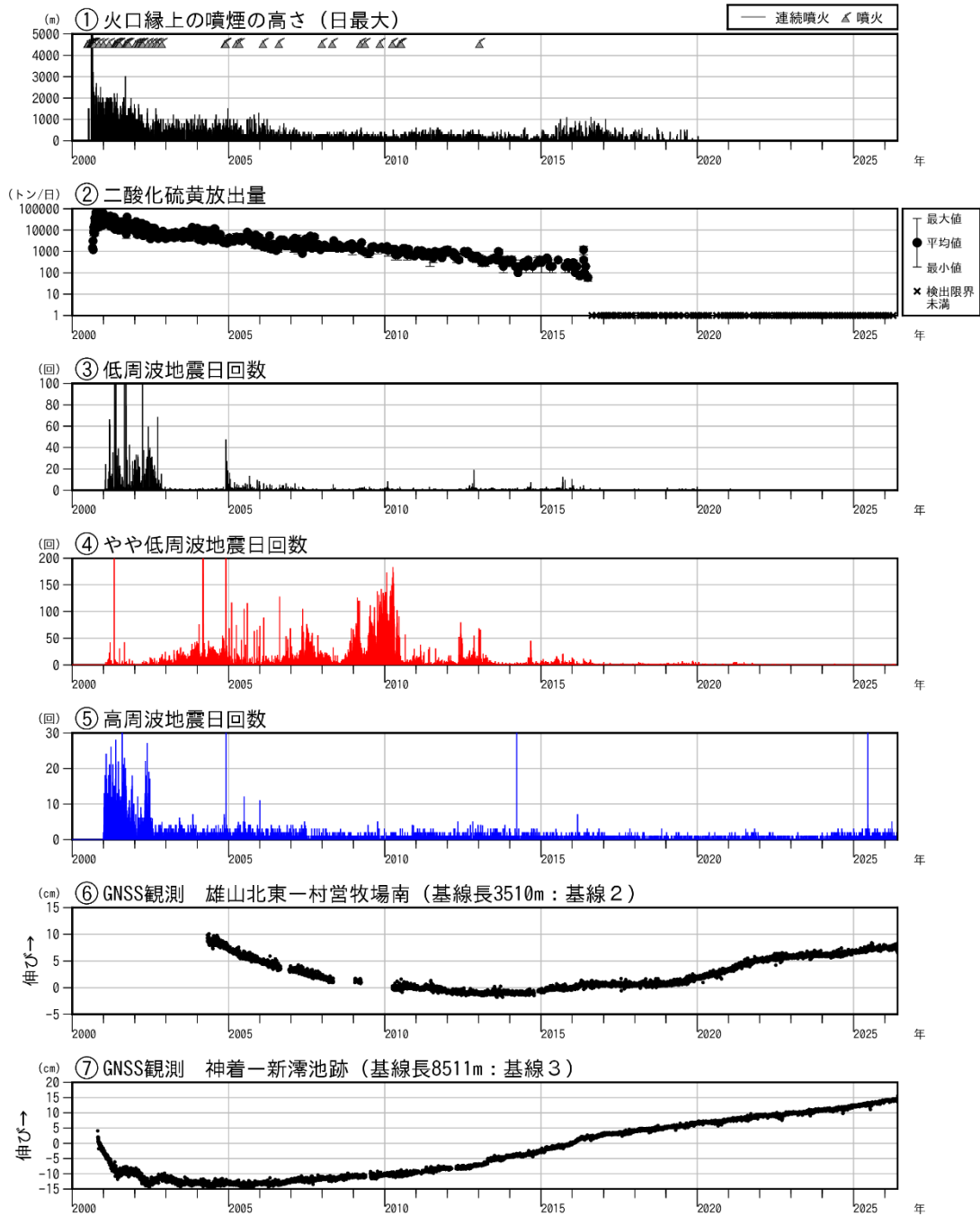
図5 三宅島 長期の火山活動経過図（2000年1月1日～2026年5月31日）
