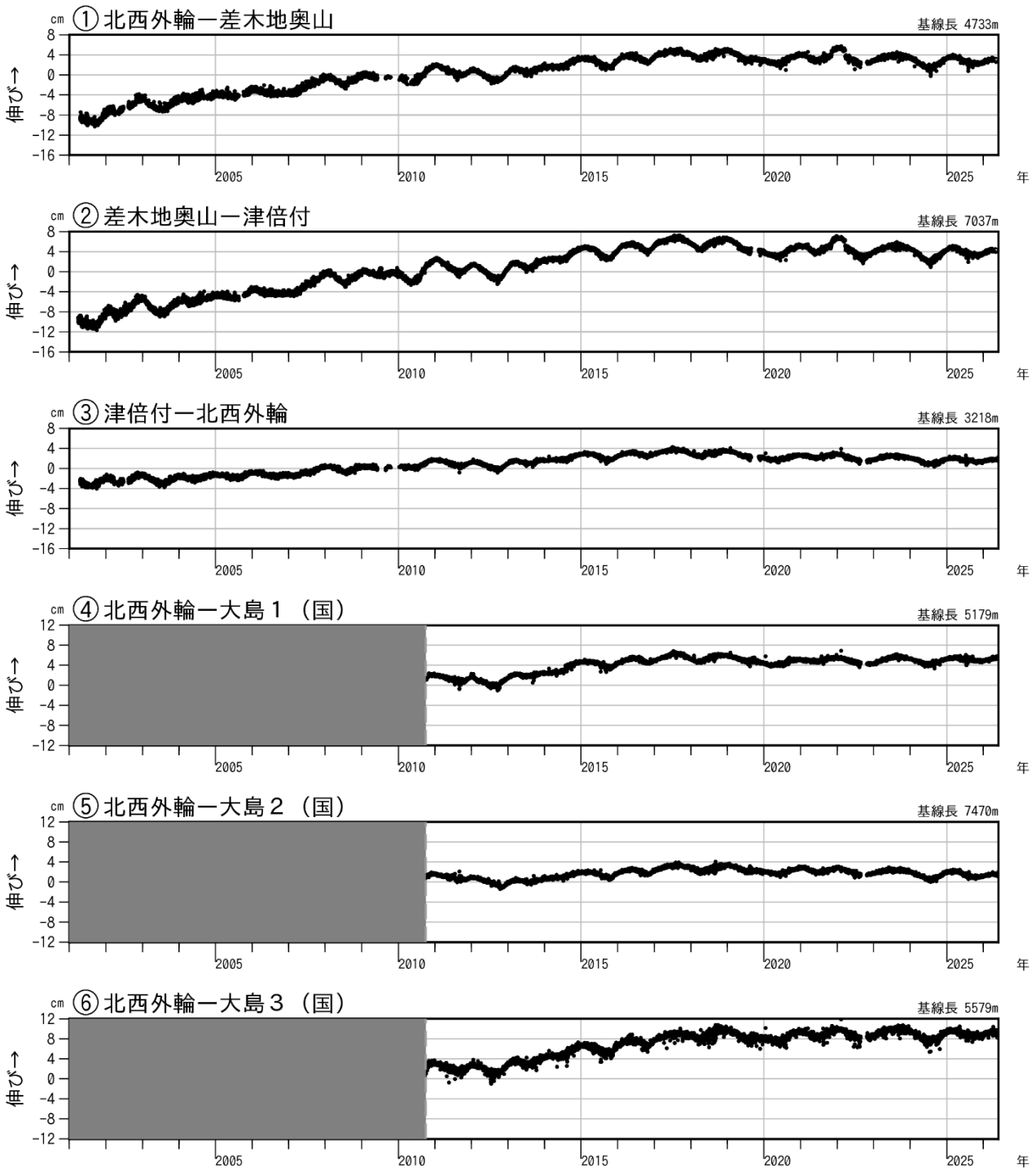
図3-1 伊豆大島 GNSS連続観測による基線長変化(2001年1月~2026年5月)
