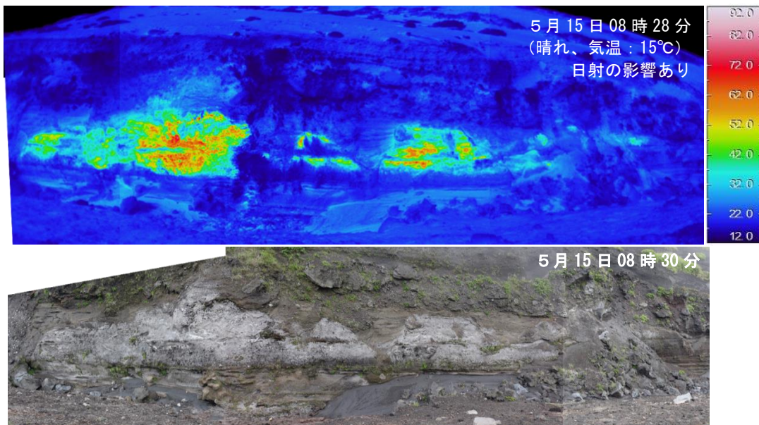
図7 伊豆大島 楯形山西谷の状況（撮影方向は図8参照）
