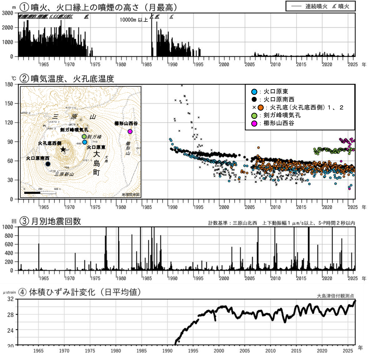
図1 伊豆大島 長期間の火山活動経過図（1961年1月～2026年5月）
