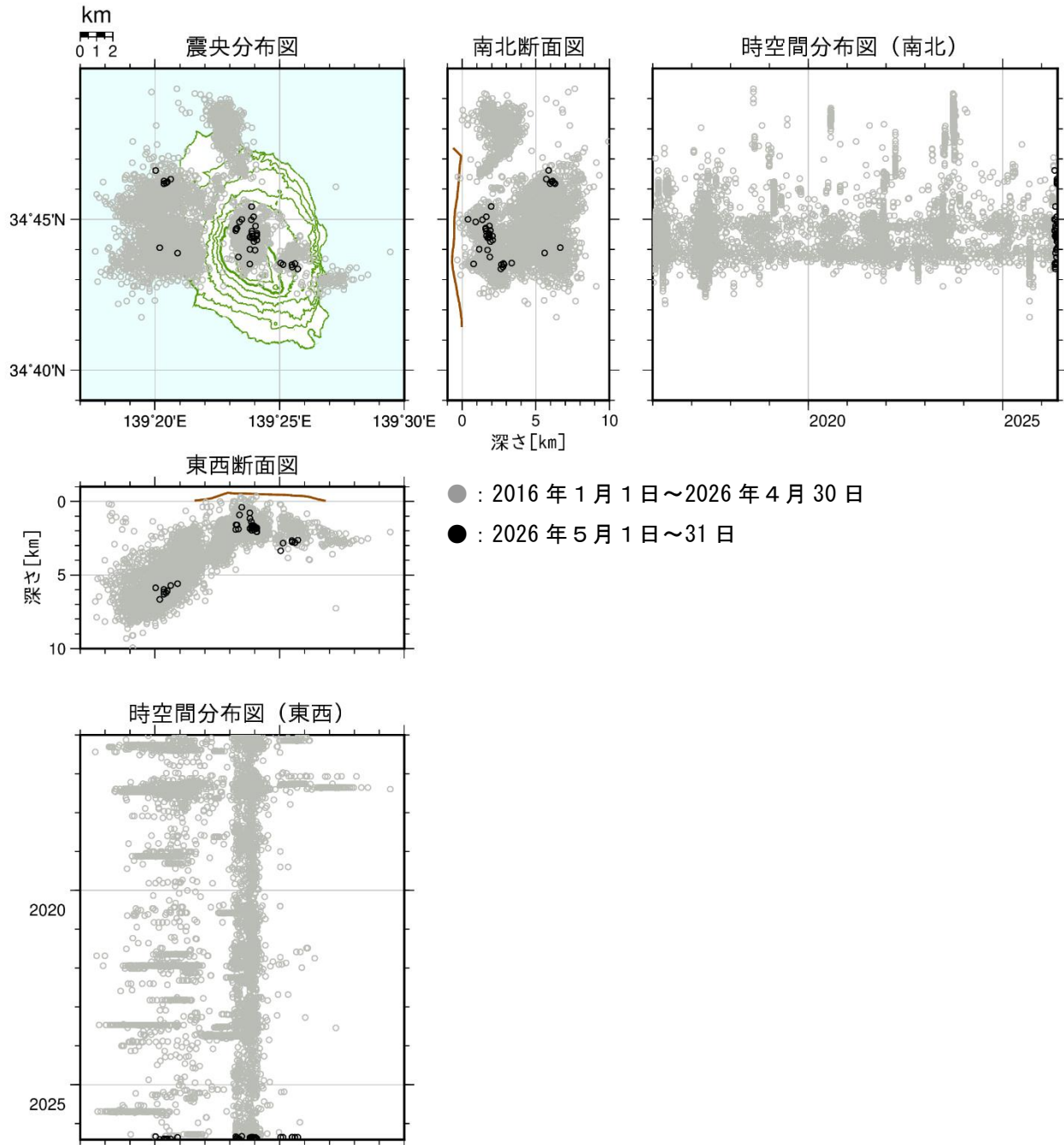
図4 伊豆大島 震源分布図（2016年1月1日～2026年5月31日）
