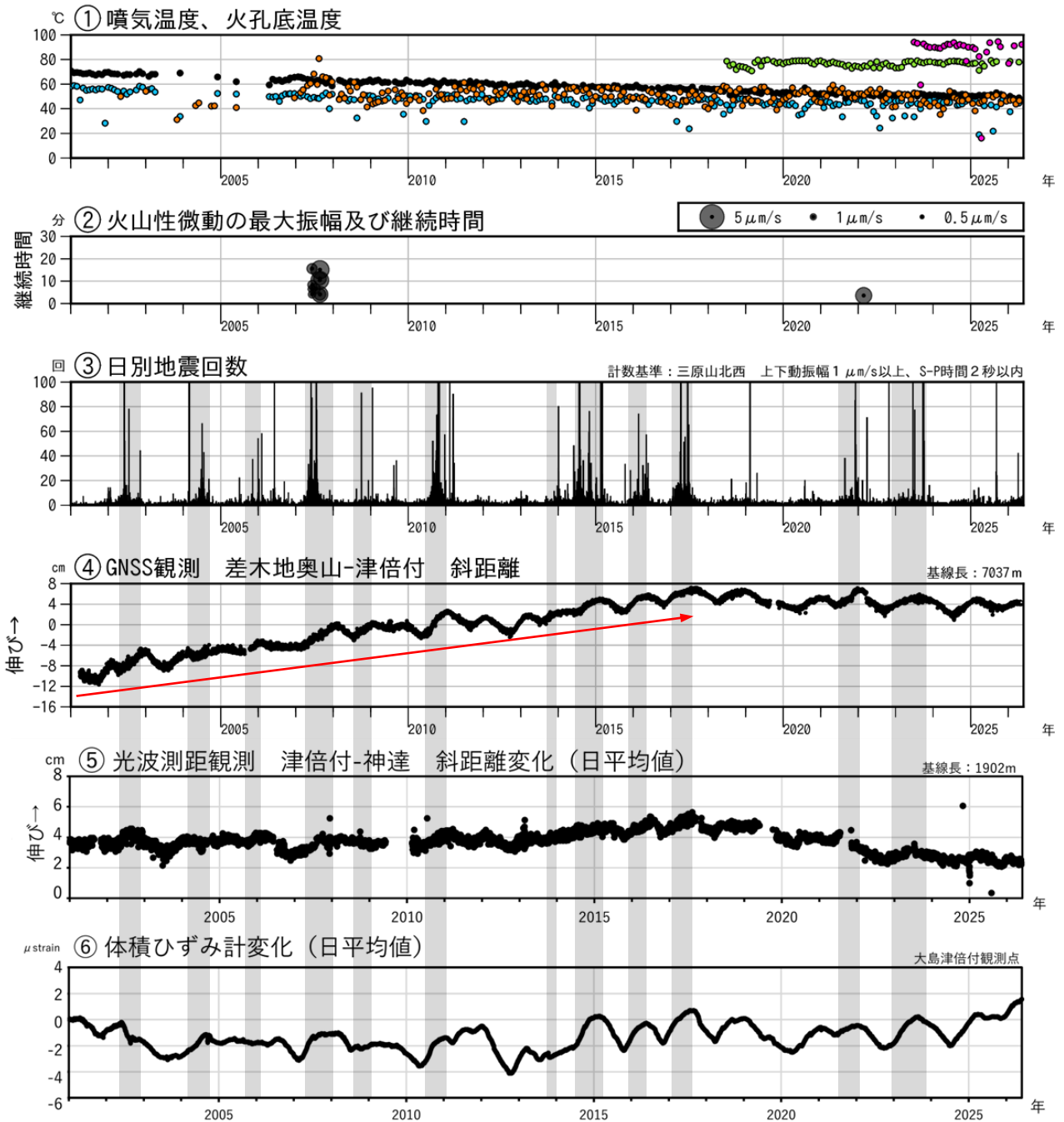
図2 伊豆大島 最近の火山活動経過図（2001年1月～2026年5月）
