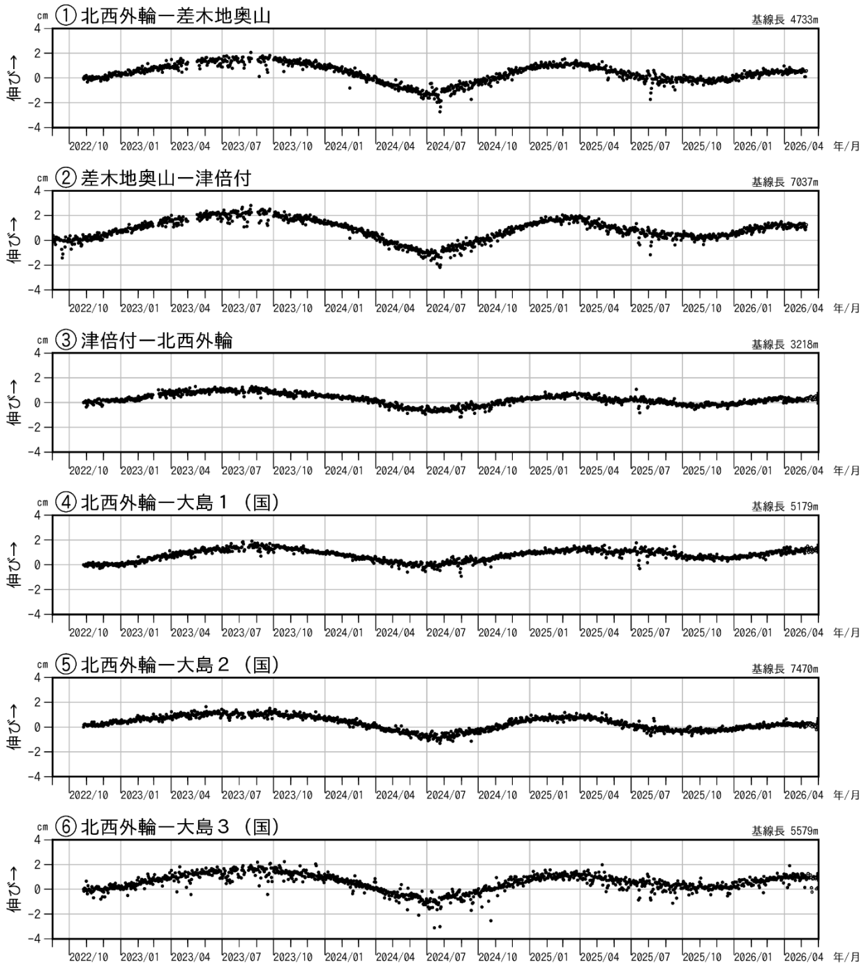
図3-2 伊豆大島 GNSS連続観測による基線長変化(2022年9月~2026年5月)
