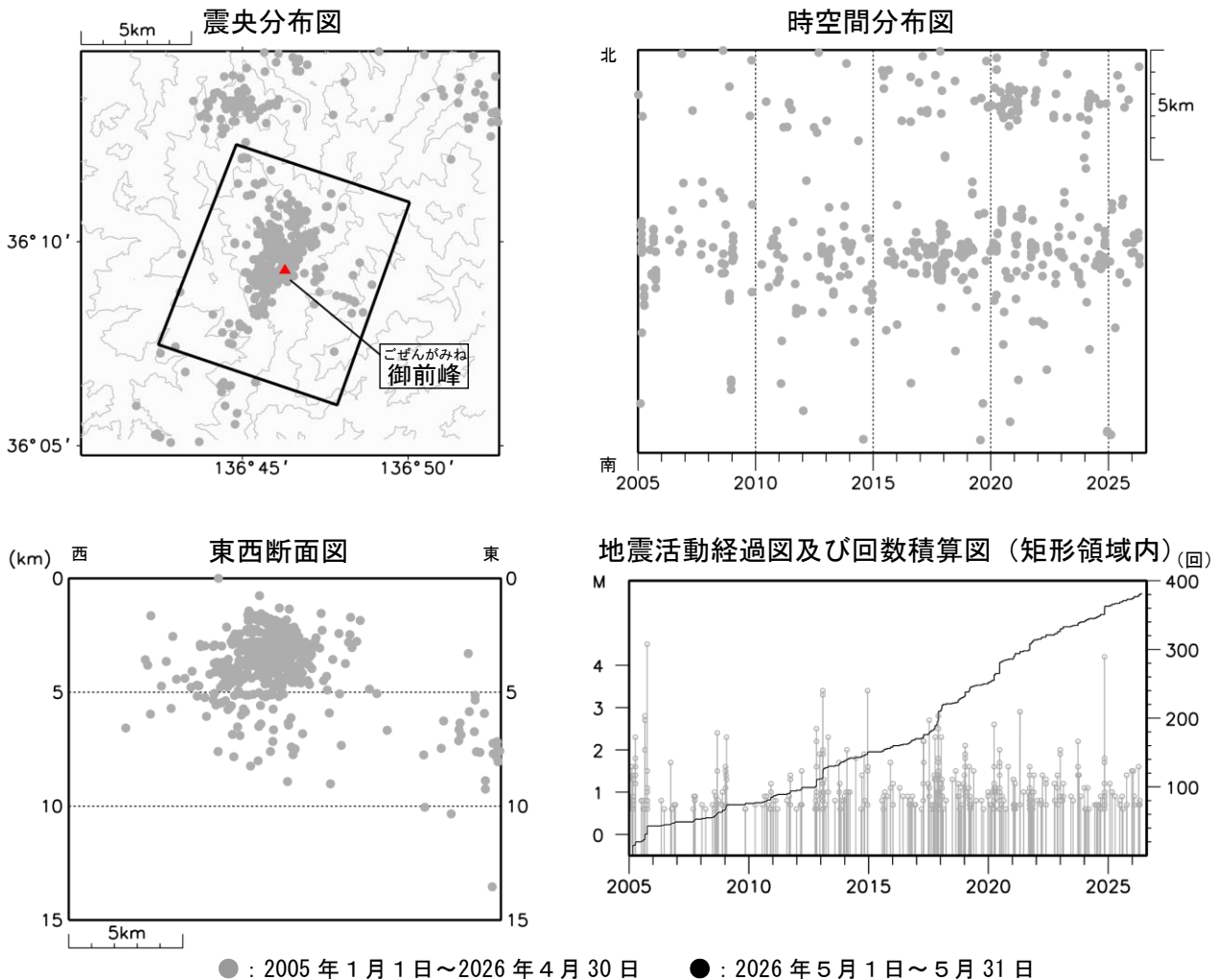
図4 白山 広域地震観測網による山体・周辺の地震活動（2005年1月1日～2026年5月31日） 広域地震観測網により震源決定したもので、深さは全て海面以下として決定しています。なお、2020年9月以降については、地震観測点の標高を考慮する等、震源決定の手法を変更しています。 M（マグニチュード）は地震の規模を表します。M0.6以上の地震を表示しています。 図中の震源要素は一部暫定値を含んでおり、後日変更することがあります。 ・今期間、白山付近の地震活動は低調に経過しました。
