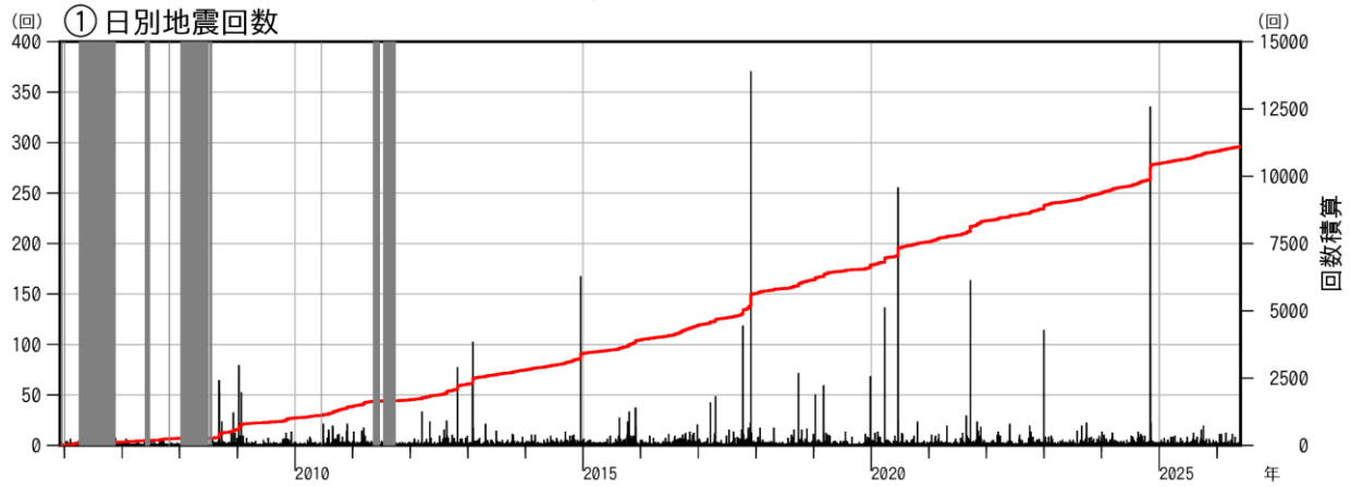
図3 白山 日別地震回数と積算回数（2005年12月1日～2026年5月31日） 図の灰色部分は機器障害による欠測期間。
