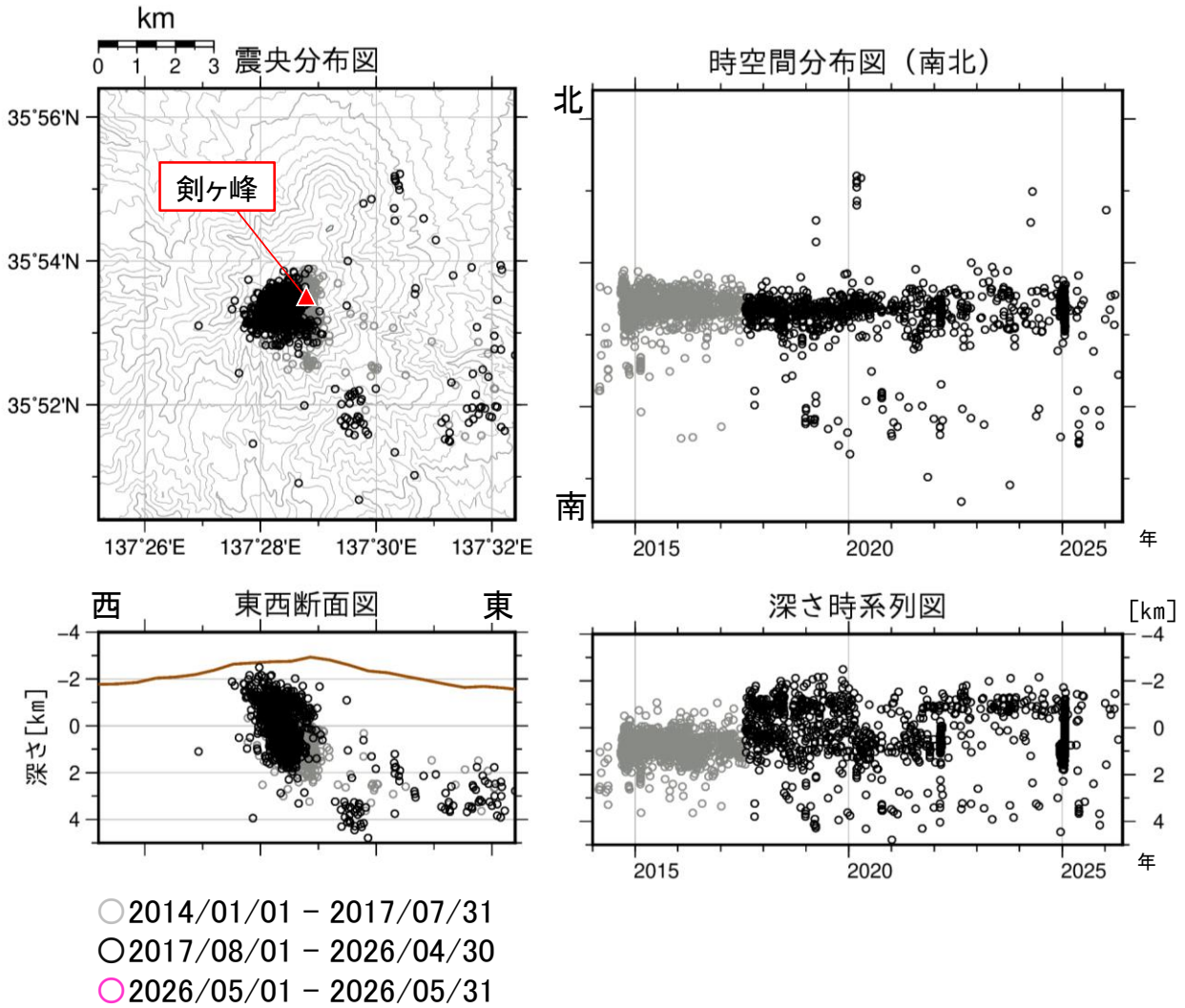
図4 御嶽山 震源分布図（2014年1月1日～2026年5月31日） 2017年8月1日以降の震源分布は、震源計算に使用する観測点を新たに追加して再計算したものを示しています。 観測点の稼働状況により、求まる震源の数の減少や位置の精度低下が生じる場合があります。
