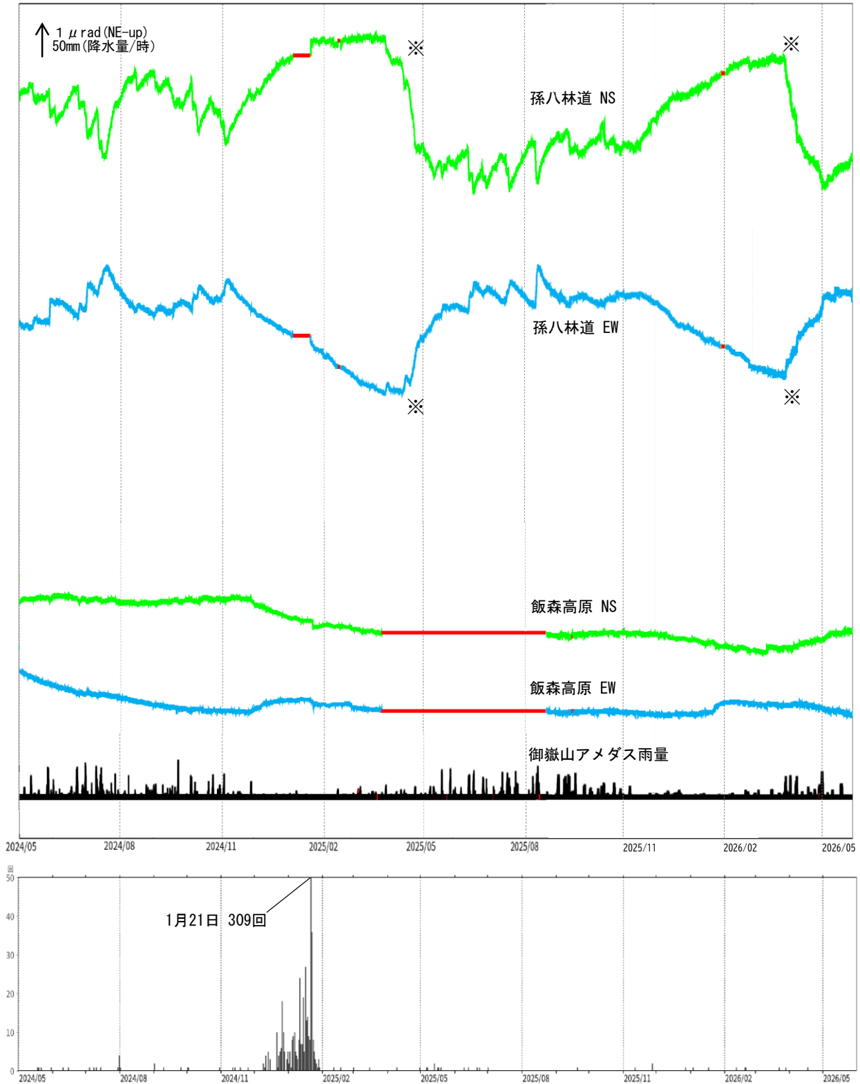
図7 御嶽山 傾斜変動と日別地震回数推移（2024年5月1日～2026年5月31日） データは時間平均値で、潮汐補正済みです。 赤線部分は欠測を示します。 ※：季節的な変動とみられます。
