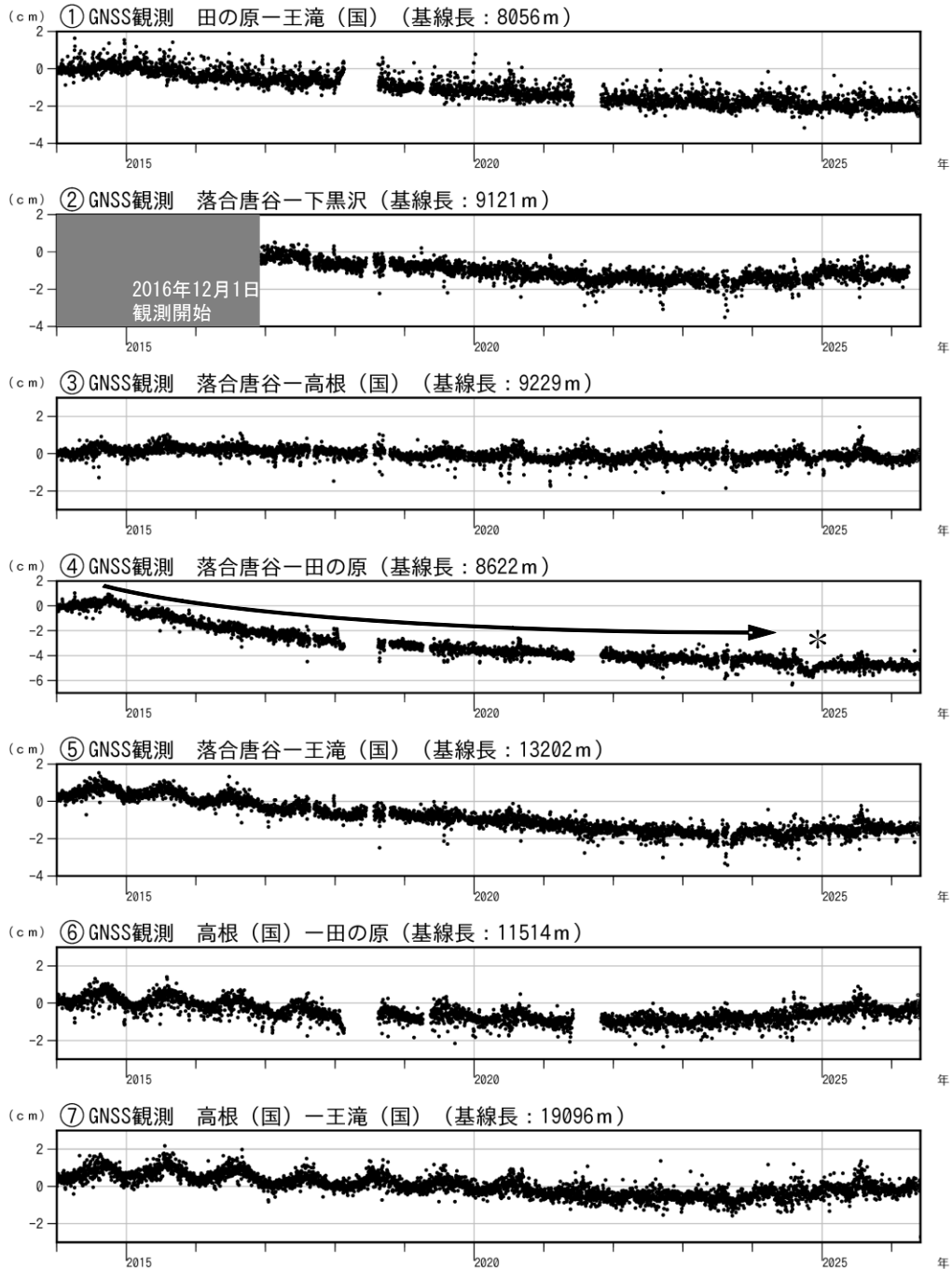
図5 御嶽山 GNSS連続観測結果（2014年1月1日～2026年5月31日）
