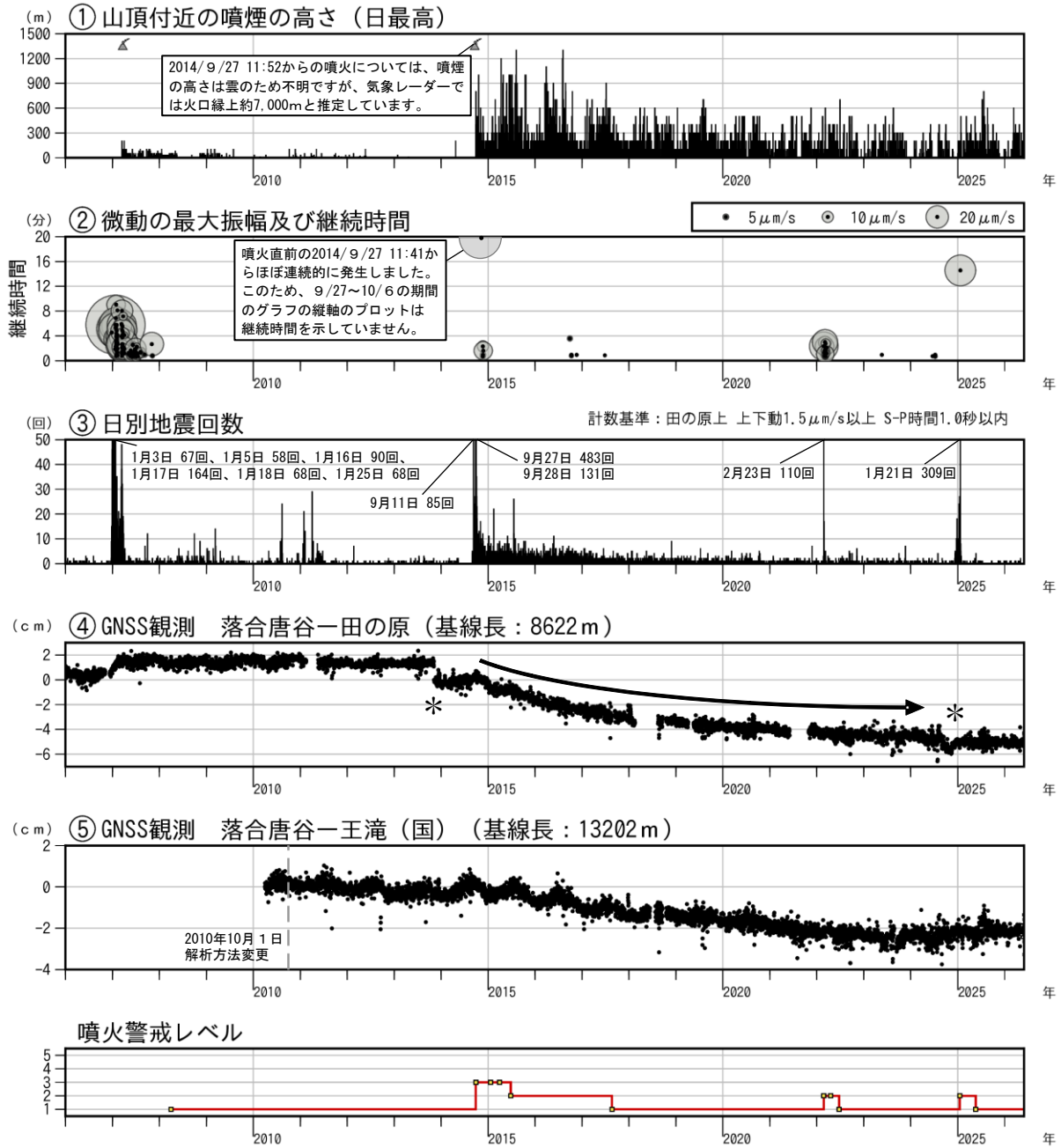
図1 御嶽山 長期間の火山活動経過図（2006年1月1日～2026年5月31日）
