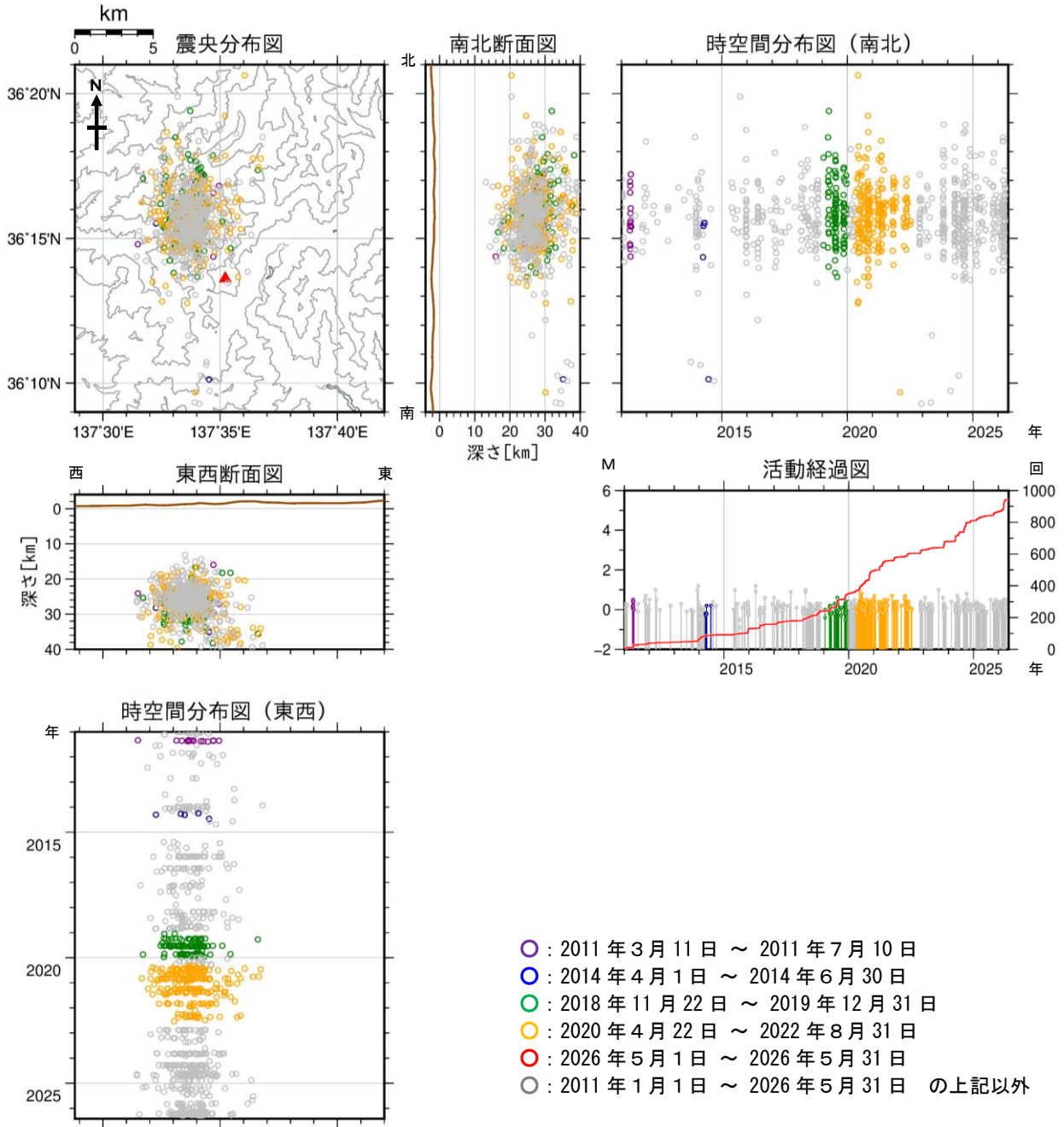
図10 焼岳 広域地震観測網による深部低周波地震の震源分布図（2011年1月1日～2026年5月31日） 広域地震観測網により震源決定したもので、深さは全て海面以下として決定しています。なお、2020年9月以降については、地震観測点の標高を考慮する等、震源決定の手法を変更しています。
