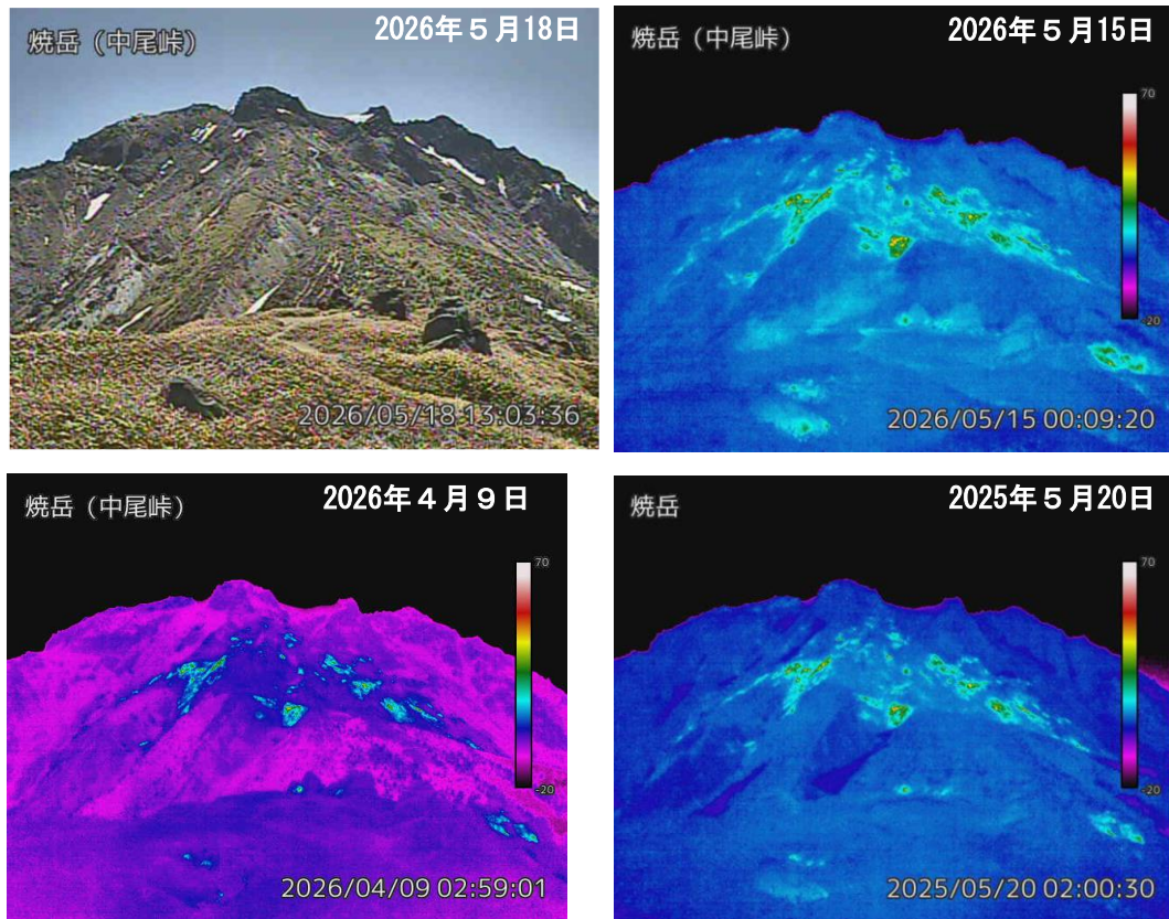
図4 焼岳 中尾峠赤外熱映像カメラによる焼岳の北側斜面の地表面温度分布と可視画像 撮影場所と撮影方向は図11を参照。 ・前月（左下図）及び前年同月（右下図）と比較して、噴気の状態や地表面温度分布に特段の変化はありません。
