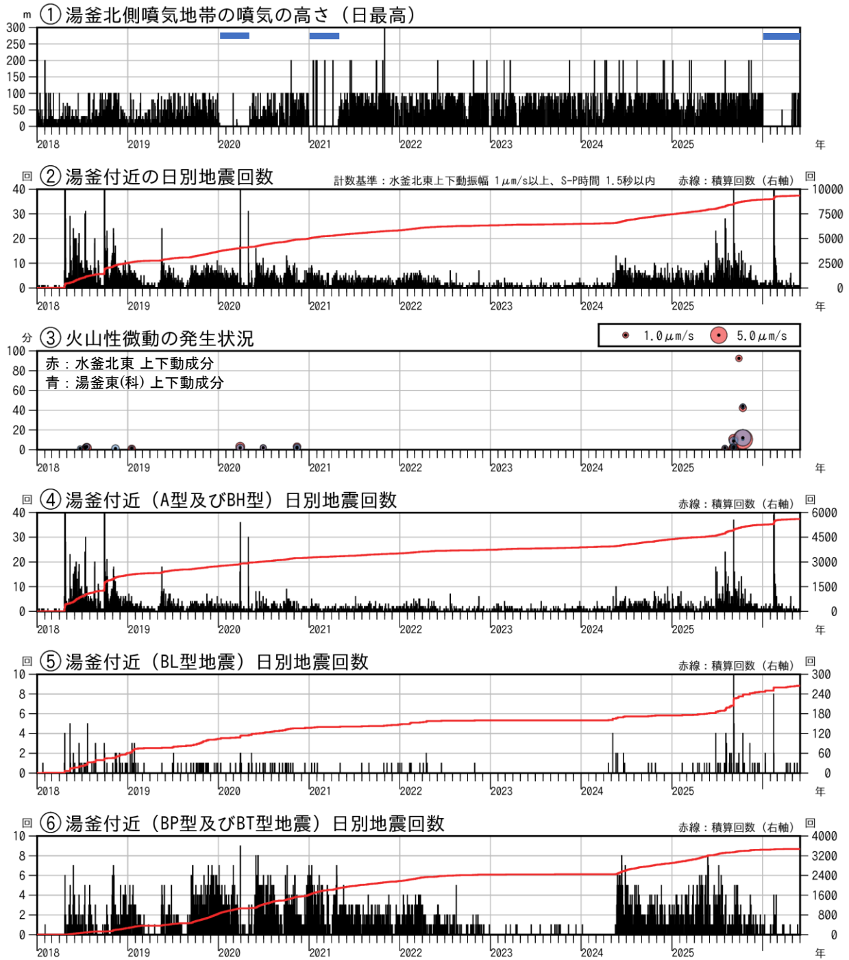
図3 草津白根山（白根山（湯釜付近）） 火山活動経過図（2018年1月1日～2026年5月31日） 上図①の青線で示す期間については、一部の観測機器で障害が発生したため、100m未満の噴気については観測できていない場合があります。 赤線は地震回数の積算を示しています。火山性地震の種類については図11を参照してください。
