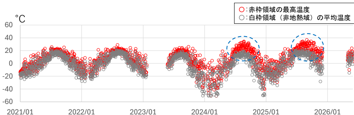
図1-2 草津白根山（白根山（湯釜付近）） 水釜北東の地熱域の状況
