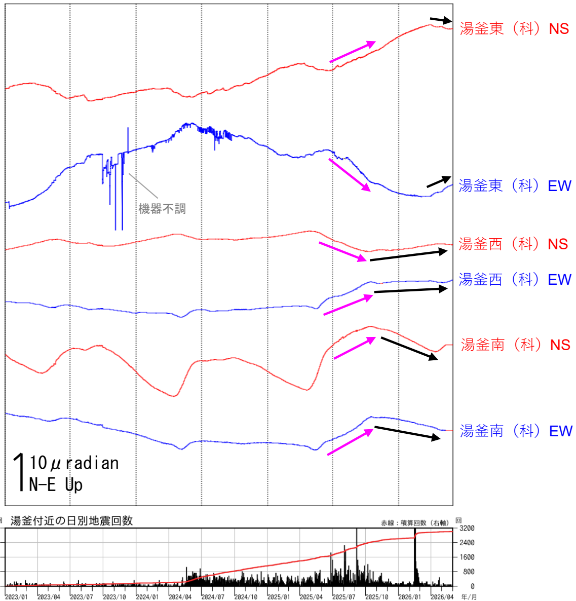
図5 草津白根山（白根山（湯釜付近）） 傾斜変動（2023年1月1日～2026年5月31日） データは時間平均値を使用しています。（科）：東京科学大学
