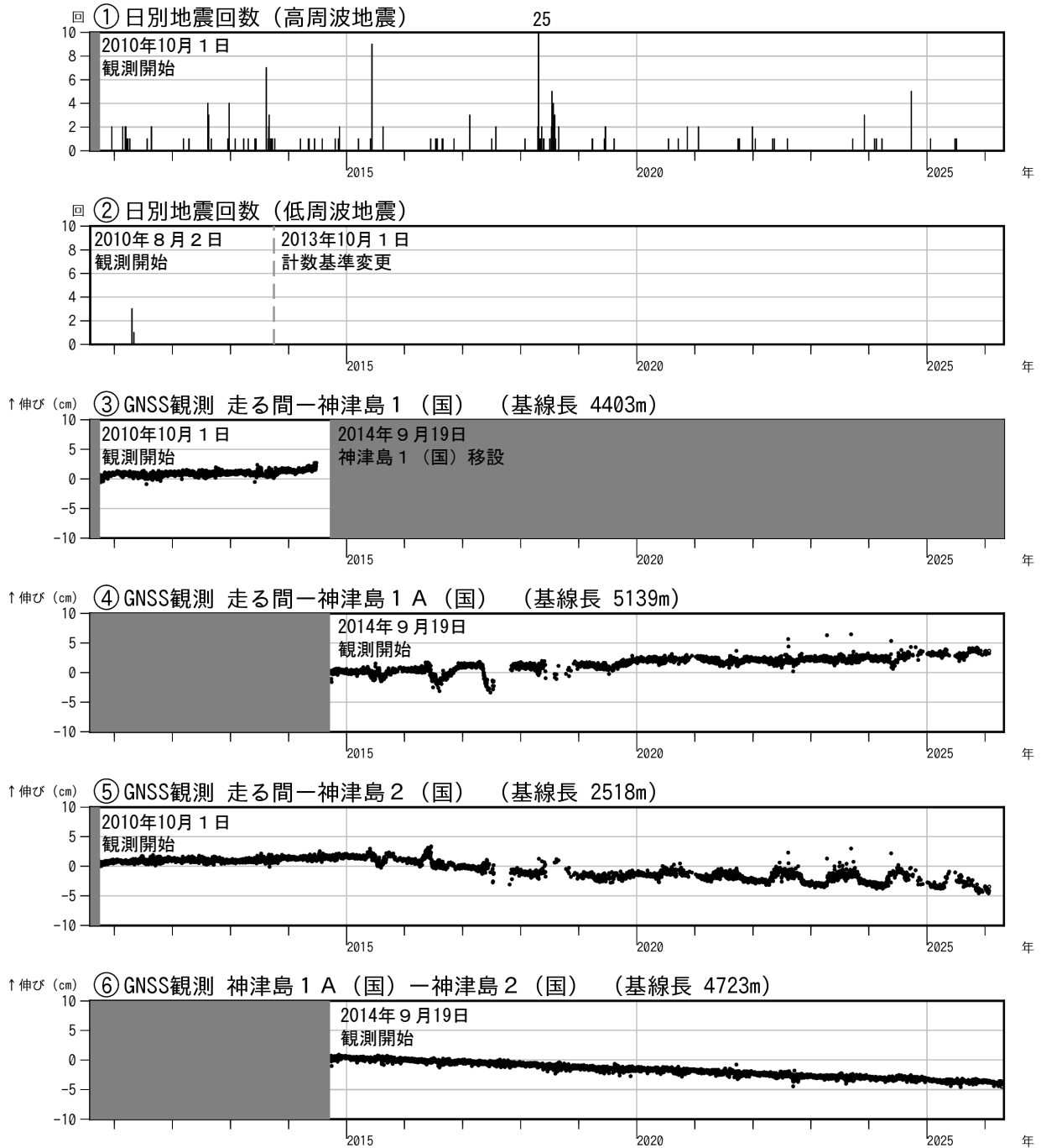
図2 神津島 火山活動経過図(2010年8月2日～2026年4月30日)
