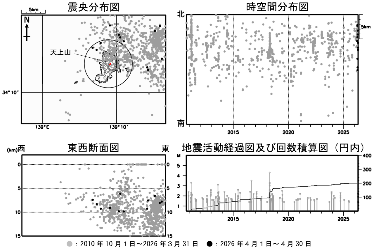
図3 神津島 広域地震観測網による山体・周辺の地震活動（2010年10月1日～2026年4月30日） 広域地震観測網により震源決定したもので、深さは全て海面以下として決定しています。なお、2020年9月以降については、地震観測点の標高を考慮する等、震源決定の手法を変更しています。 M（マグニチュード）は地震の規模を表し、M1.4以上の地震を示しています。 図中の震源要素は一部暫定値が含まれており、後日変更することがあります。 計数対象（天上山西から半径約5km、深さ約15km以内）以外の地震が含まれるため、図2-①の日別地震回数（高周波地震）とは異なります。 震央分布図中の円は火山性地震の回数の計数対象（天上山西から半径5km、深さ15km以内）の範囲を示しています。 ・地震活動は低調に経過しました。
