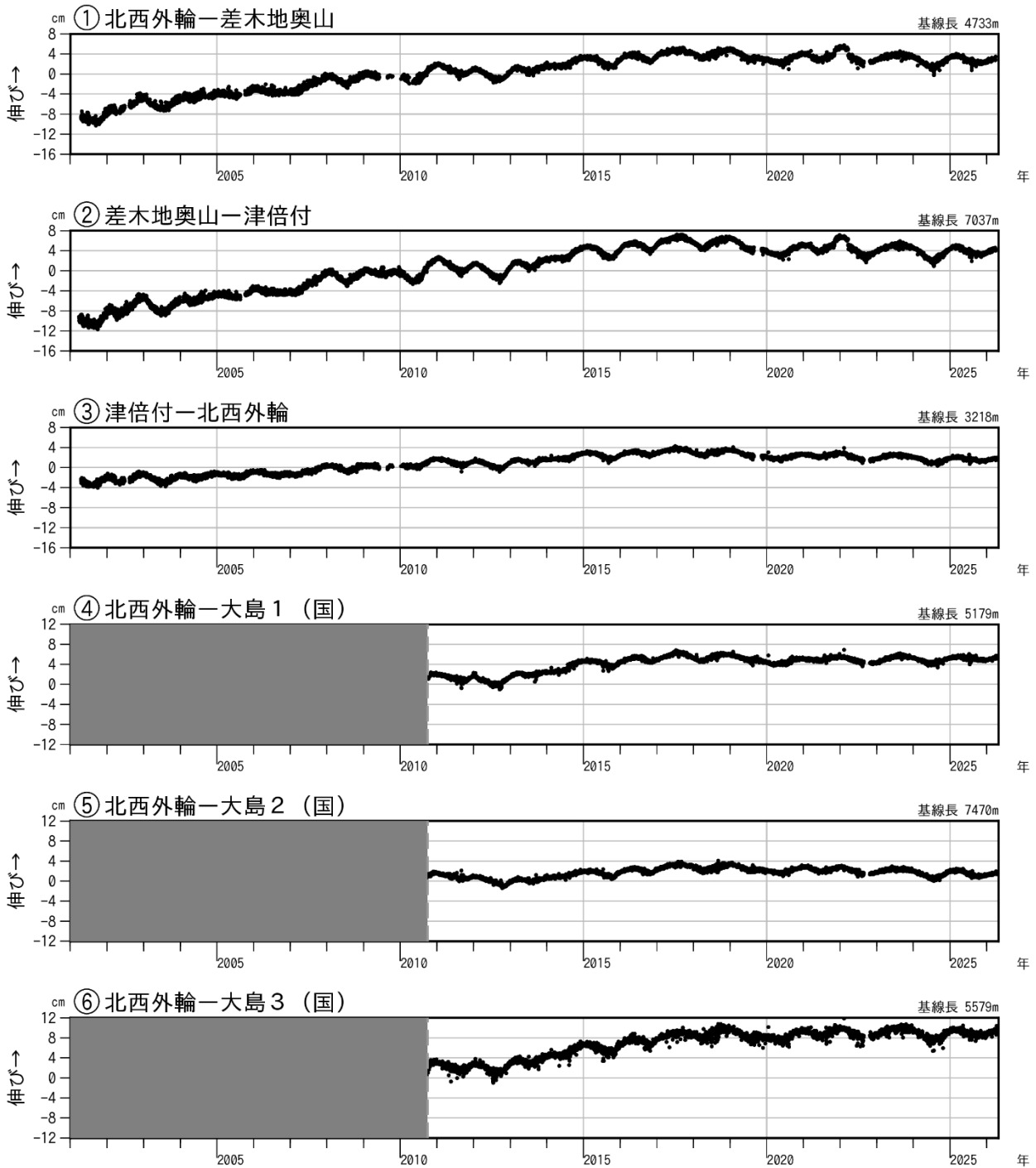
図3-1 伊豆大島 GNSS連続観測による基線長変化(2001年1月~2026年4月)
