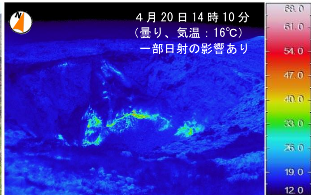
図6-1 伊豆大島 中央火口内の状況（撮影方向は図8参照）
