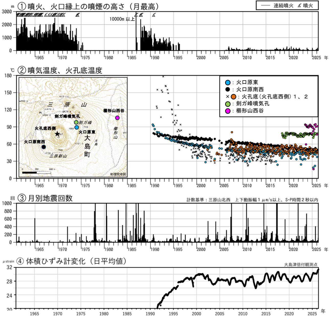
図1 伊豆大島 長期間の火山活動経過図（1961年1月～2026年4月）
