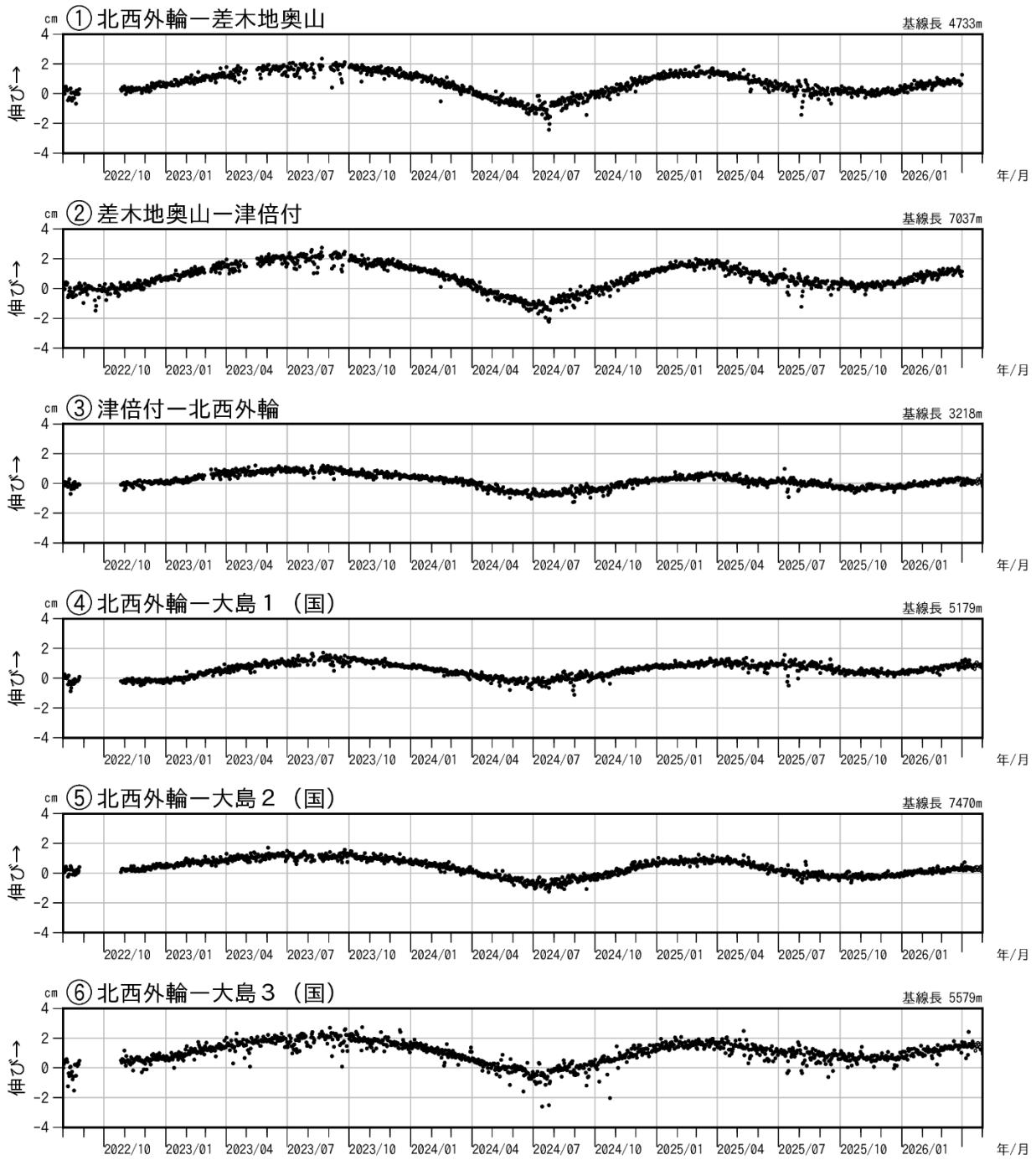
図3-2 伊豆大島 GNSS 連続観測による基線長変化(2022年8月~2026年4月)
