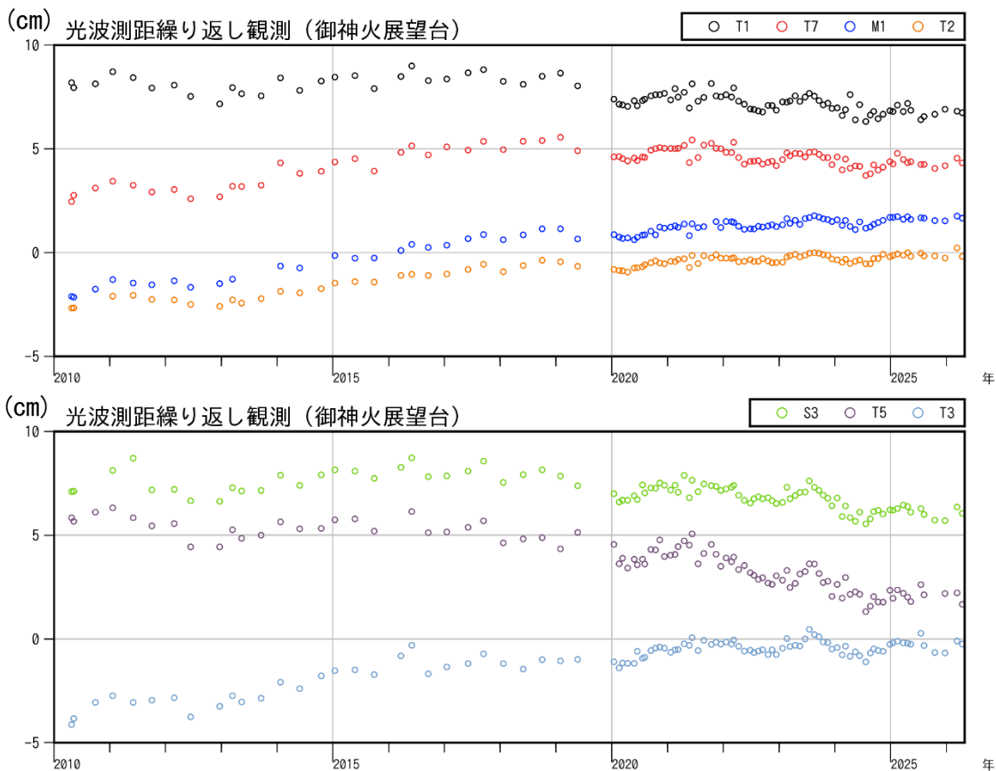
図7 伊豆大島 光波測距繰り返し観測による基線長変化
