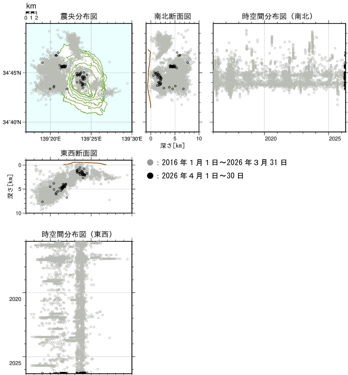
図4 伊豆大島 震源分布図（2016年1月1日～2026年4月30日）
