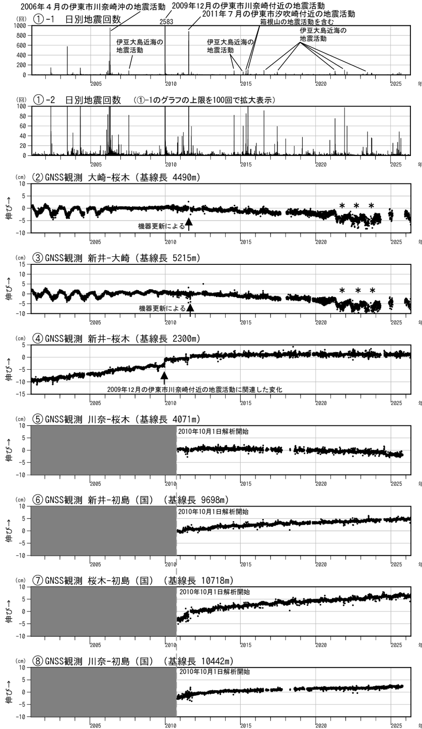
図3 伊豆東部火山群 火山活動経過図 (2001年2月1日~2026年4月30日)
