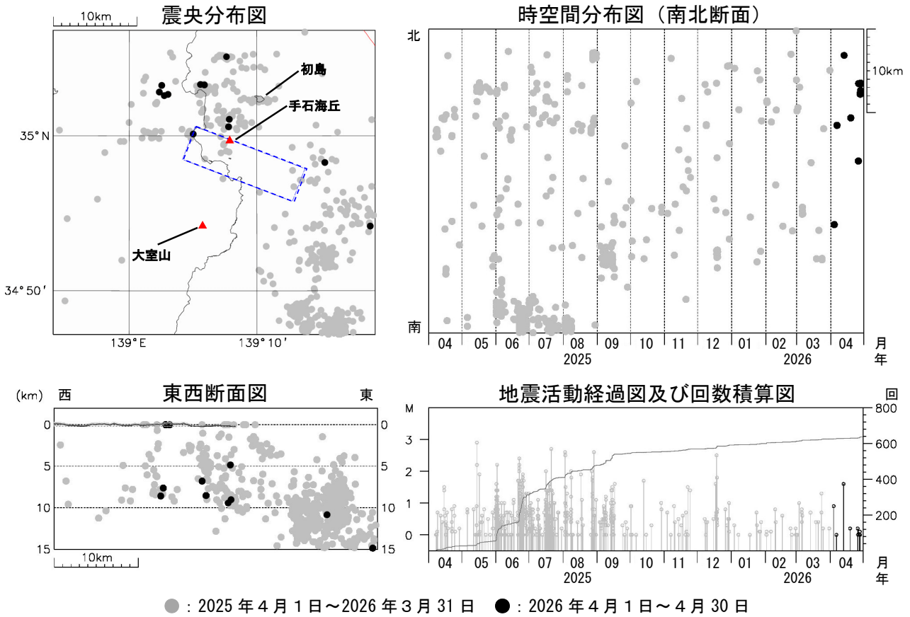
図2 伊豆東部火山群 広域地震観測網による震源分布図（2025年4月1日～2026年4月30日） □の領域は群発地震活動の発生する可能性がある範囲（火口が出現する可能性のある範囲）を示しています。 ( https://www.data.jma.go.jp/vois/data/filing/level/PDF/level_316.pdf ) 広域地震観測網により震源決定したもので、深さは全て海面以下として決定しています。 M（マグニチュード）は地震の規模を表し、M0.0以上を表示しています。 図中の震源要素は一部暫定値が含まれており、後日変更することがあります。 この図では、関係機関の地震波形を一元的に処理し、地震観測点の標高を考慮する等した手法で得られた震源を用いています。
