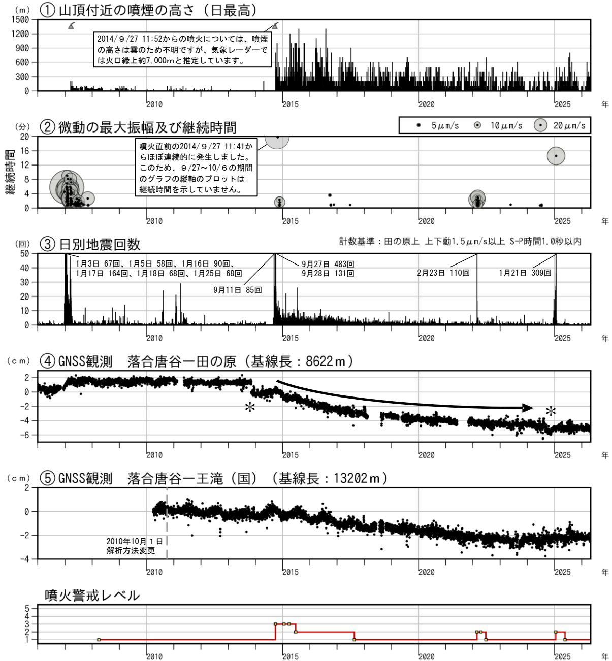
図1 御嶽山 長期間の火山活動経過図（2006年1月1日～2026年4月30日）
