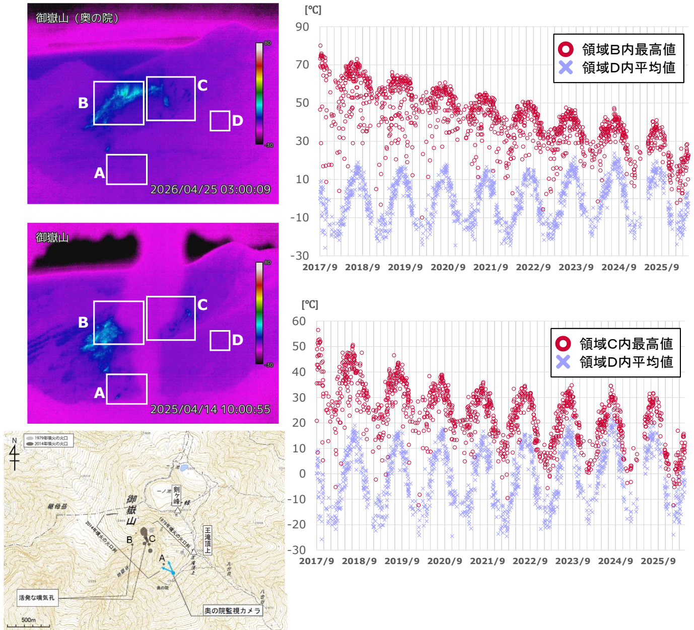
図3 御嶽山 奥の院赤外熱映像カメラによる地獄谷火口における最高温度の推移 (2017年9月13日～2026年4月30日)
