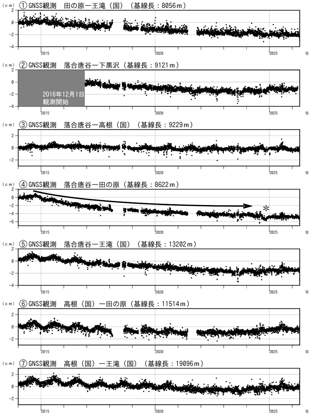
図5 御嶽山 GNSS 連続観測結果（2014年1月1日～2026年4月30日）
