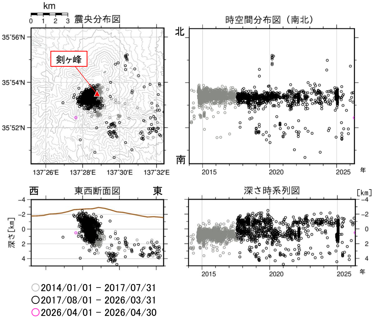
図4 御嶽山 震源分布図（2014年1月1日～2026年4月30日） 2017年8月1日以降の震源分布は、震源計算に使用する観測点を新たに追加して再計算したものを示しています。 観測点の稼動状況により、求まる震源の数の減少や位置の精度低下が生じる場合があります。
