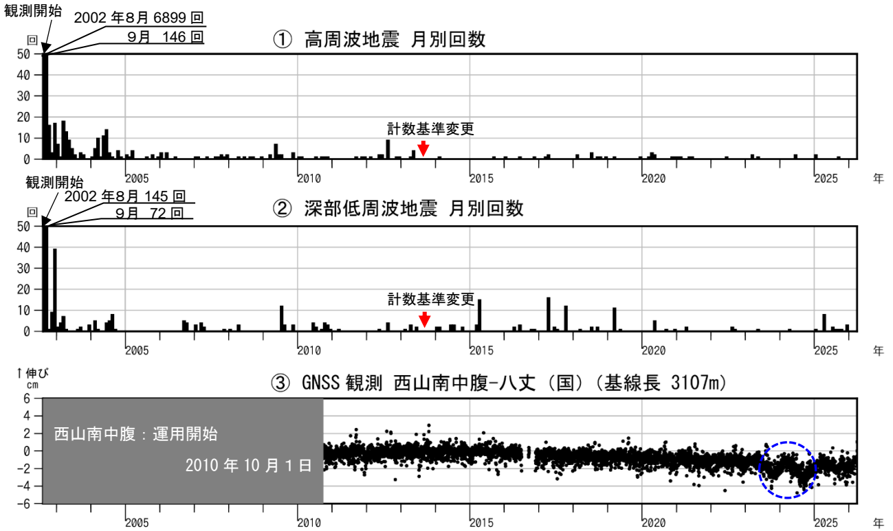
図2 八丈島 火山活動経過図（2002年8月13日～2026年3月31日）
