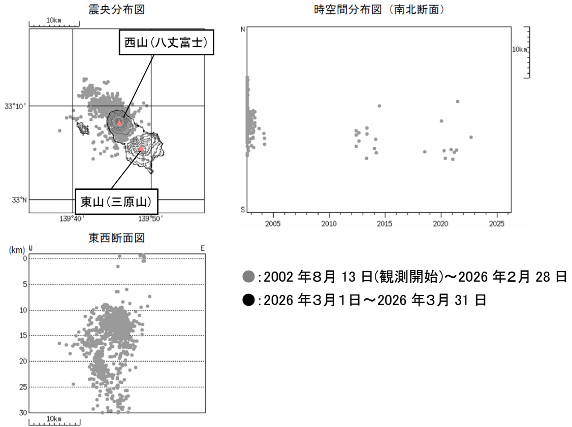
図3 八丈島 震源分布図（2002年8月13日～2026年3月31日）
