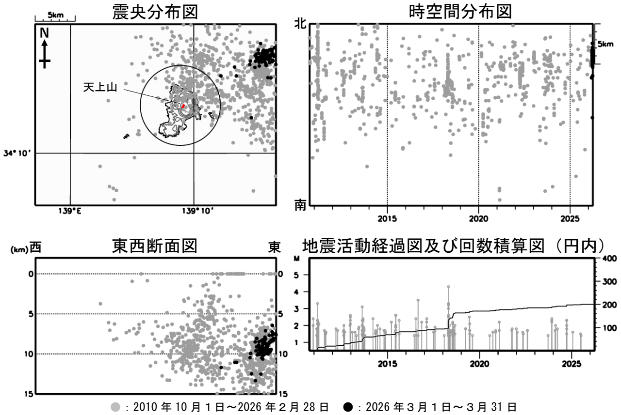
図3 神津島 広域地震観測網による山体・周辺の地震活動（2010年10月1日～2026年3月31日） 広域地震観測網により震源決定したもので、深さは全て海面以下として決定しています。なお、2020年9月以降については、地震観測点の標高を考慮する等、震源決定の手法を変更しています。 M（マグニチュード）は地震の規模を表し、M1.4以上の地震を示しています。 図中の震源要素は一部暫定値が含まれており、後日変更することがあります。 計数対象（天上山西から半径約5km、深さ約15km以内）以外の地震が含まれるため、図2-①の日別地震回数（高周波地震）とは異なります。 震央分布図中の円は火山性地震の回数の計数対象（天上山西から半径5km、深さ15km以内）の範囲を示しています。 ・地震活動は低調に経過しました。
