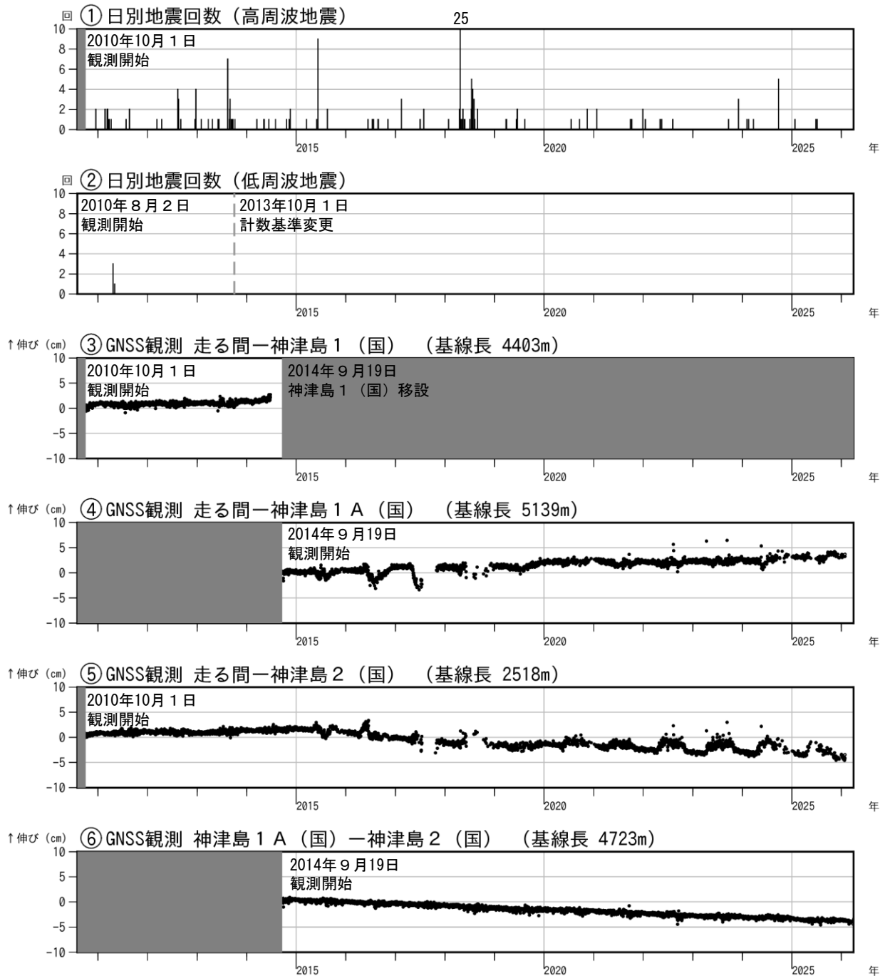
図2 神津島 火山活動経過図(2010年8月2日～2026年3月31日)
