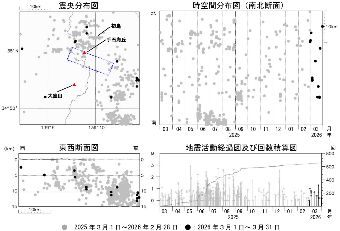
図2 伊豆東部火山群 広域地震観測網による震源分布図（2025年3月1日～2026年3月31日） □の領域は群発地震活動の発生する可能性がある範囲（火口が出現する可能性のある範囲）を示しています。 https://www.data.jma.go.jp/vois/data/filing/level/PDF/level_316.pdf 広域地震観測網により震源決定したもので、深さは全て海面以下として決定しています。 M（マグニチュード）は地震の規模を表し、M0.0以上を表示しています。 図中の震源要素は一部暫定値が含まれており、後日変更することがあります。 この図では、関係機関の地震波形を一元的に処理し、地震観測点の標高を考慮する等した手法で得られた震源を用いています。
