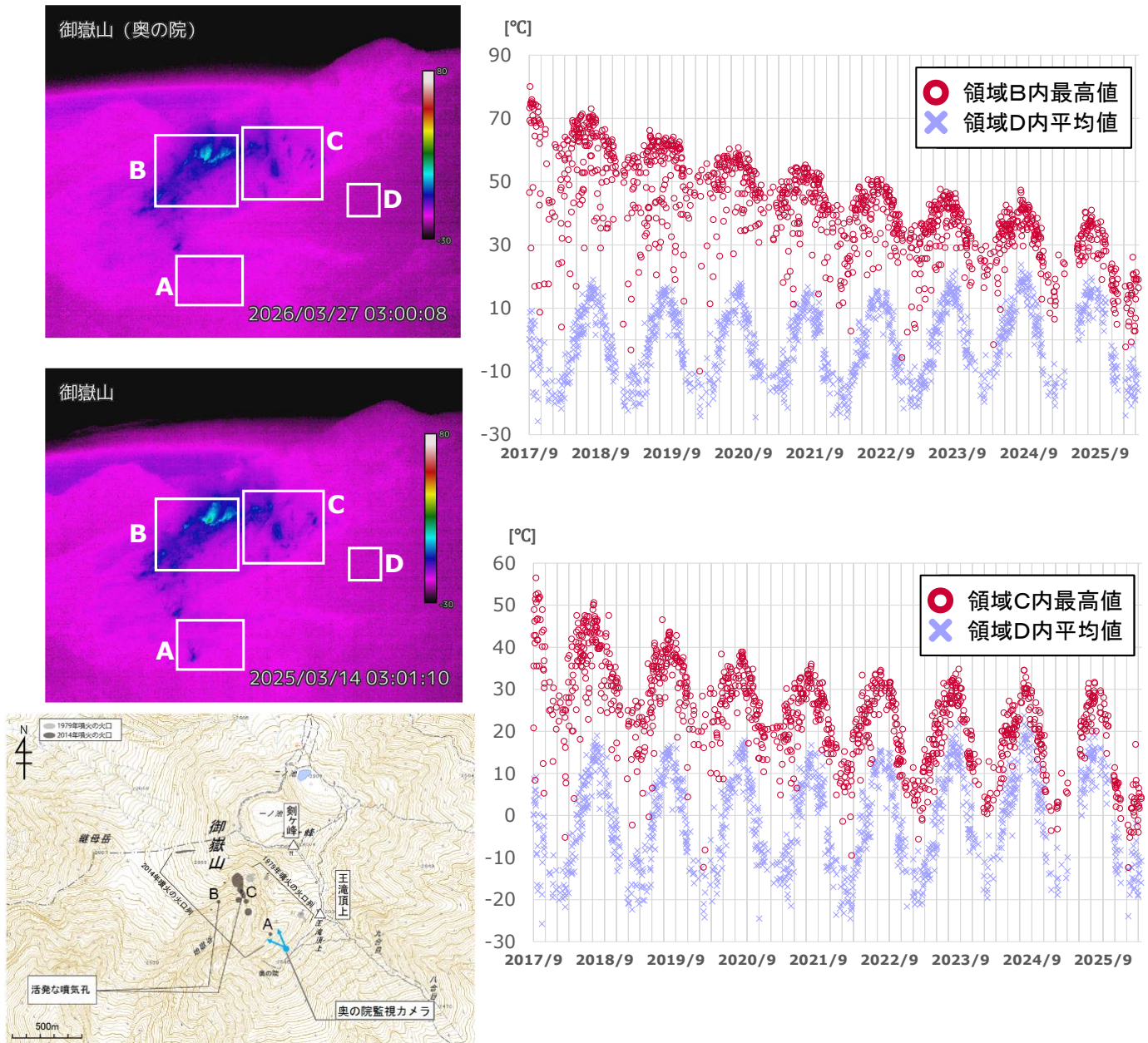
図3 御嶽山 奥の院赤外熱映像カメラによる地獄谷火口における最高温度の推移 (2017年9月13日～2026年3月31日)
