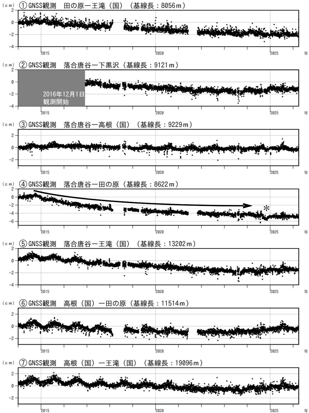
図5 御嶽山 GNSS連続観測結果（2014年1月1日～2026年3月31日）
