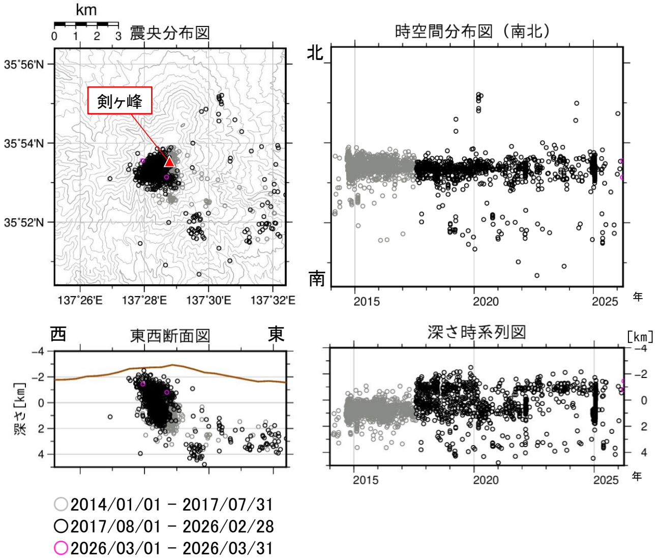
図4 御嶽山 震源分布図（2014年1月1日～2026年3月31日） 2017年8月1日以降の震源分布は、震源計算に使用する観測点を新たに追加して再計算したものを示しています。 観測点の稼働状況により、求まる震源の数の減少や位置の精度低下が生じる場合があります。
