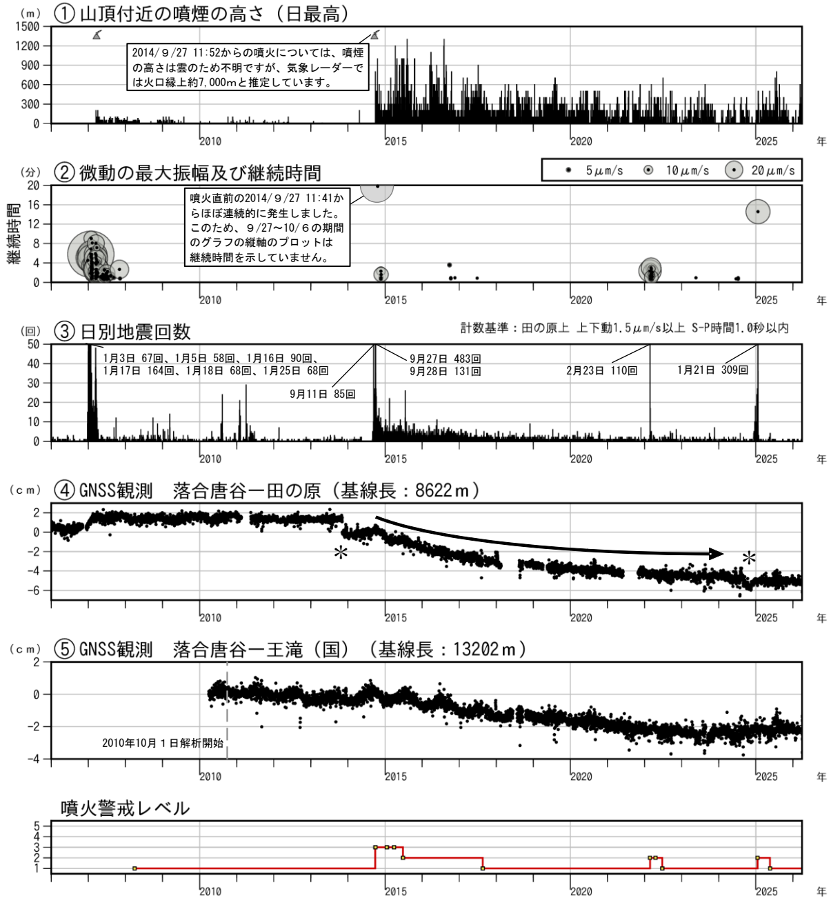
図1 御嶽山 長期間の火山活動経過図（2006年1月1日～2026年3月31日）
