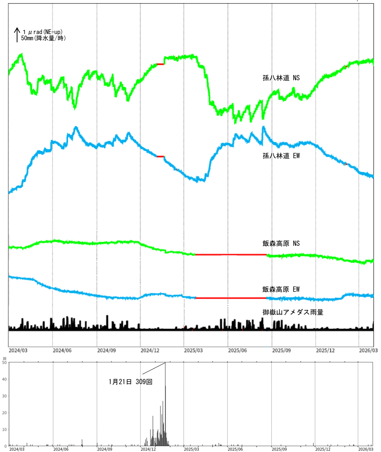
図7 御嶽山 傾斜変動と日別地震回数の推移（2024年3月1日～2026年3月31日）
