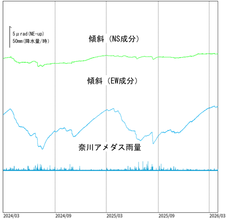
図4 乗鞍岳 三本滝観測点における傾斜データ（2024年3月1日～2026年3月31日） ・傾斜計による観測では、火山活動によるとみられる変動は認められません。
