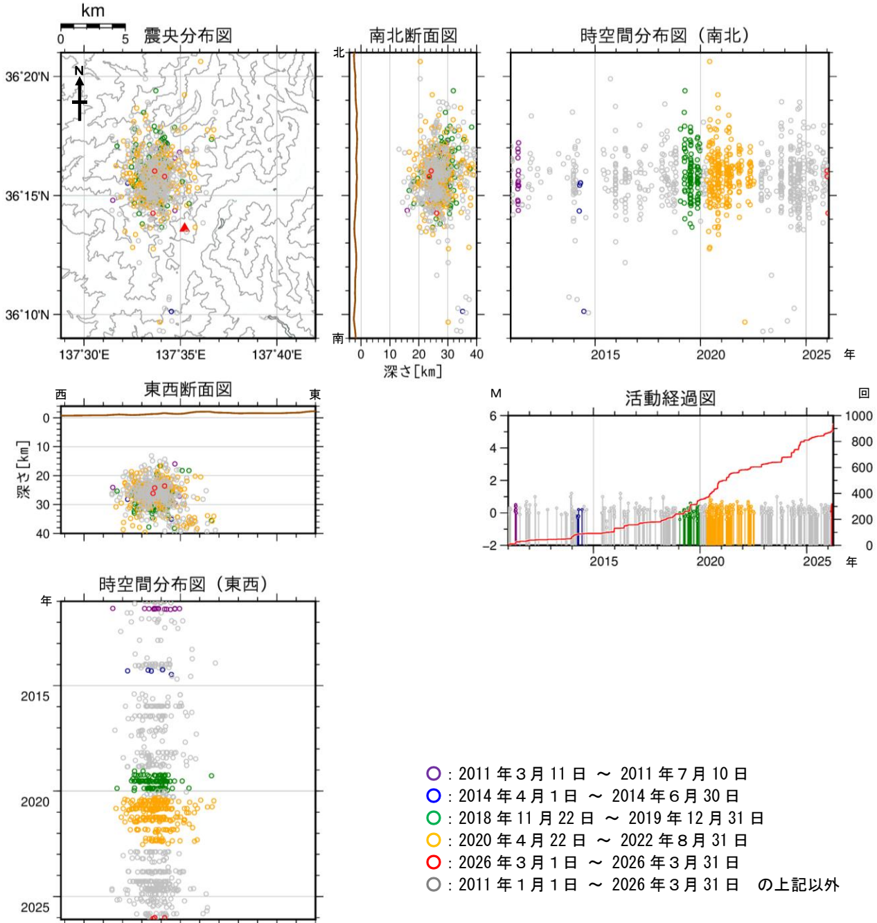
図10 焼岳 広域地震観測網による深部低周波地震の震源分布図（2011年1月1日～2026年3月31日） 広域地震観測網により震源決定したもので、深さは全て海面以下として決定しています。なお、2020年9月以降については、地震観測点の標高を考慮する等、震源決定の手法を変更しています。 M（マグニチュード）は地震の規模を表します。 図中の震源要素は一部暫定値が含まれており、後日変更することがあります。
