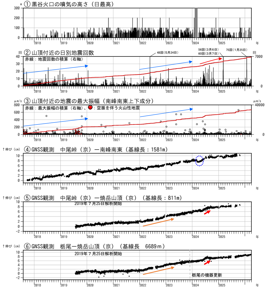
図1 焼岳 火山活動経過図（2017年8月1日～2026年3月31日）
