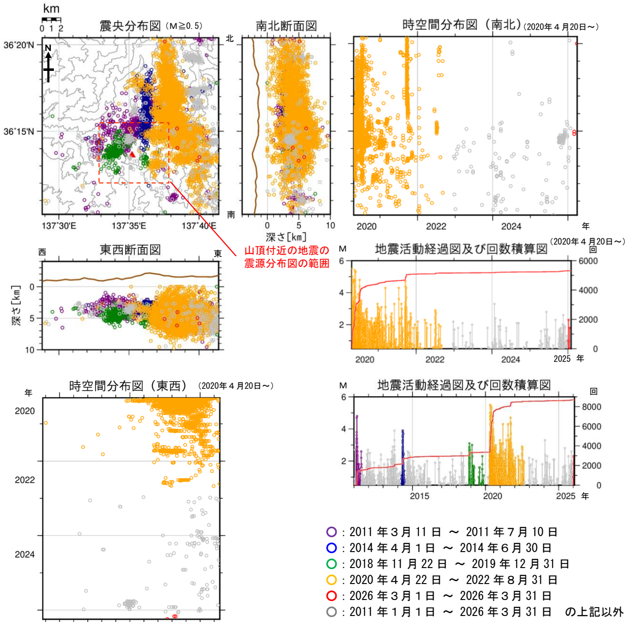
図9 焼岳 広域地震観測網による山体及び周辺の地震活動(2011年1月1日～2026年3月31日)
