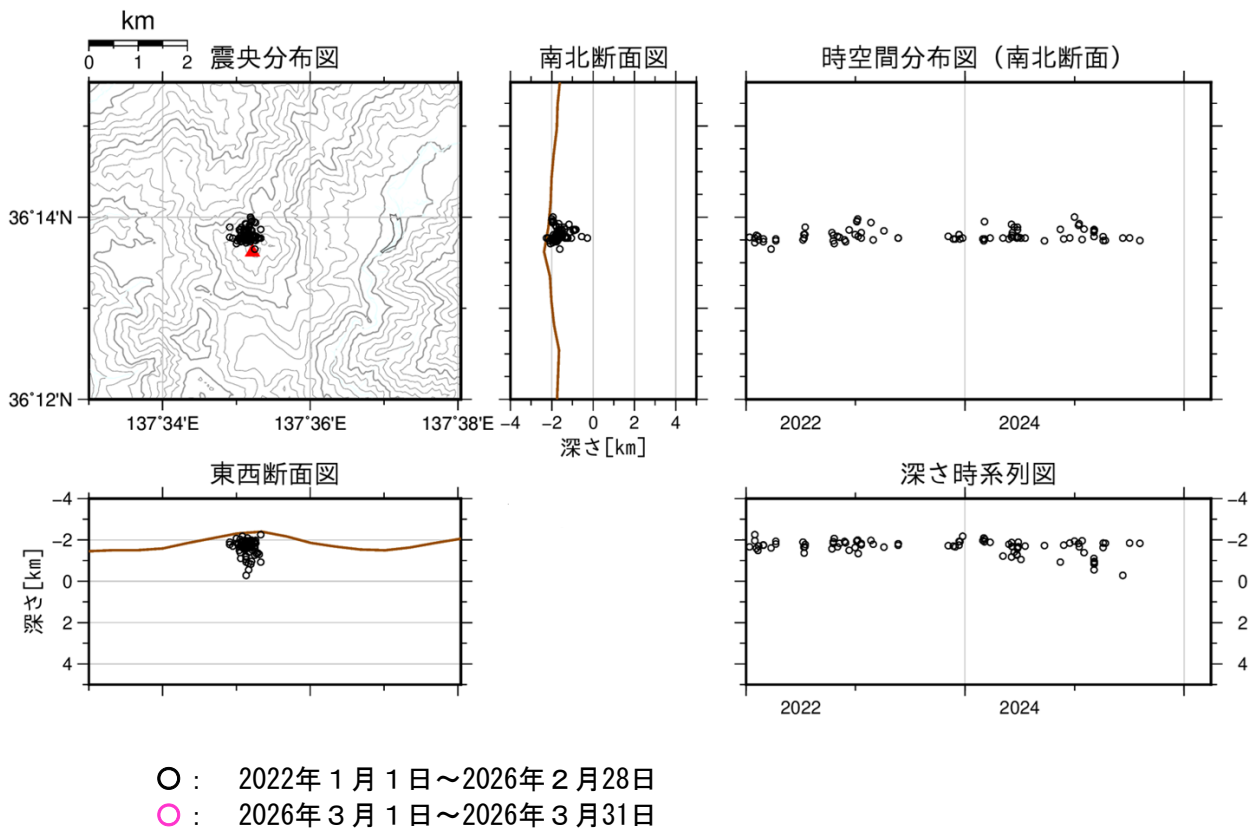
図2 焼岳 山頂付近の地震の震源分布図（2022年1月1日～2026年3月31日）
