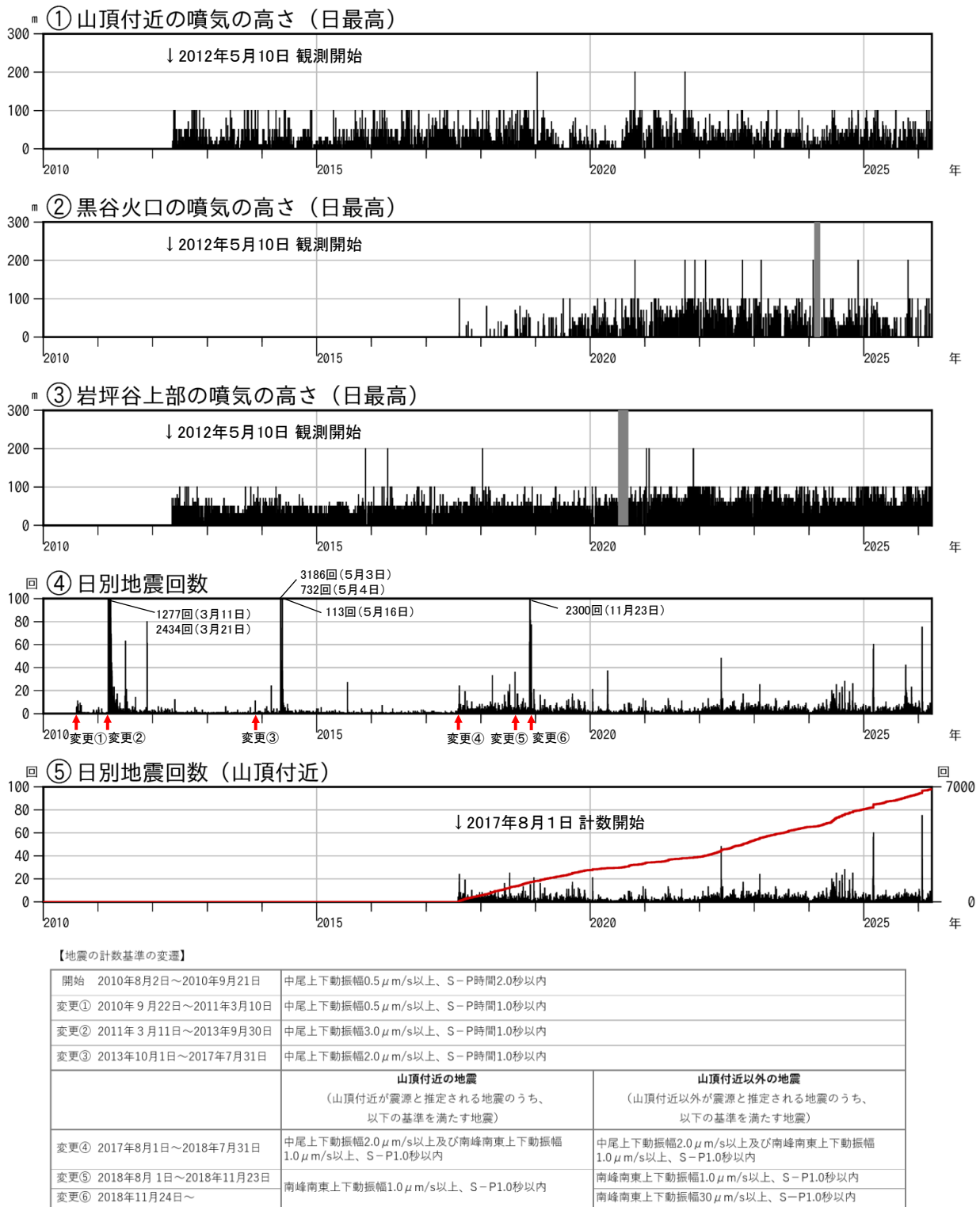
図5 焼岳 噴気の高さと地震回数の推移(2010年8月2日～2026年3月31日)
