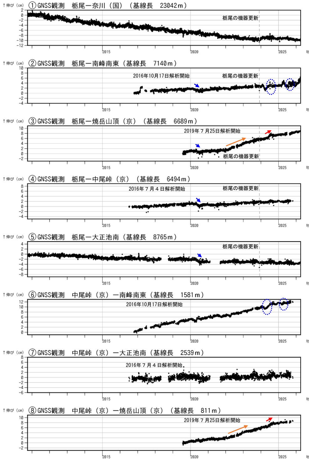
図6 焼岳 GNSS 連続観測による基線長変化 (2010年10月1日~2026年3月31日)
