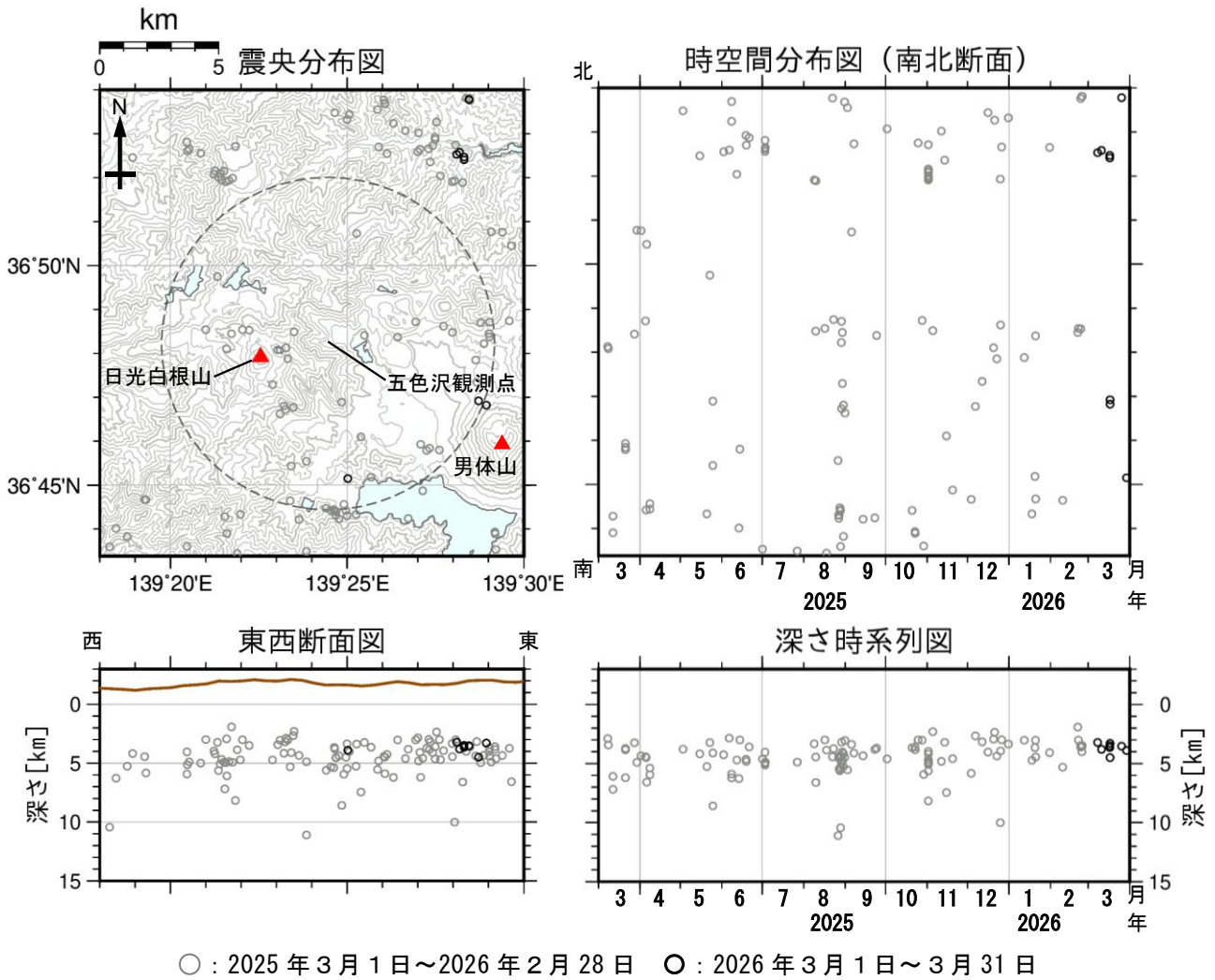
図3 日光白根山 広域地震観測網による山体周辺の地震活動 (2025年3月1日～2026年3月31日)
