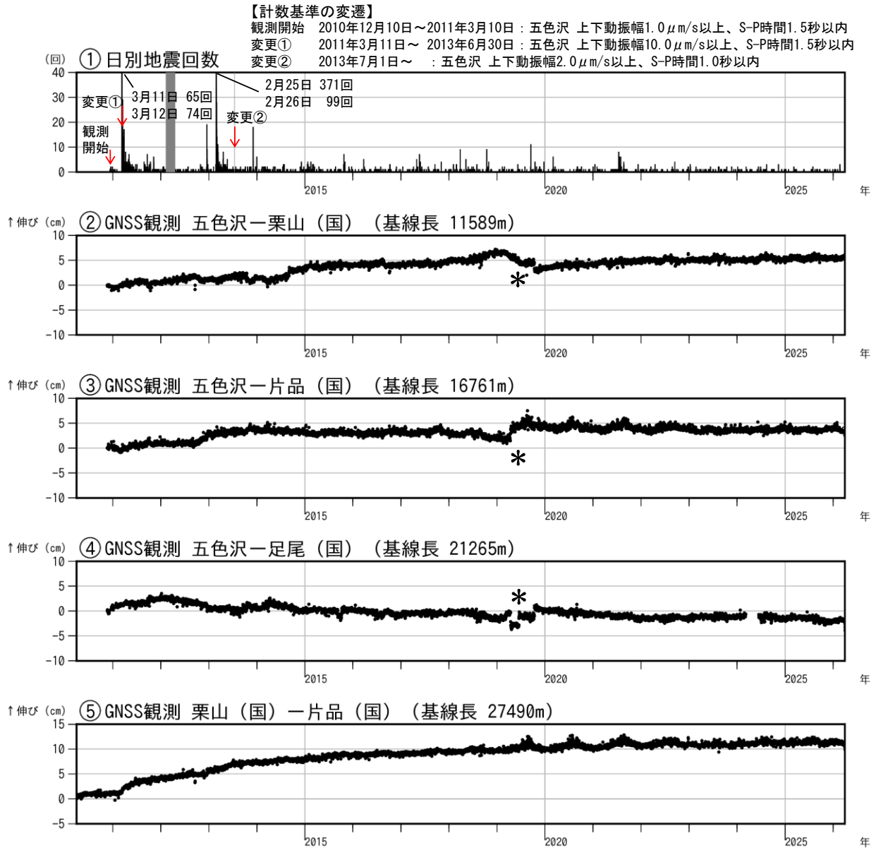
図2 日光白根山 火山活動経過図（2010年4月1日～2026年3月31日）
