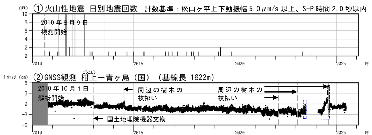
図3 青ヶ島 火山活動経過図（2010年8月9日～2026年1月31日）
