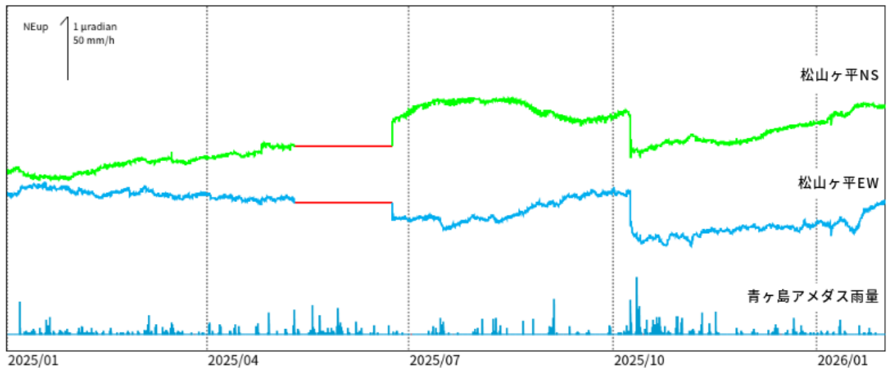
図4 青ヶ島 松山ヶ平観測点における傾斜データ（2025年1月1日～2026年1月31日） グラフの赤線部分は欠測を示す。
