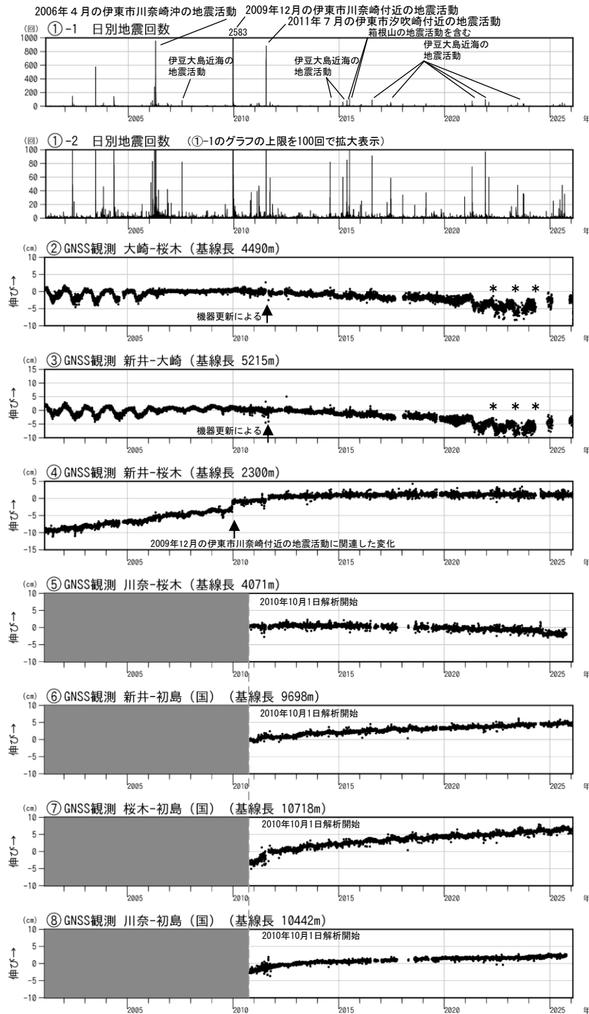
図3 伊豆東部火山群 火山活動経過図（2001年2月1日～2026年1月31日）
