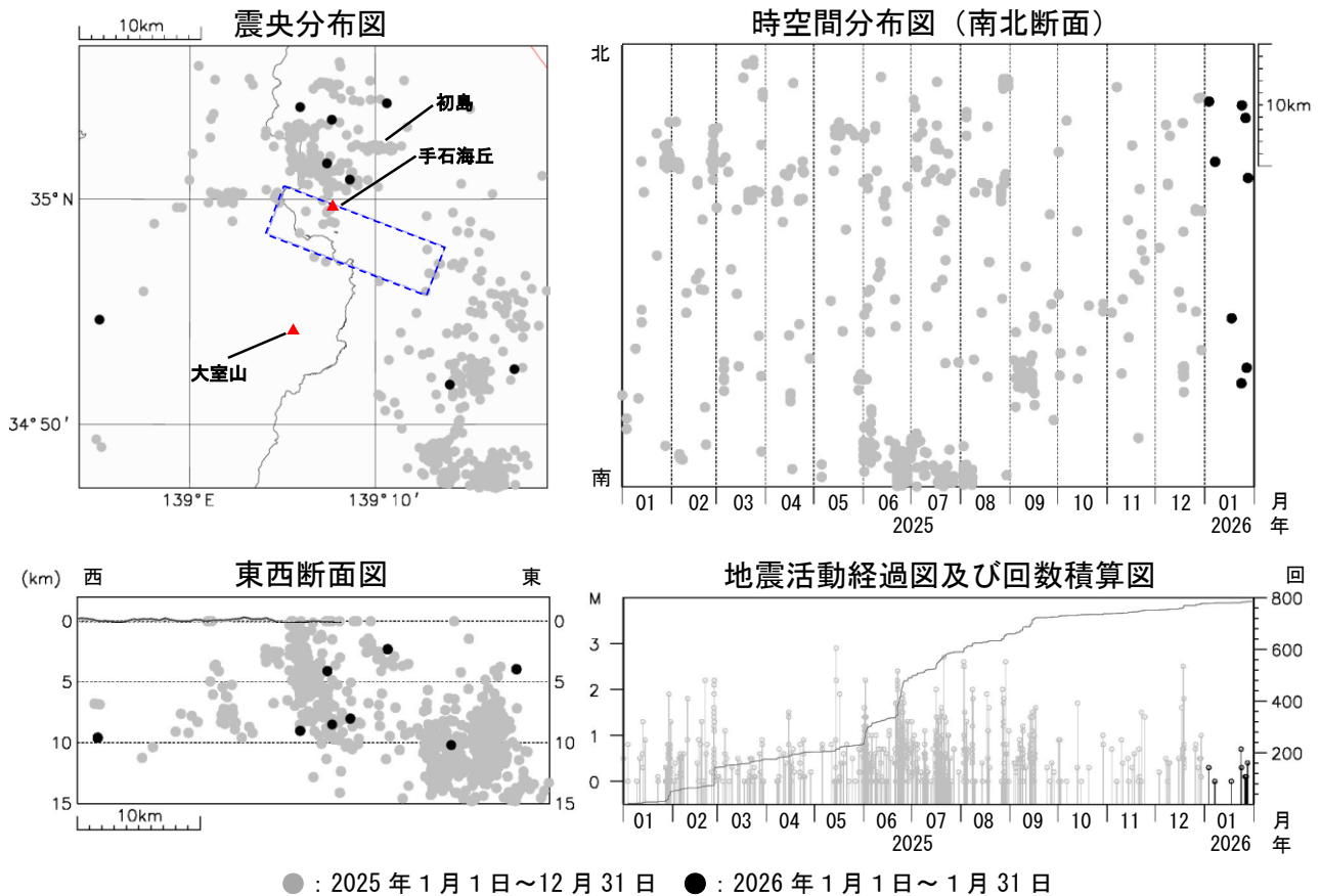
図2 伊豆東部火山群 広域地震観測網による震源分布図（2025 年 1 月 1 日～2026 年 1 月 31 日） □ の領域は群発地震活動の発生する可能性がある範囲（火口が出現する可能性のある範囲）を示しています。 https://www.data.jma.go.jp/vois/data/filing/level/PDF/level_316.pdf 広域地震観測網により震源決定したもので、深さは全て海面以下として決定しています。 M（マグニチュード）は地震の規模を表し、M0.0 以上を表示しています。 図中の震源要素は一部暫定値が含まれており、後日変更することがあります。 この図では、関係機関の地震波形を一元的に処理し、地震観測点の標高を考慮する等した手法で得られた震源を用いています。
