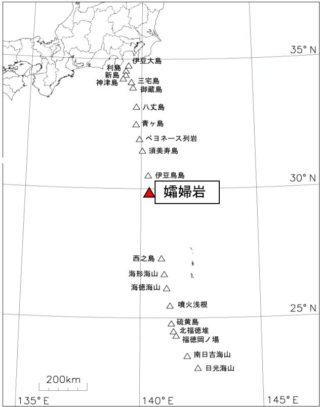
図2 伊豆・小笠原諸島の活火山分布及び孀婦岩の位置図
