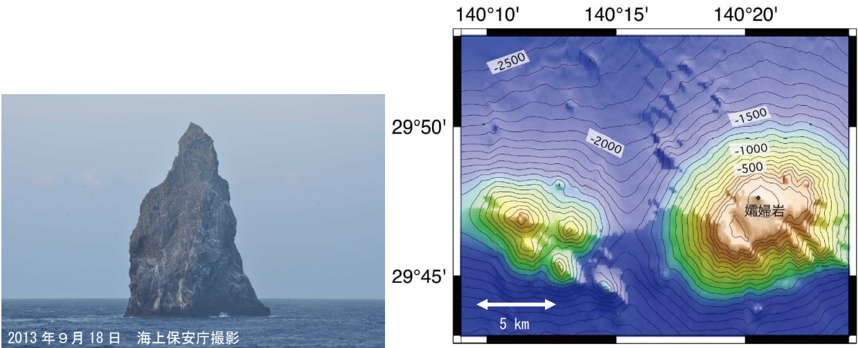
図3 孀婦岩（左図）及び付近の海底地形図（右図）
