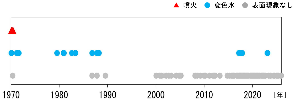
図4 ベヨネース列岩 1970年以降の活動状況
