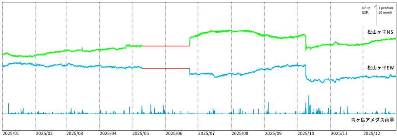
図4 青ヶ島 松山ヶ平観測点における傾斜データ（2025年1月1日～2025年12月31日） グラフの赤線部分は欠測を示す。 ・傾斜計による観測では、火山活動によるとみられる変動は認められません。
