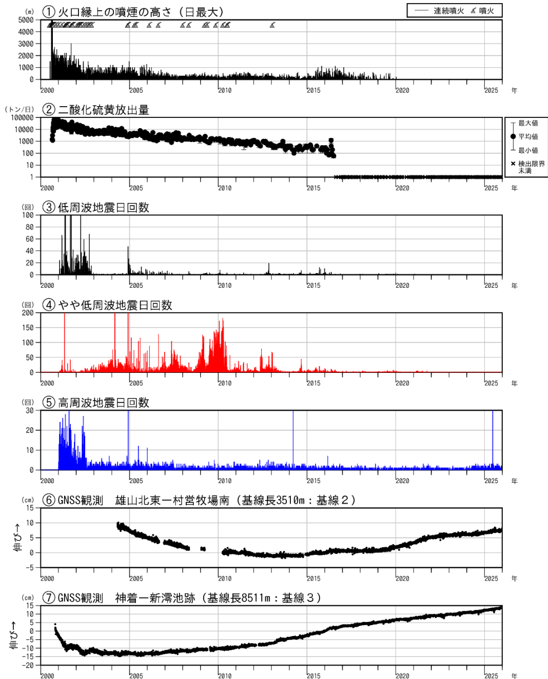
図6 三宅島 長期の火山活動経過図（2000年1月1日～2025年12月31日）
