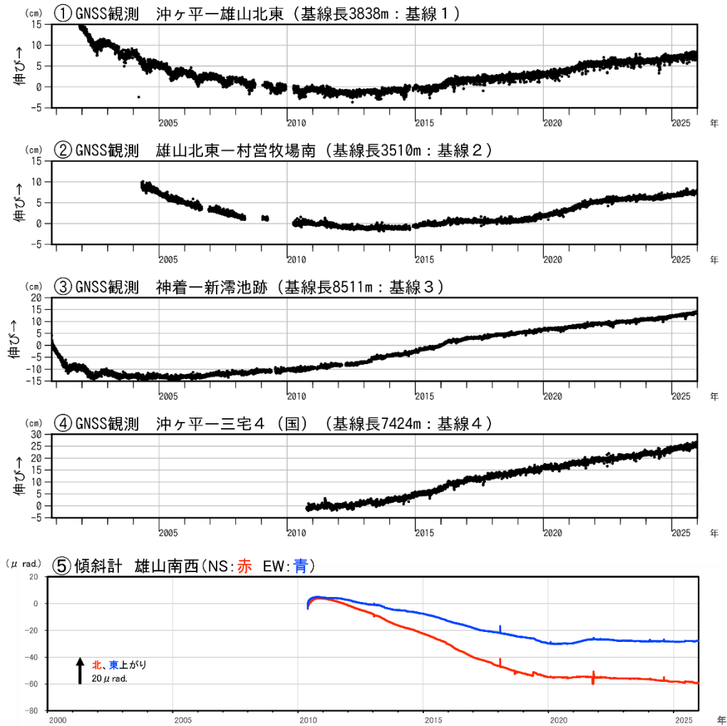
図7 三宅島 GNSS 連続観測及び傾斜計観測結果（2000 年 10 月 26 日～2025 年 12 月 31 日）
