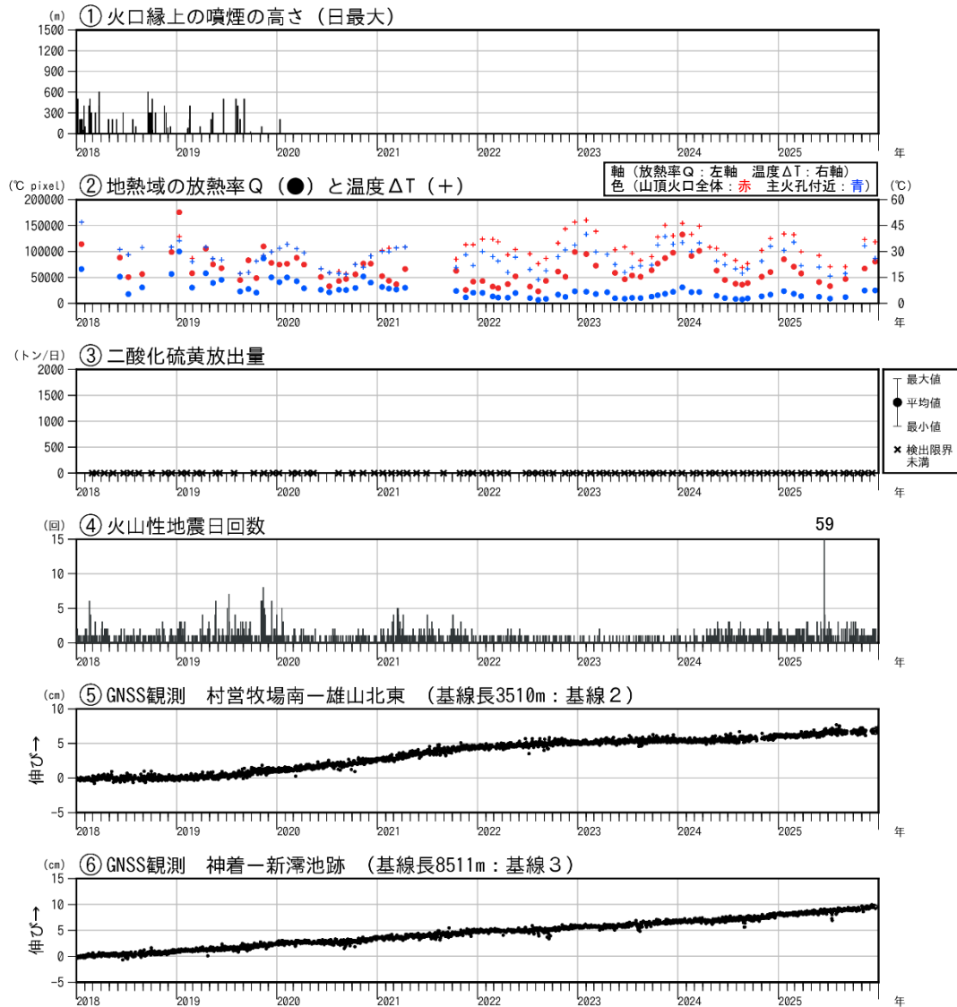
図5 三宅島 火山活動経過図（2018年1月1日～2025年12月31日）
