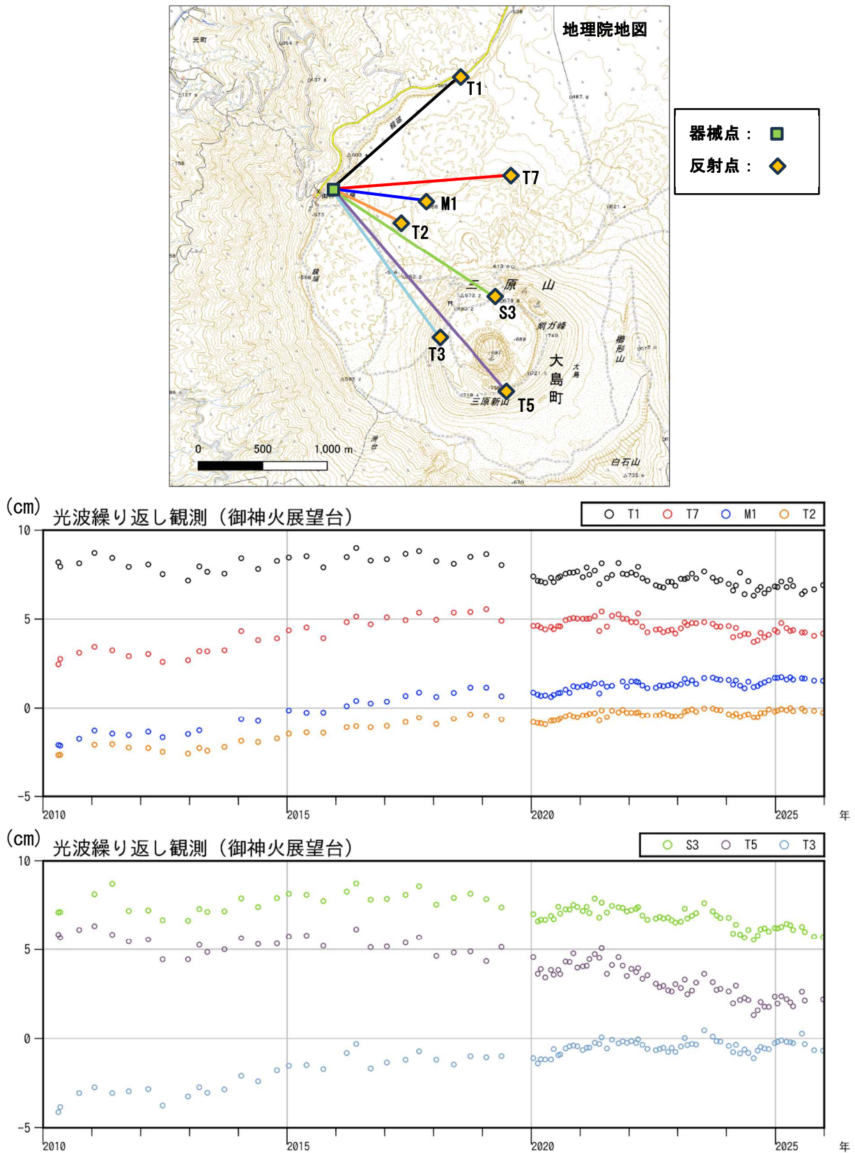
図7 伊豆大島 光波測距繰り返し観測による基線長変化
