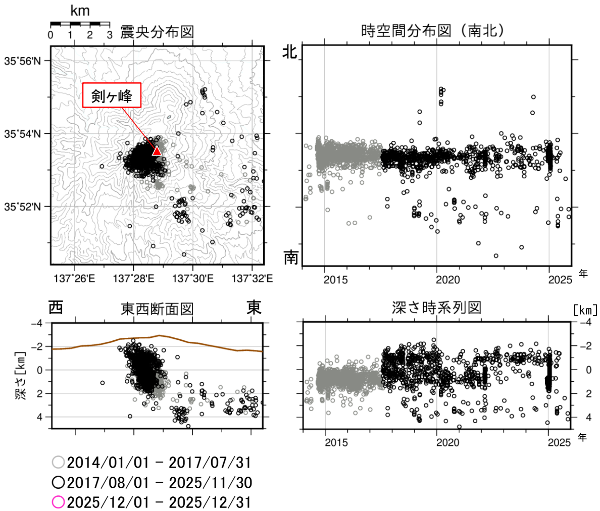
図 4 御嶽山 震源分布図（2014 年 1 月 1 日～2025 年 12 月 31 日）
