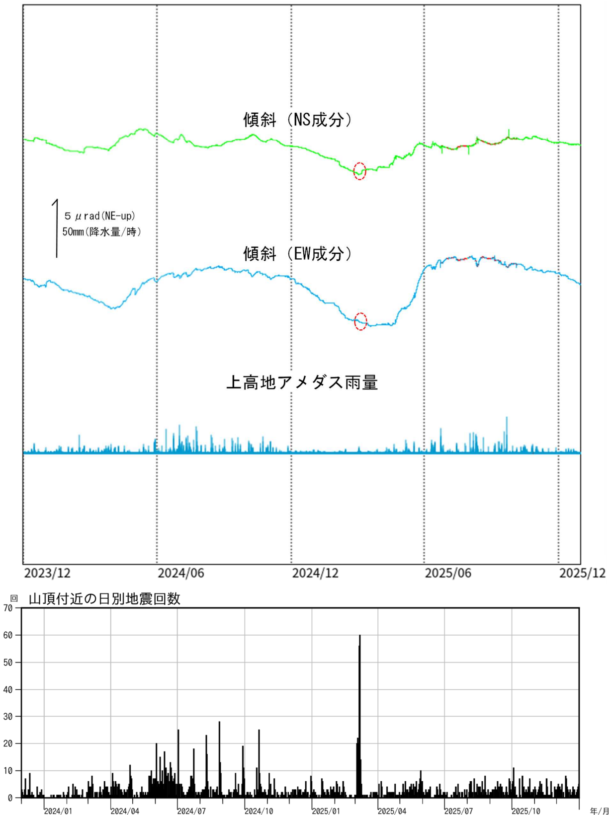
図8 焼岳 南峰南東観測点における傾斜データ（2023年12月1日～2025年12月31日） 赤線部分は欠測を示します。
