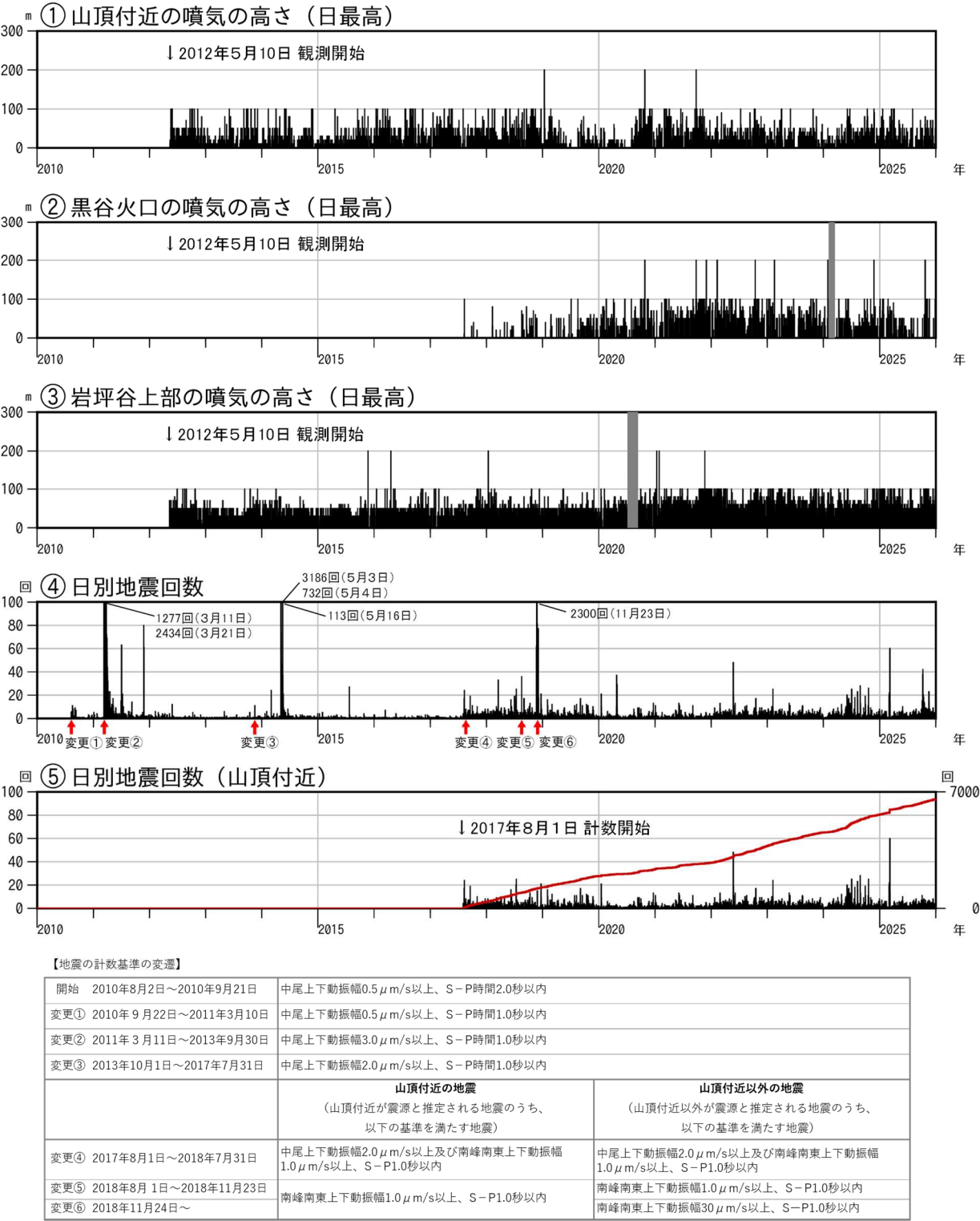
図5 焼岳 噴気の高さと地震回数の推移(2010年8月2日～2025年12月31日) ②黒谷火口の噴気の高さは、2024年2月5日から3月14日にかけて、障害のため欠測（灰色の期間）。 ③岩坪谷上部の噴気の高さは、2020年7月7日から9月10日にかけて、障害のため欠測（灰色の期間）。 ④2017年8月1日以降、山頂付近の地震と山頂付近以外の地震を分けて計数していますが、④ではこれらを合計した回数を示しています。図中の赤矢印は計数基準の変更を示しています。 ⑤山頂付近の日別地震回数（左軸）と日別地震回数の積算（右軸）を示しています。 ・黒谷火口では、2017年夏頃から噴気が時々観測されるようになり、2019年夏頃から噴気を観測する日が増えました。
