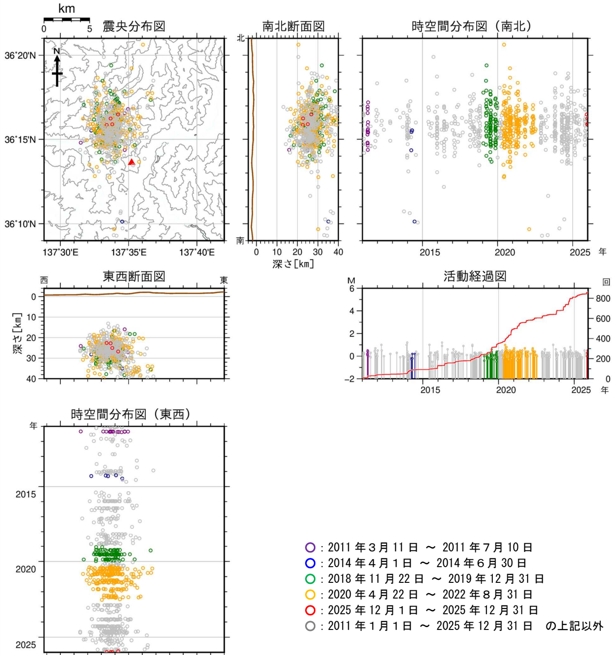
図10 焼岳 広域地震観測網による深部低周波地震の震源分布図（2011年1月1日～2025年12月31日）
