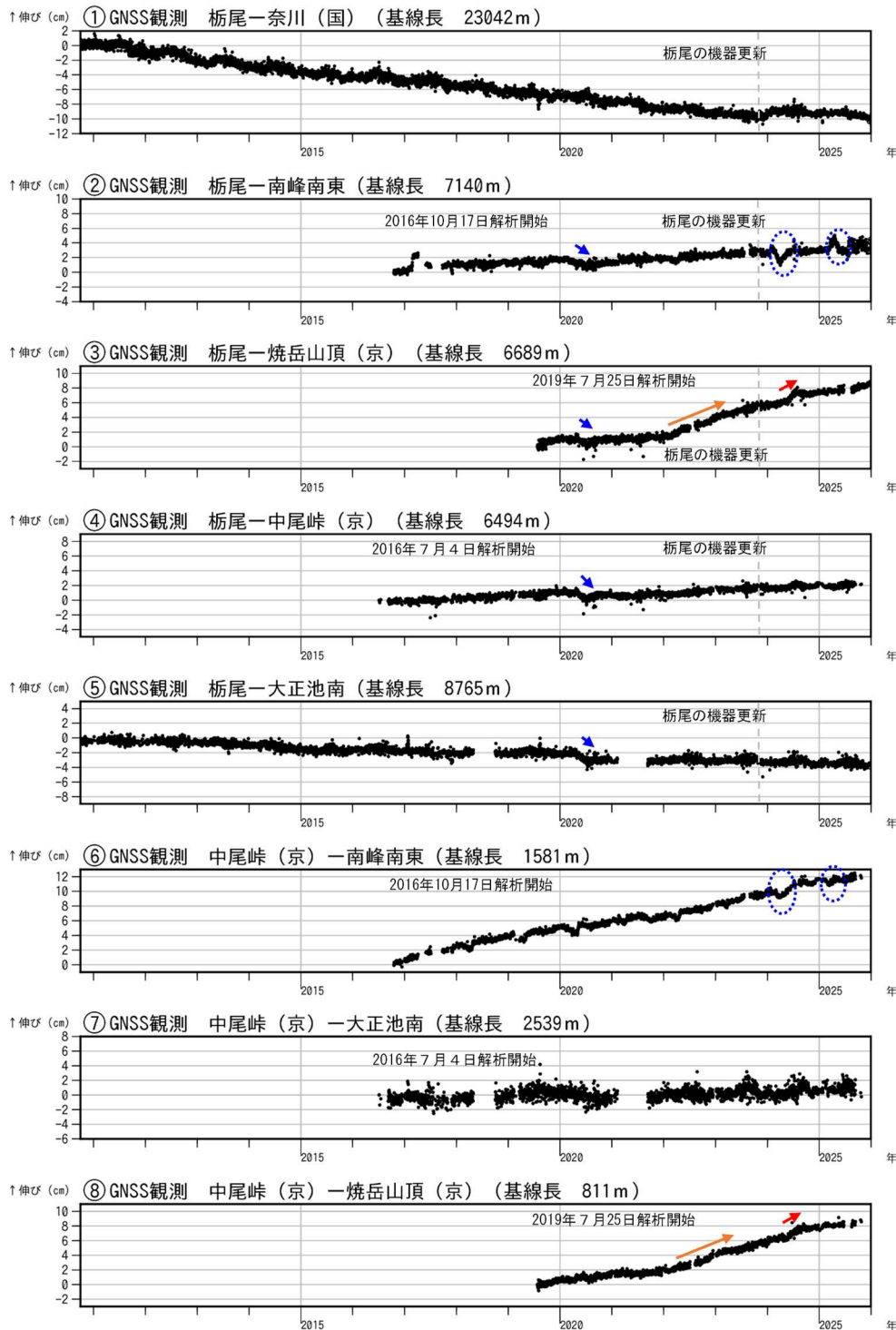
図6 焼岳 GNSS 連続観測による基線長変化（2010年10月1日～2025年12月31日）
