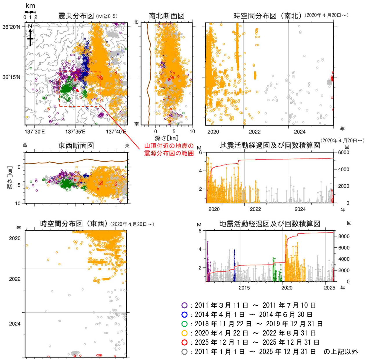
図9 焼岳 広域地震観測網による山体及び周辺の地震活動(2011年1月1日～2025年12月31日)
