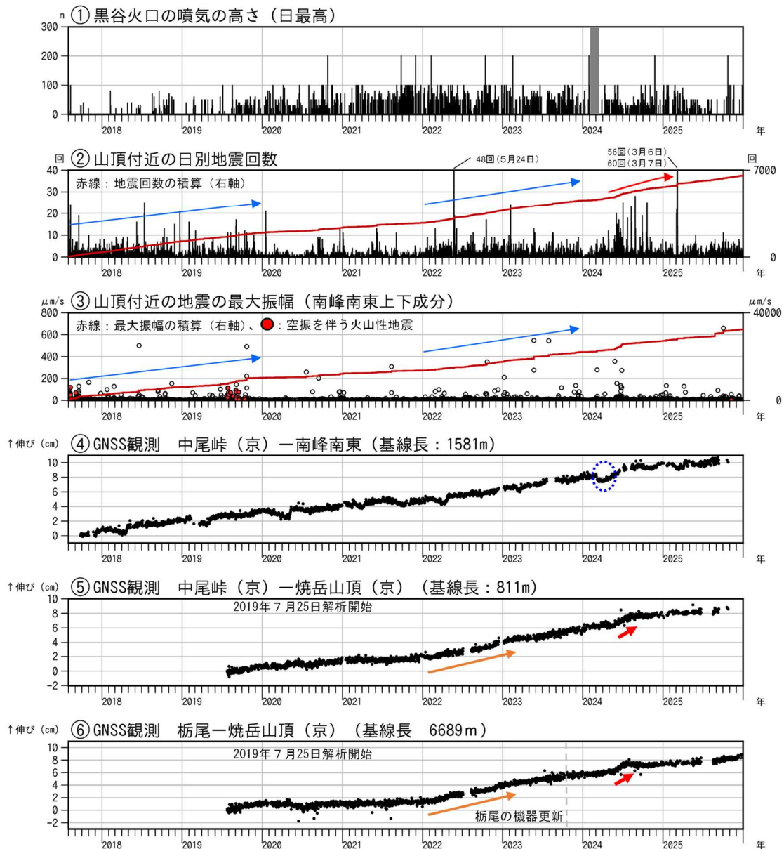
図1 焼岳 火山活動経過図（2017年8月1日～2025年12月31日）
