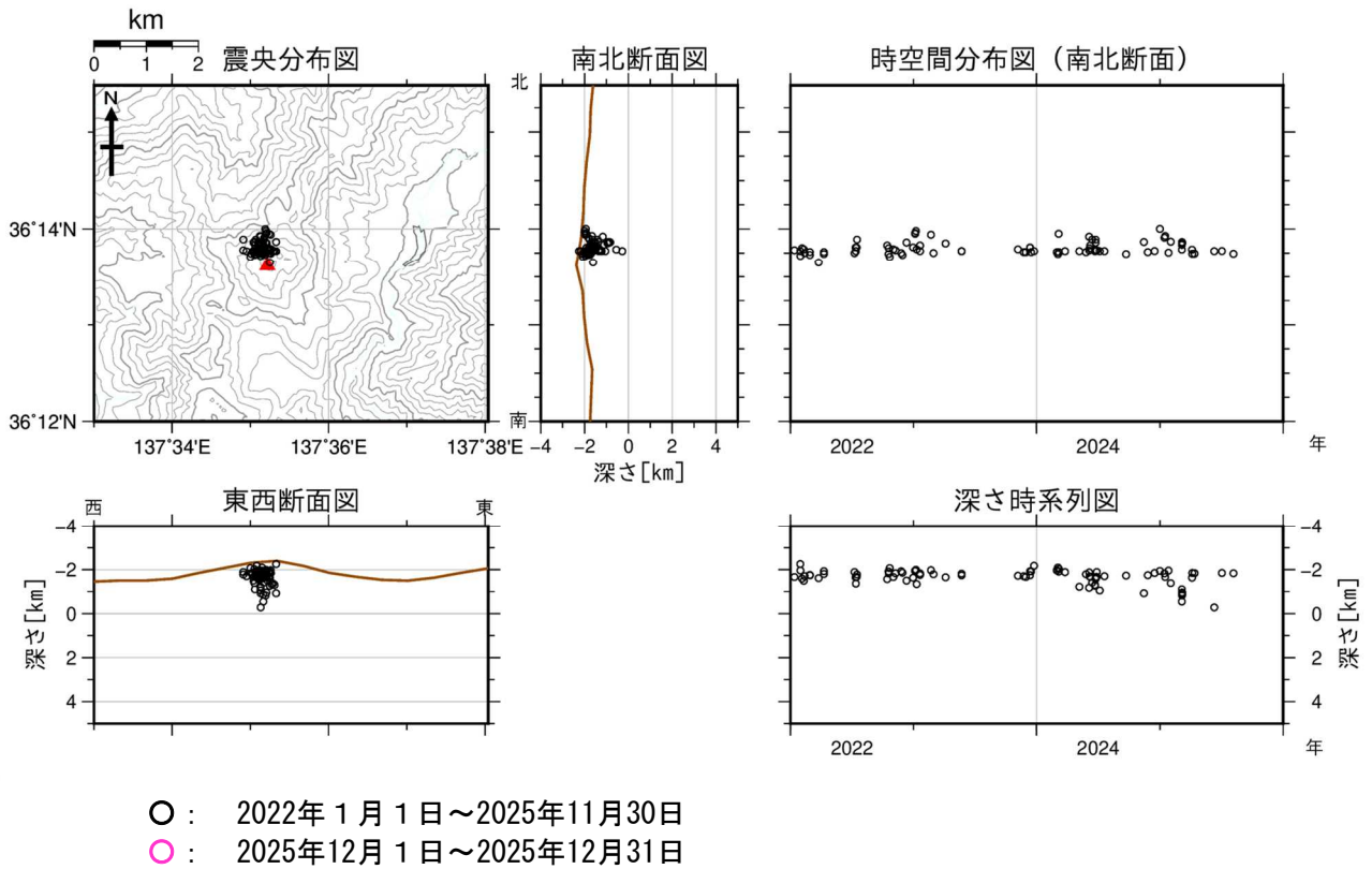
図2 焼岳 山頂付近の地震の震源分布図（2022年1月1日～2025年12月31日）
