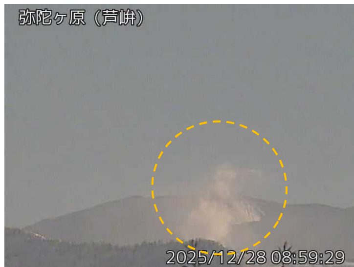
図1 弥陀ヶ原 地獄谷からの噴気の状況（橙丸）（12月28日、芦峠監視カメラによる）
