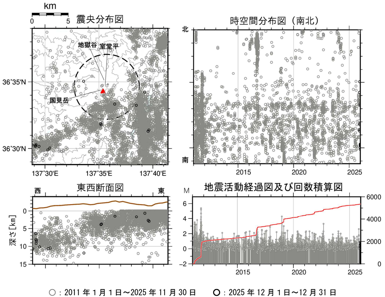
図2 弥陀ヶ原 広域地震観測網による山体・周辺の地震活動（2011年1月1日～2025年12月31日） 震央分布図中の円は弥陀ヶ原の計数対象地震（室堂平でS-P時間1秒以内）のおよその範囲を示しています。 広域地震観測網により震源決定したもので、深さは全て海面以下として決定しています。なお、2020年9月以降については、地震観測点の標高を考慮する等、震源決定の手法を変更しています。 図中の震源要素は一部暫定値が含まれており、後日変更することがあります。
