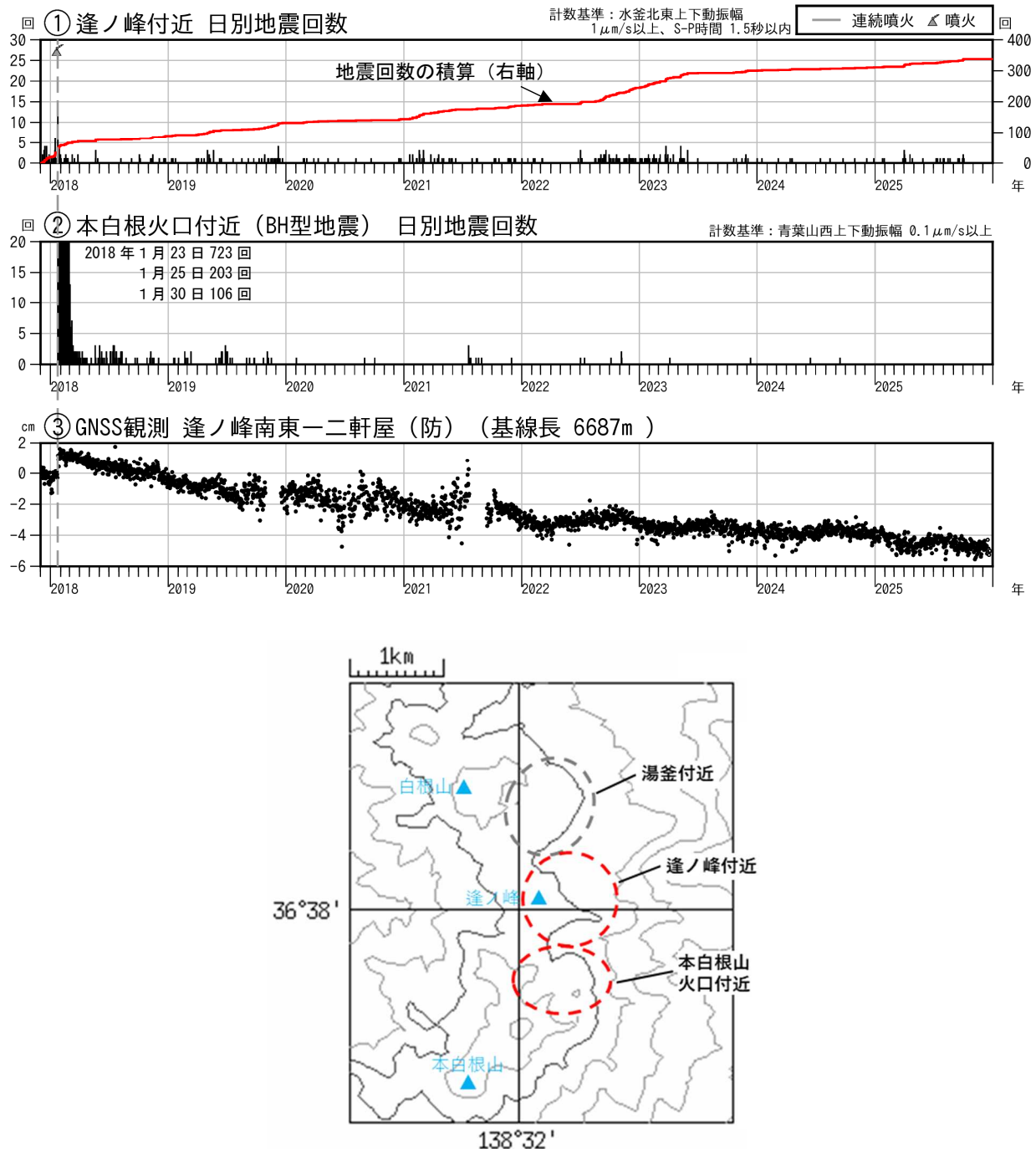
図15 草津白根山（本白根山） 火山活動経過図（2017年12月1日～2025年12月31日）
