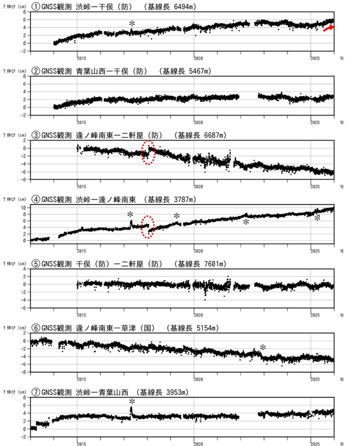
図 7-1 草津白根山 GNSS 連続観測結果 (2013 年 1 月 1 日～2025 年 12 月 31 日)
