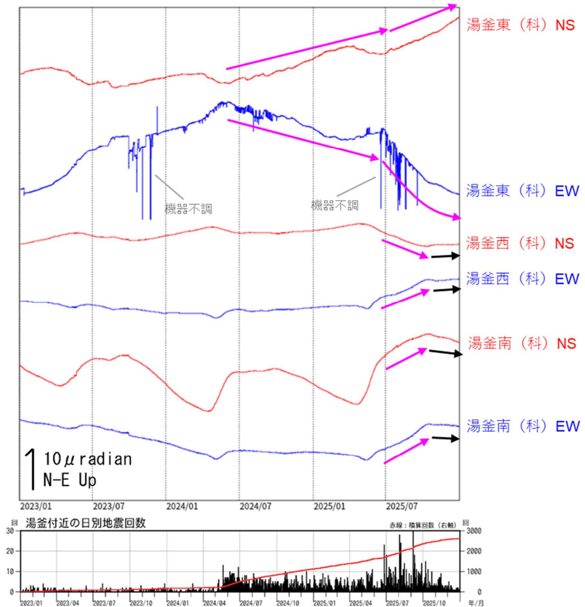
図6 草津白根山（白根山（湯釜付近）） 傾斜変動（2023年1月～2025年12月31日） データは時間平均値を使用しています。（科）：東京科学大学
