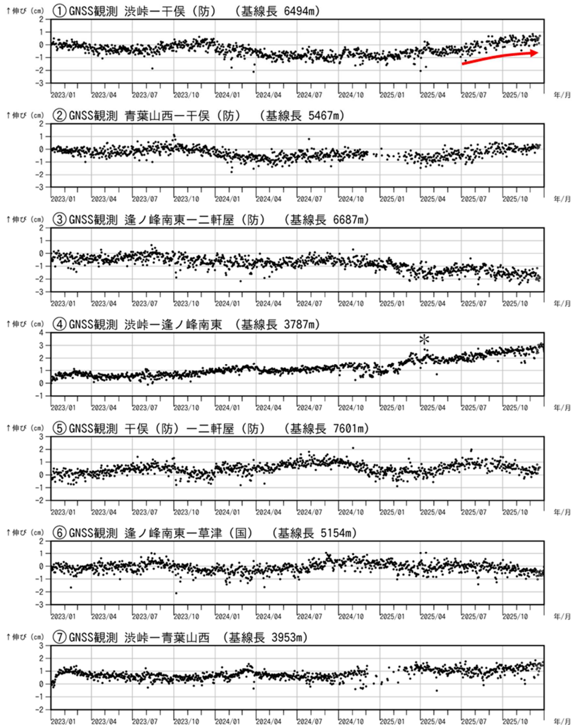
図7-2 草津白根山 GNSS 連続観測結果 (2023 年 1 月 1 日～2025 年 12 月 31 日)
