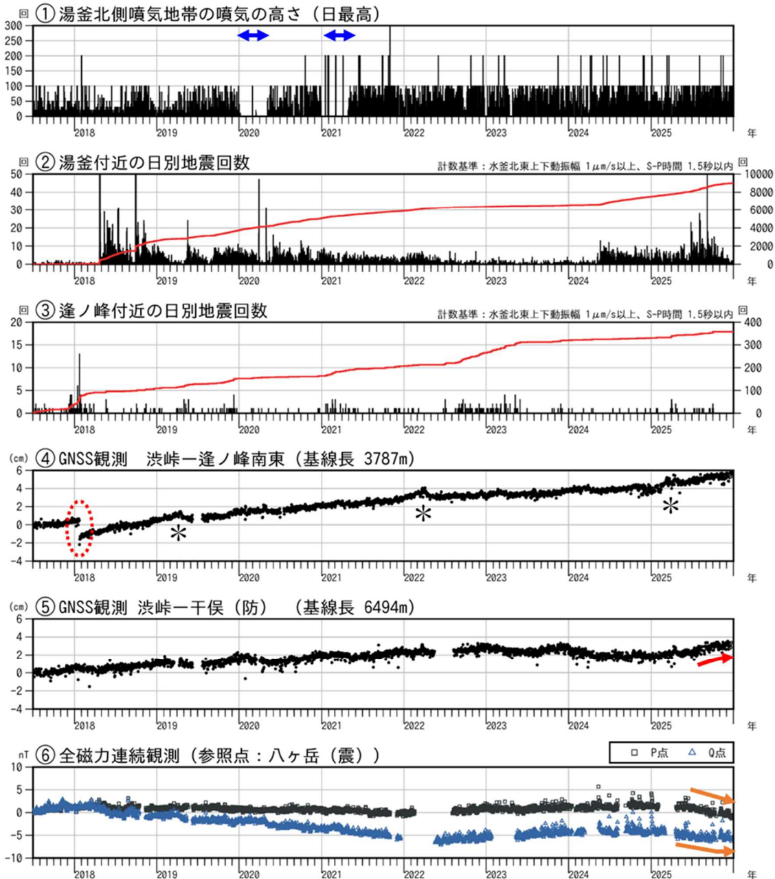
図9 草津白根山（白根山（湯釜付近）） 火山活動経過図（2017年7月1日～2025年12月31日）
