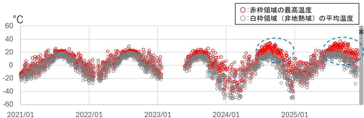
図 1－4 草津白根山（白根山（湯釜付近）） 水釜北東の地熱域の状況 (2021 年 1 月 1 日～2025 年 12 月 31 日)
