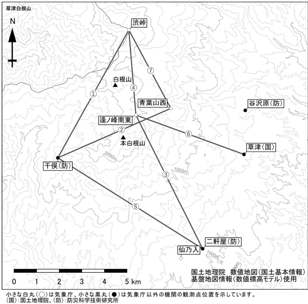
図8 草津白根山 GNSS 観測点配置図 図中の GNSS 基線は図7、図9 及び図 15 に対応しています。
