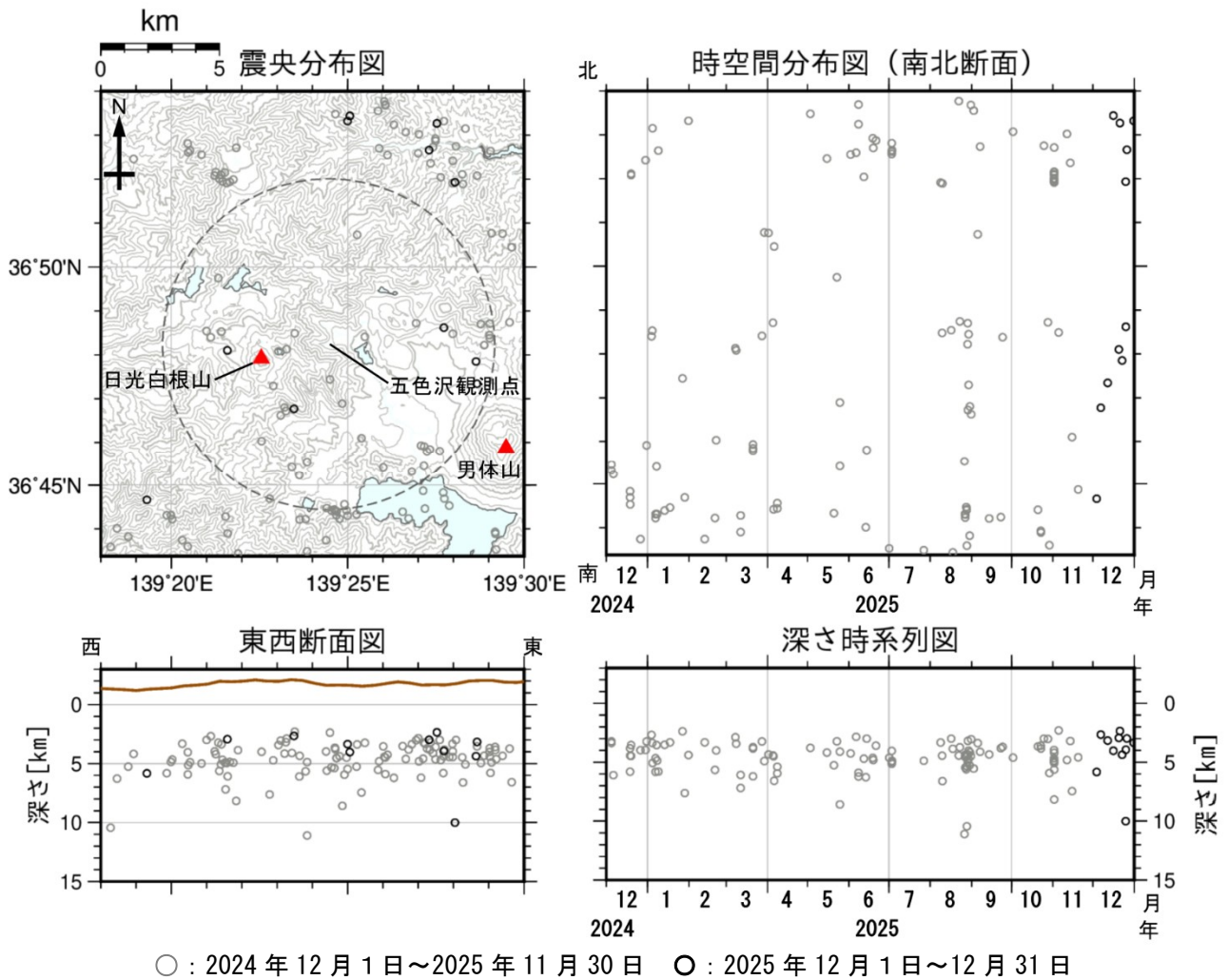
図3 日光白根山 広域地震観測網による山体周辺の地震活動 (2024 年 12 月 1 日～2025 年 12 月 31 日)
