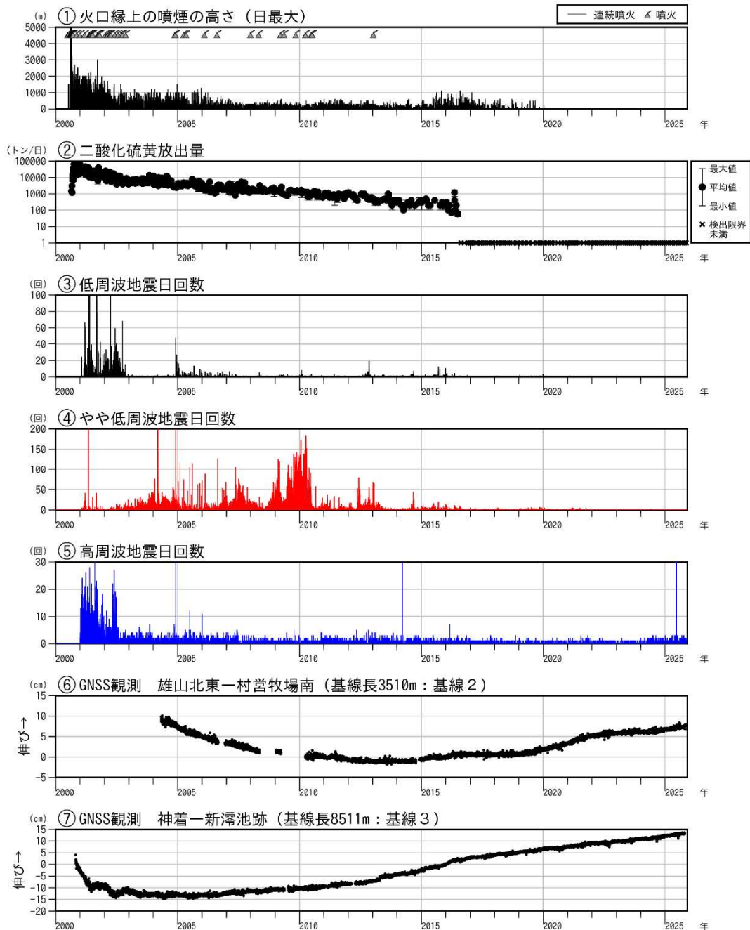
図6 三宅島 長期の火山活動経過図（2000年1月1日～2025年11月30日）
