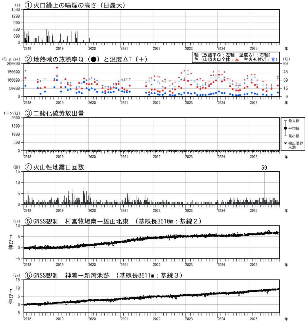
図5 三宅島 火山活動経過図（2018年1月1日～2025年11月30日）
