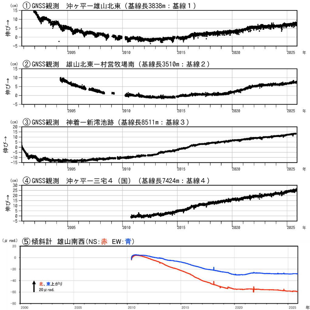
図7 三宅島 GNSS 連続観測及び傾斜計観測結果（2000年10月26日～2025年11月30日）
